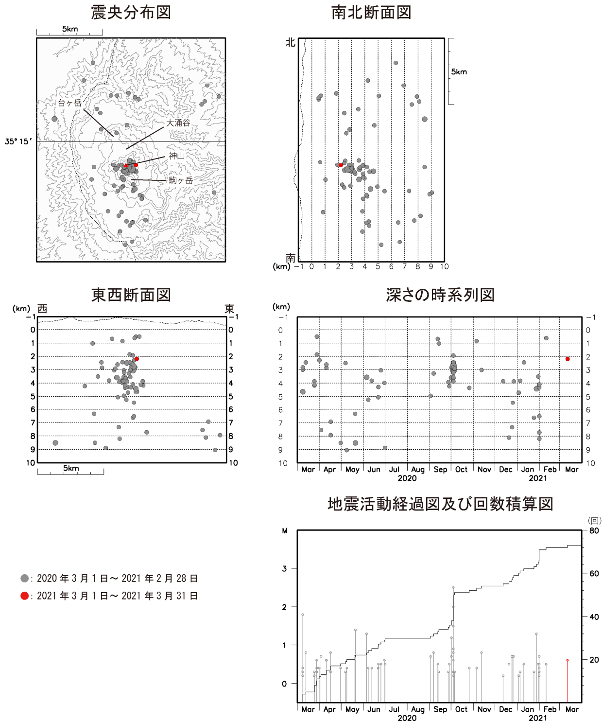
図8 箱根山 広域地震観測網による山体周辺の震源分布図（2020年3月1日～2021年3月31日）
