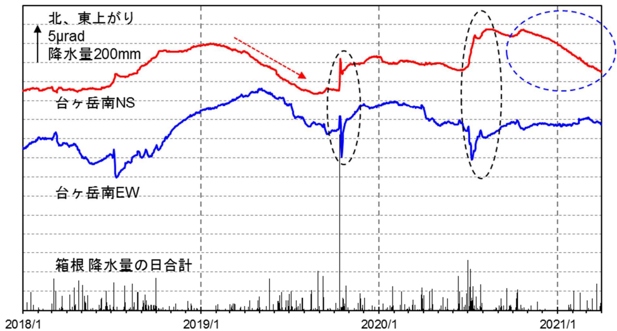
図9 箱根山 台ヶ岳南観測点における傾斜データ（2018年1月1日～2021年3月31日）
