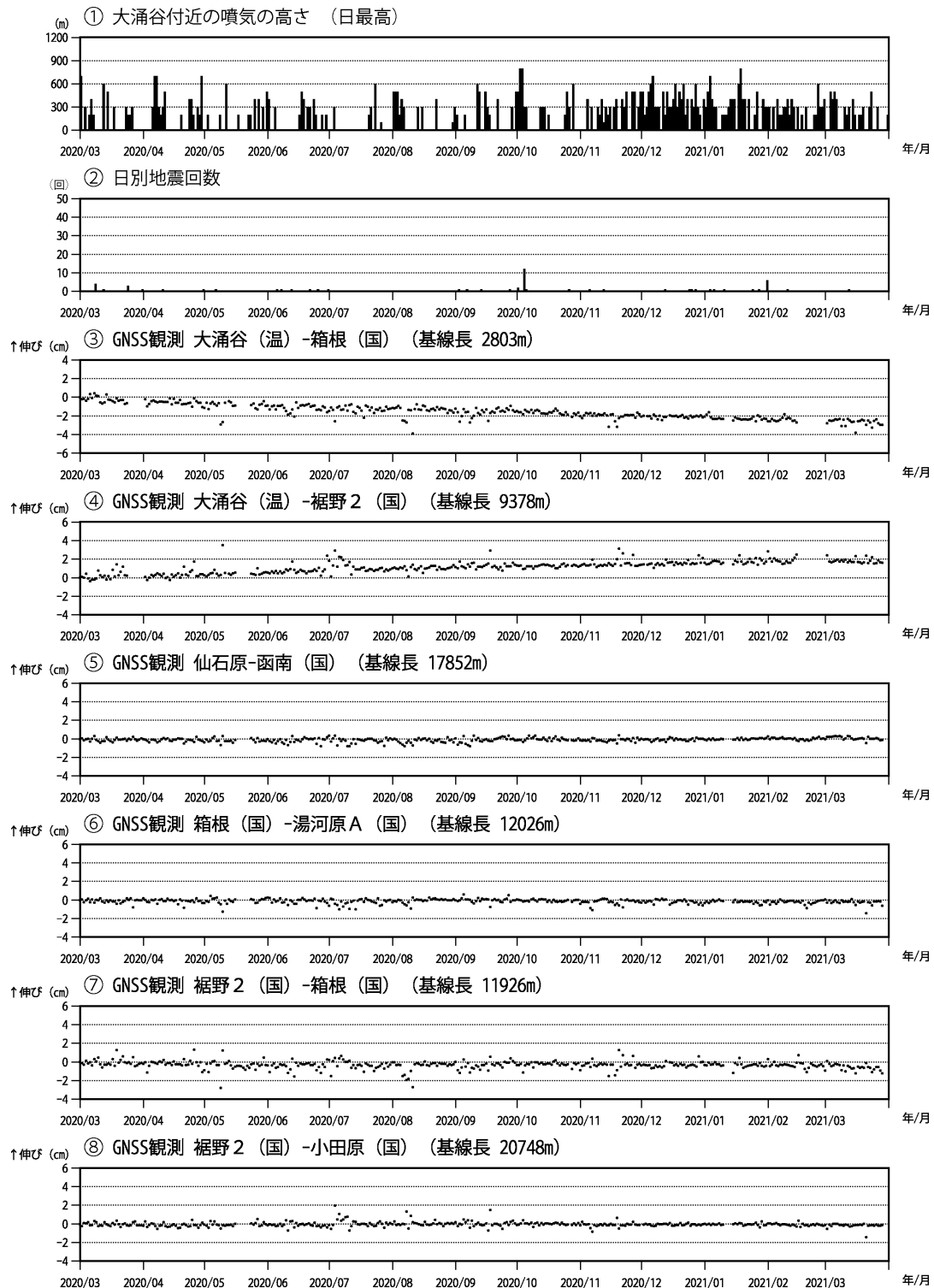
図7 箱根山 火山活動経過図（2020年3月1日～2021年3月31日）
