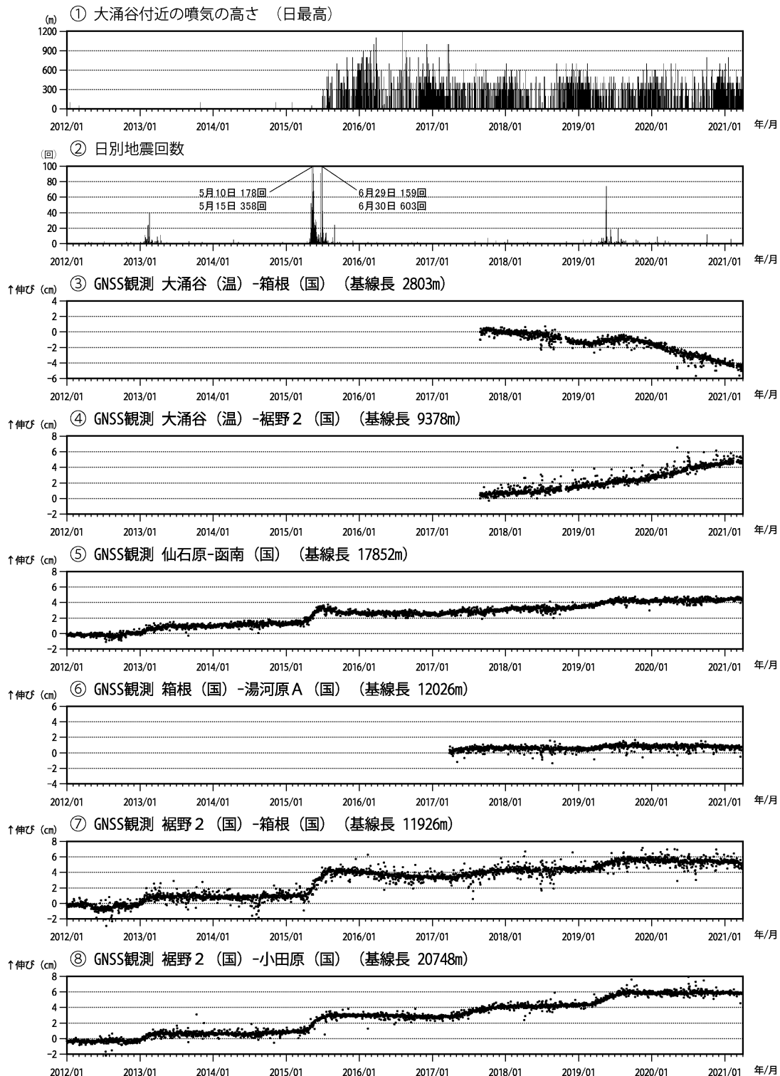
図6 箱根山 火山活動経過図（2012年1月1日～2021年3月31日）
