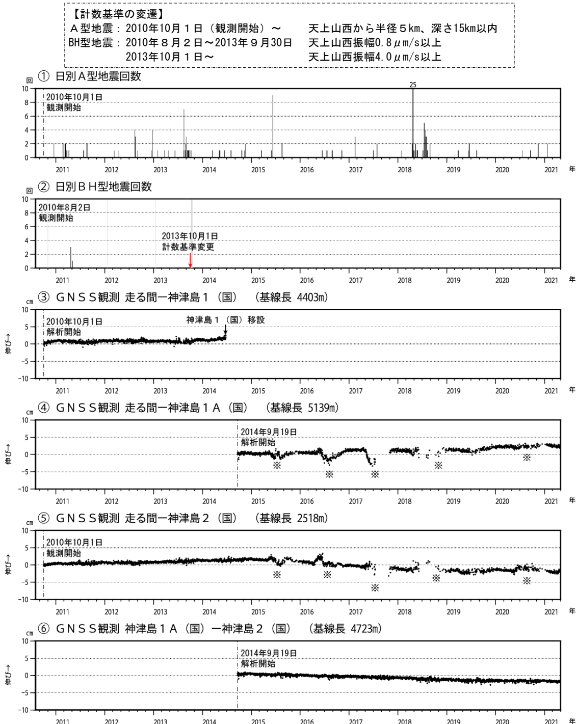
図2 神津島 火山活動経過図(2010年8月2日～2021年4月30日)
