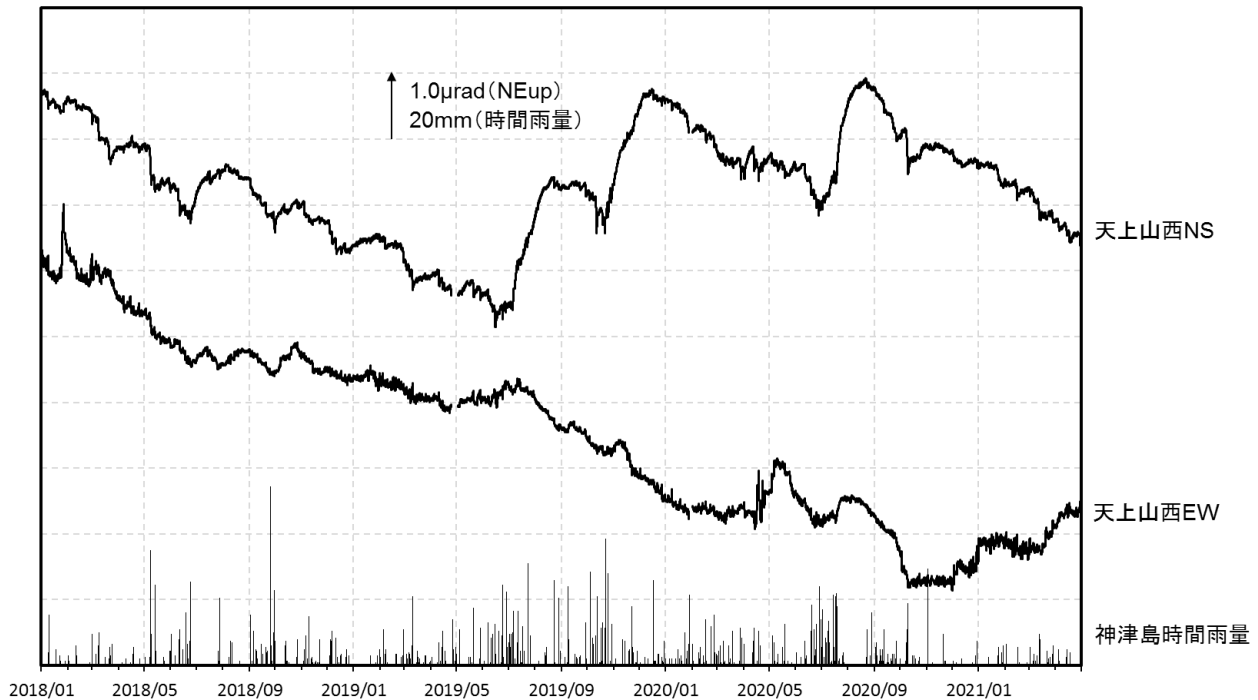
図4 神津島 天上山西観測点の傾斜変動（2018年1月1日～2021年4月30日） 地震等による一部のステップを除去しています。図中の空白部分は欠測を示します。 ・火山活動によるとみられる変動は認められません。
