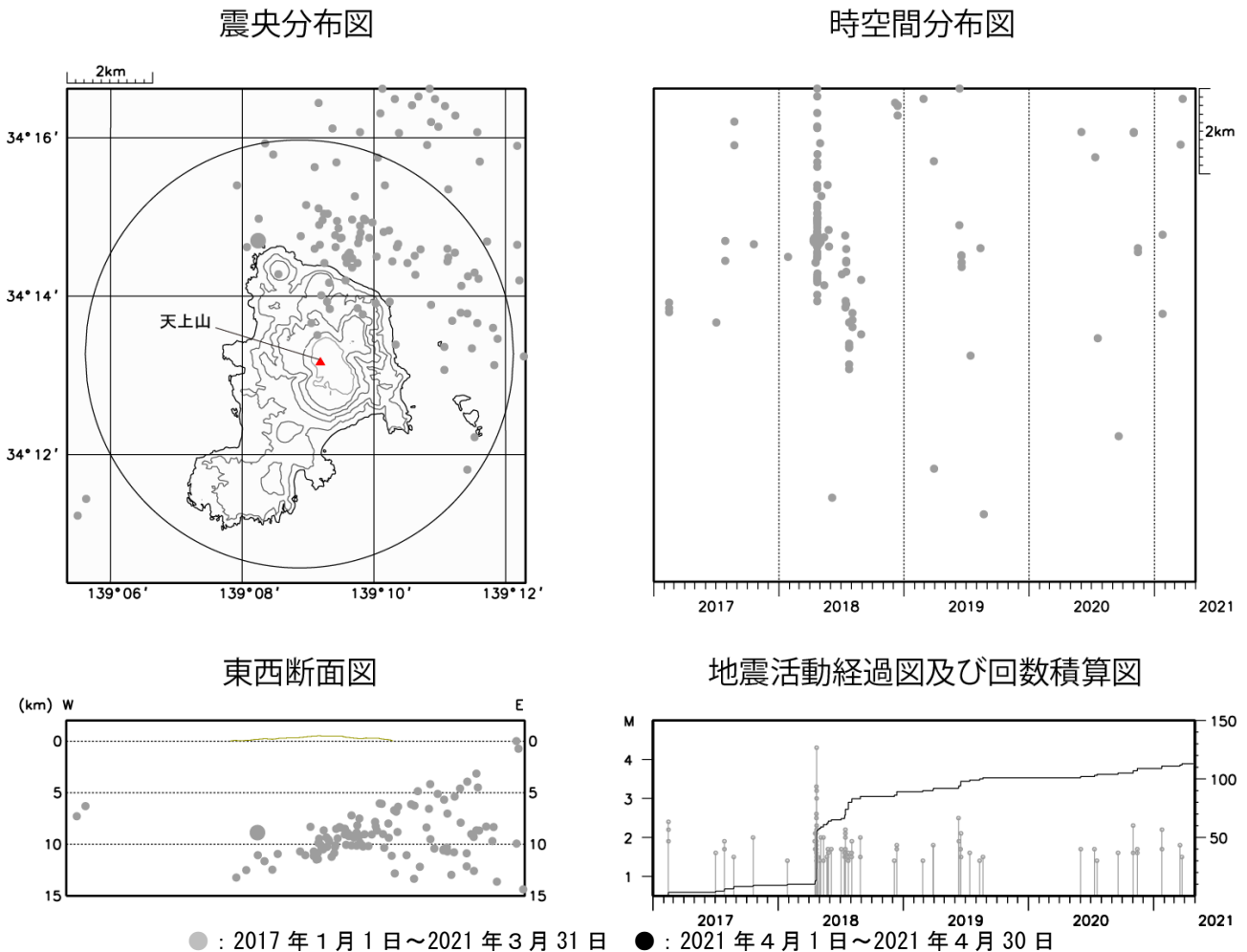
図3 神津島 広域地震観測網による山体・周辺の地震活動（2017年1月1日～2021年4月30日）
