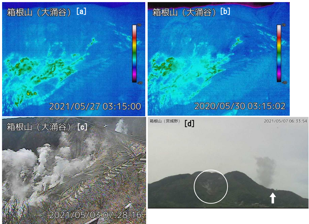
図3 箱根山 大涌谷及び早雲地獄の状況（a～c：大涌谷監視カメラによる、d：宮城野監視カメラによる）
