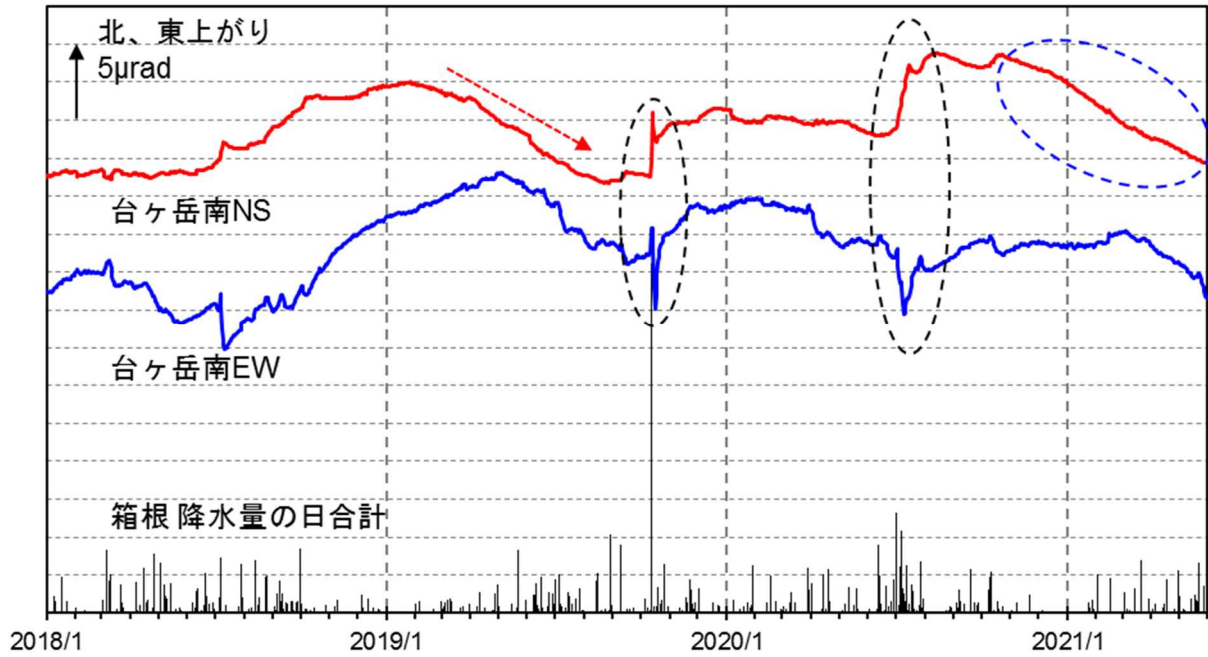
図9 箱根山 台ヶ岳南観測点における傾斜データ（2018年1月1日～2021年5月31日）
