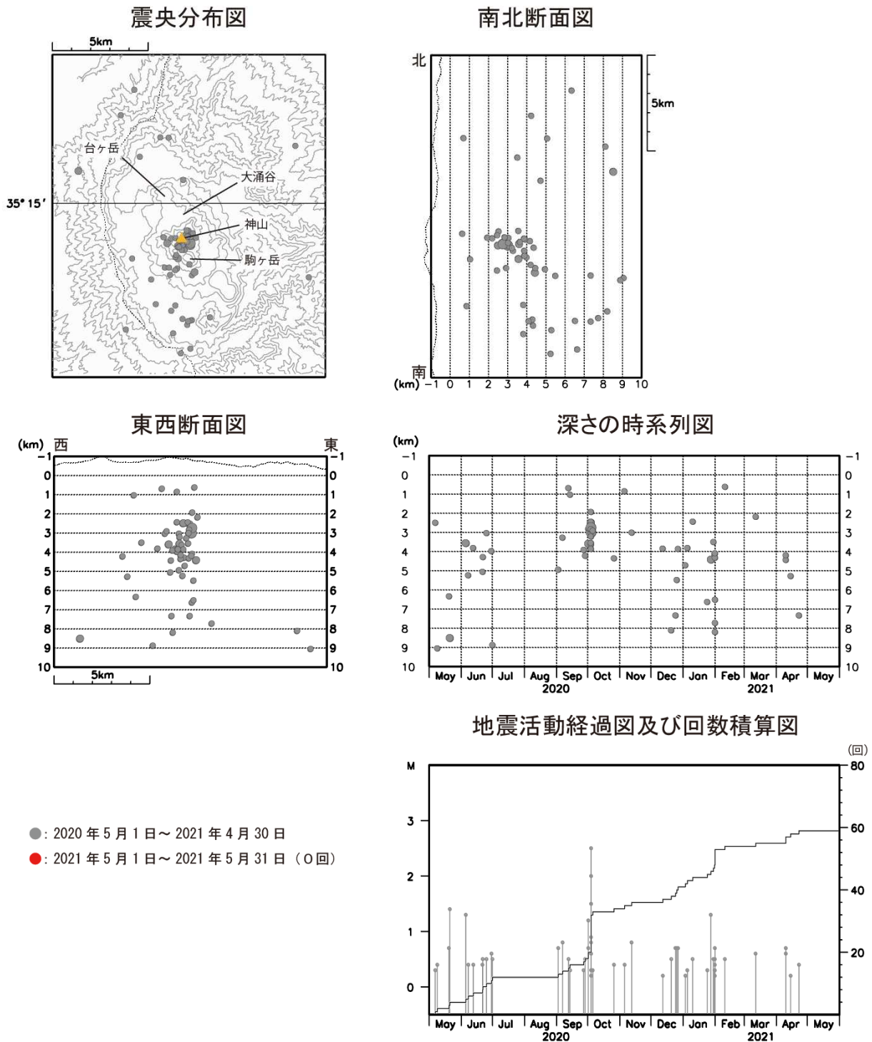
図8 箱根山 広域地震観測網による山体周辺の震源分布図（2020年5月1日～2021年5月31日）
