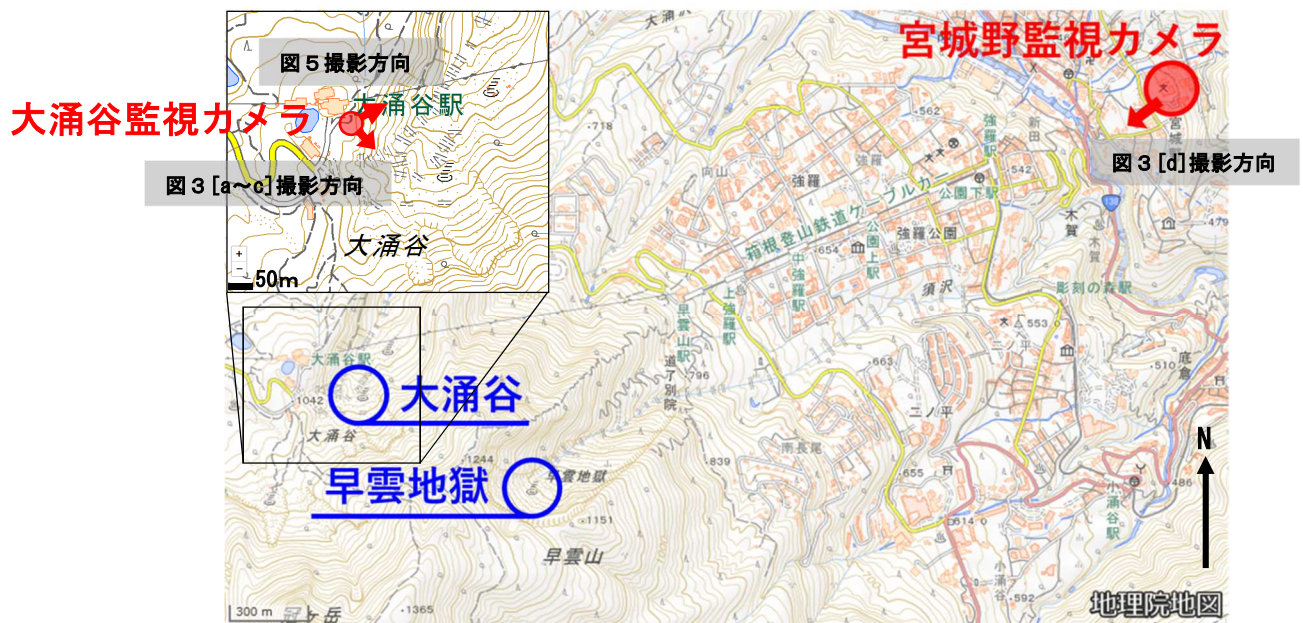
図4 箱根山 噴気場所（大涌谷・早雲地獄）位置図及び図3と図5の撮影場所（地理院地図） 赤丸及び赤矢印は監視カメラ設置場所及びその撮影方向
