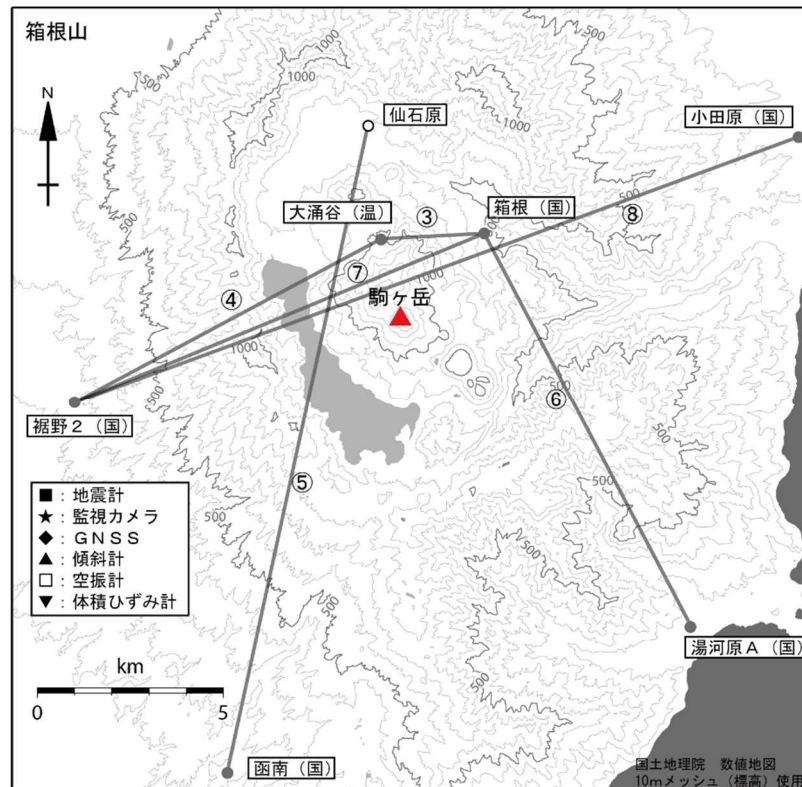
図2 箱根山 GNSS 連続観測点配置図 小さな白丸（○）は気象庁、小さな黒丸（●）は気象庁以外の観測点を示しています。 （国）：国土地理院、（温）：神奈川県温泉地学研究所 GNSS 基線③～⑧は図5及び図6の③～⑧に対応しています。
