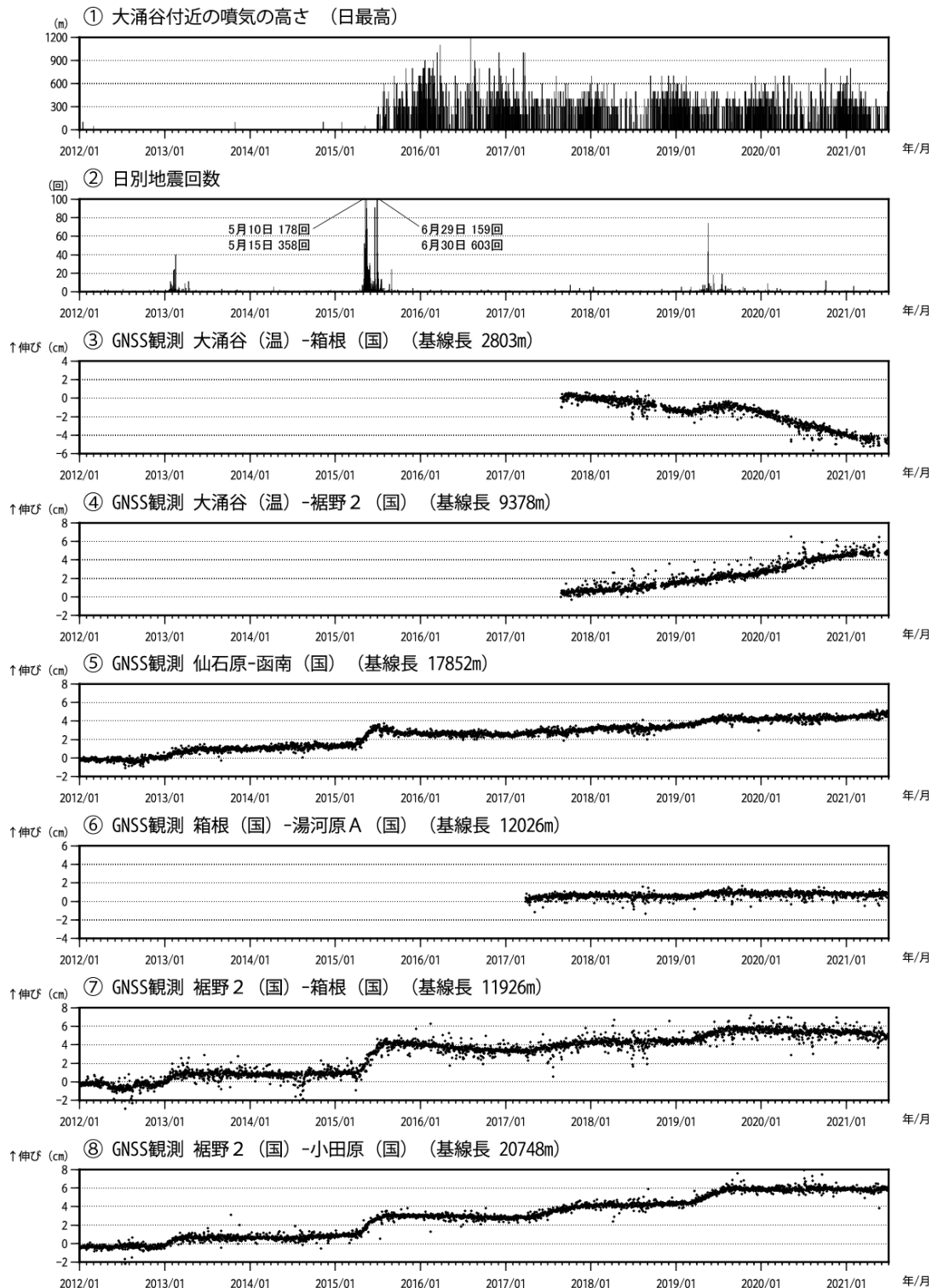
図5 箱根山 火山活動経過図（2012年1月1日～2021年6月30日）
