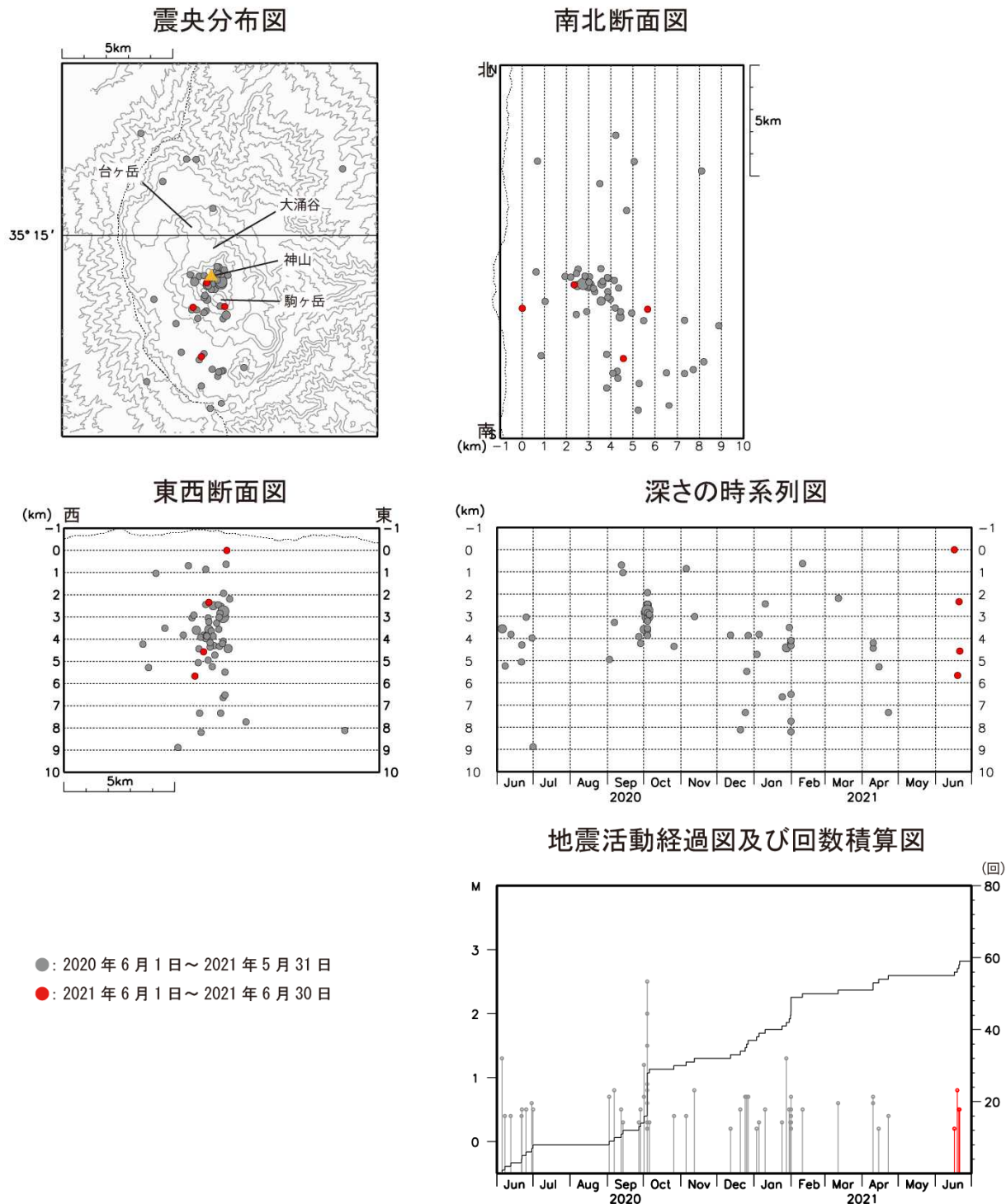
図7 箱根山 広域地震観測網による山体周辺の震源分布図（2020年6月1日～2021年6月30日）
