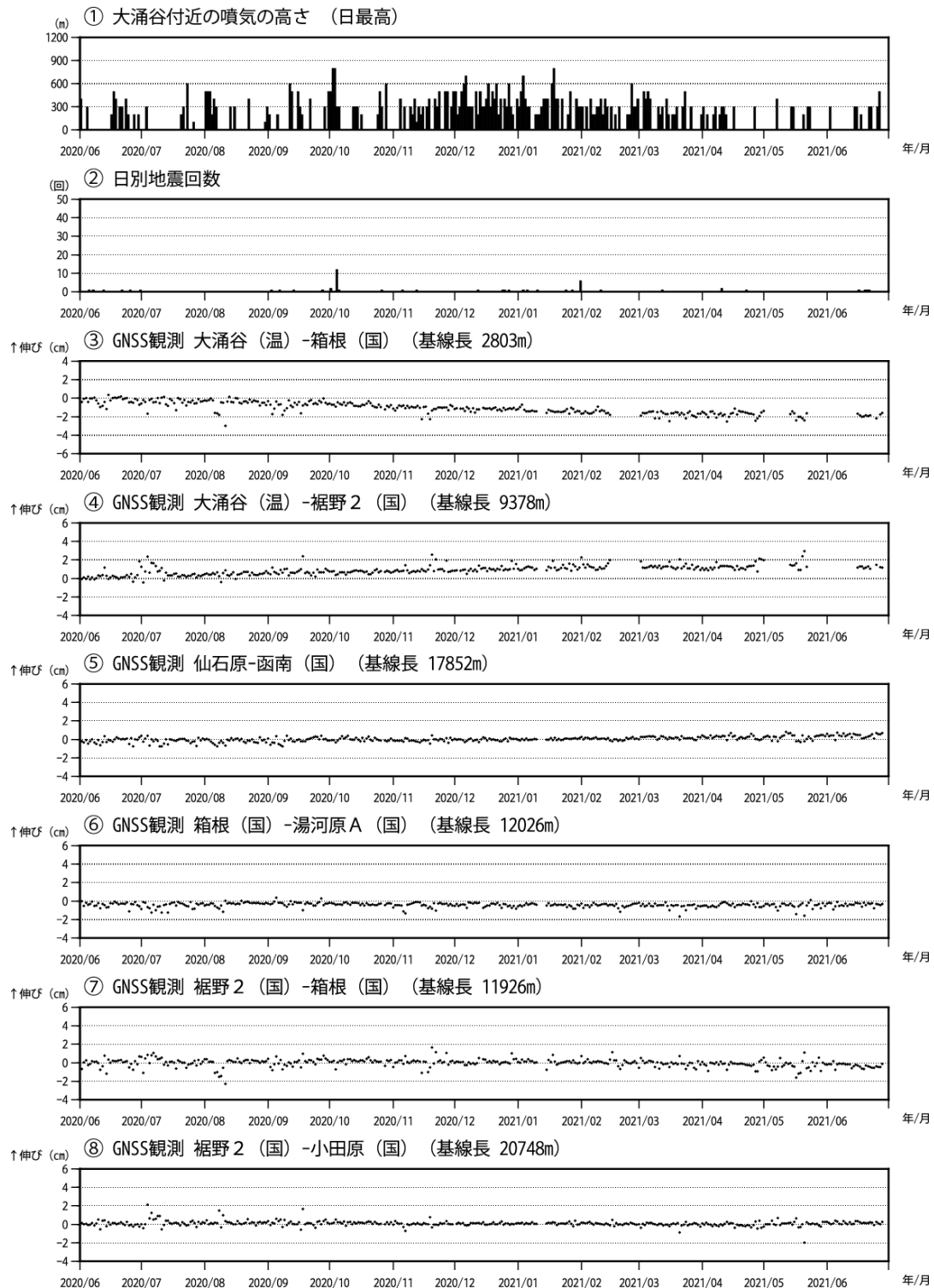
図6 箱根山 火山活動経過図（2020年6月1日～2021年6月30日）
