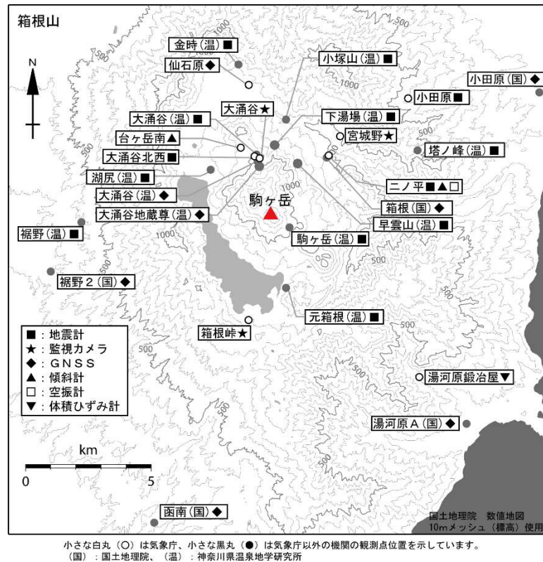
図1 箱根山 観測点配置図 小さな白丸（○）は気象庁、小さな黒丸（●）は気象庁以外の観測点を示しています。 （国）：国土地理院、（温）：神奈川県温泉地学研究所
