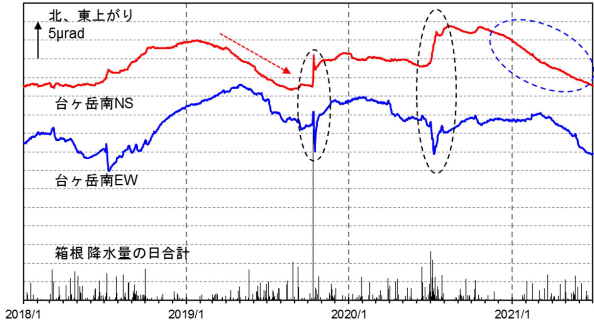
図8 箱根山 台ヶ岳南観測点における傾斜データ（2018年1月1日～2021年6月30日）
