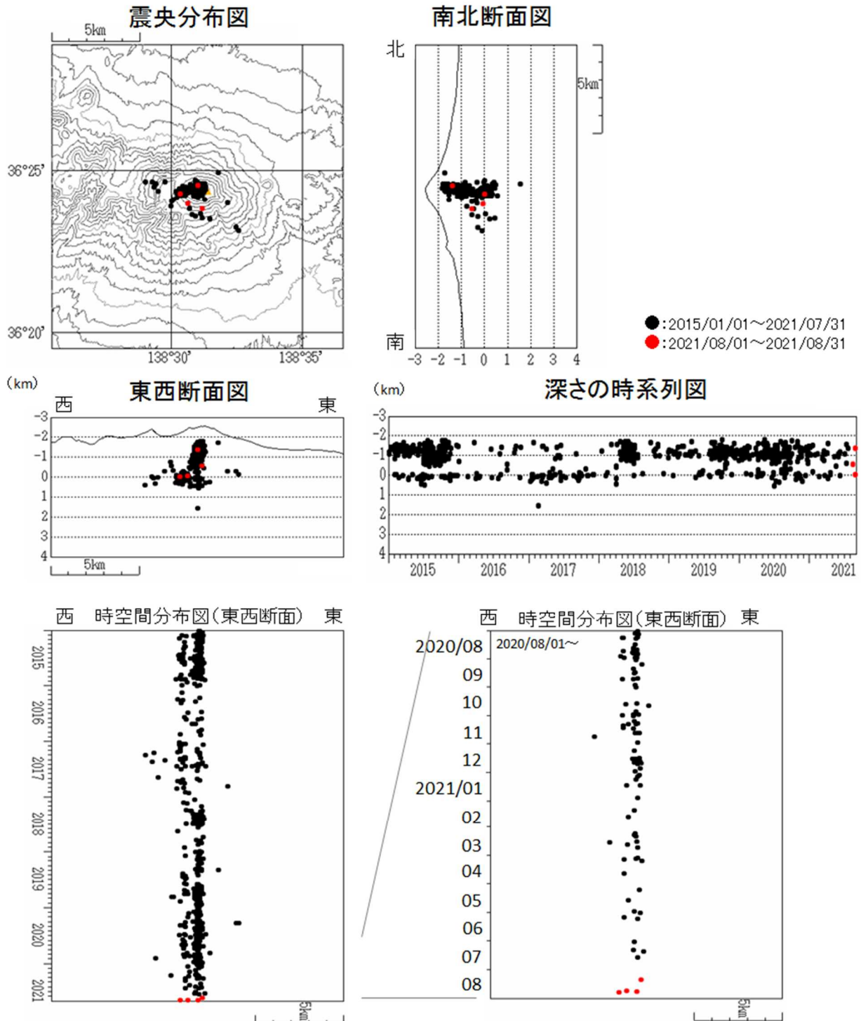
図5 浅間山 震源分布図（2015年1月1日～2021年8月31日） ・火山性地震の震源は、従来からみられている山頂直下の海拔0～2 km 付近に分布しています。
