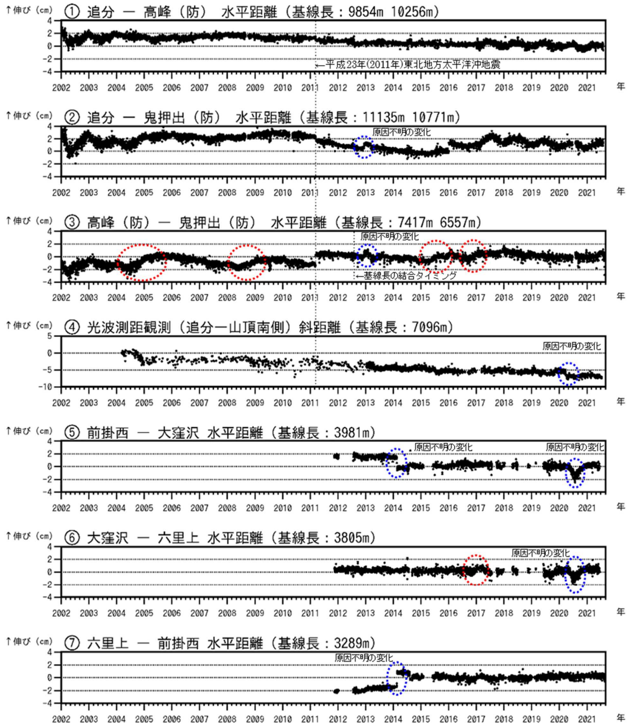
図6-1 浅間山 GNSS連続観測及び光波測距観測の結果(2002年1月1日~2021年8月31日)
