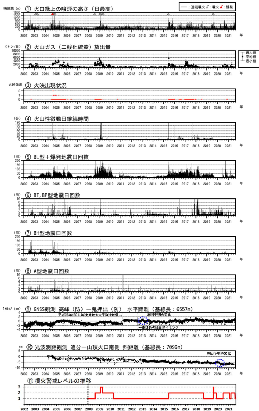
図4 浅間山 火山活動経過図（2002年1月1日～2021年8月31日）
