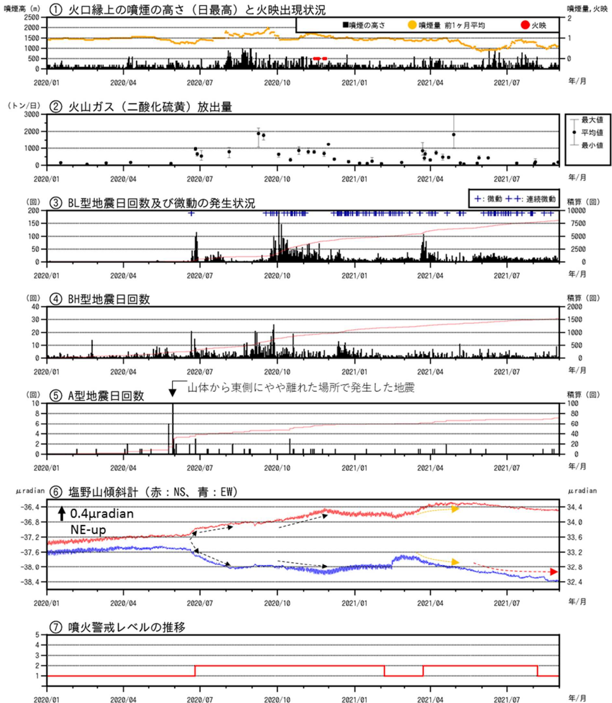
図3 浅間山 火山活動経過図（2020年1月1日～2021年8月31日）
