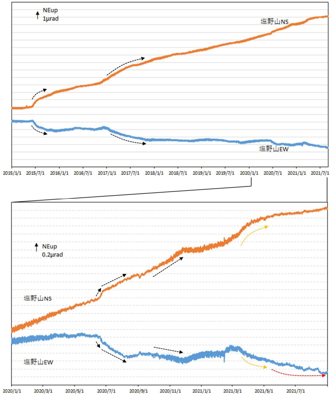
図8 浅間山 塩野山観測点における傾斜データ（2015年1月1日～2021年8月31日）
