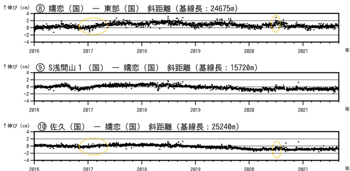
図6-2 浅間山 GNSS連続観測結果(2016年1月1日~2021年8月31日)
