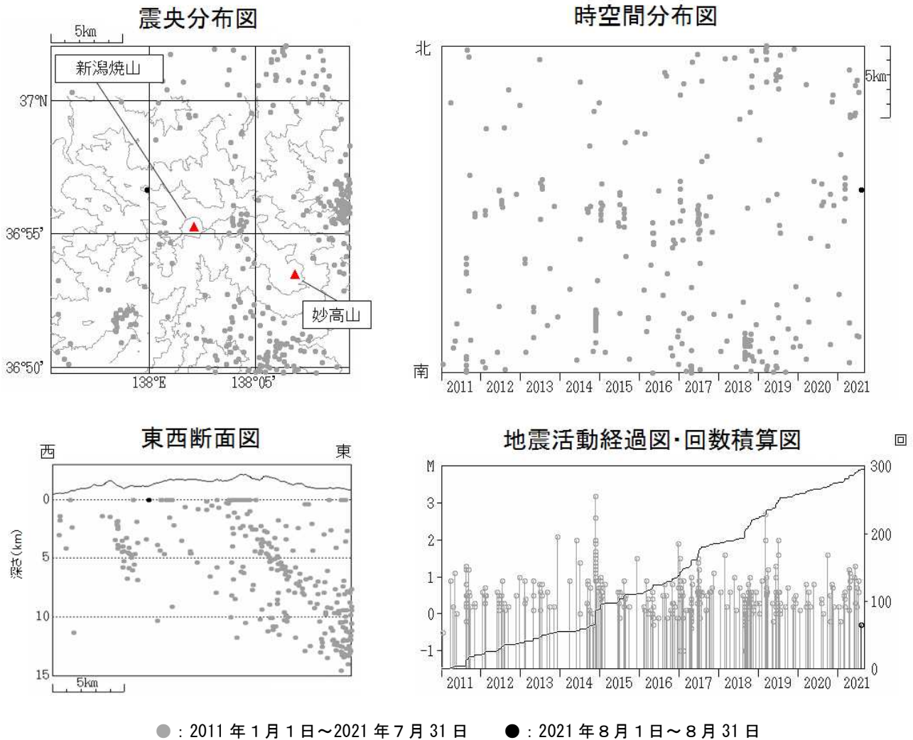
図4 新潟焼山 広域地震観測網による山体・周辺の地震活動（2011 年 1 月 1 日～2021 年 8 月 31 日）
