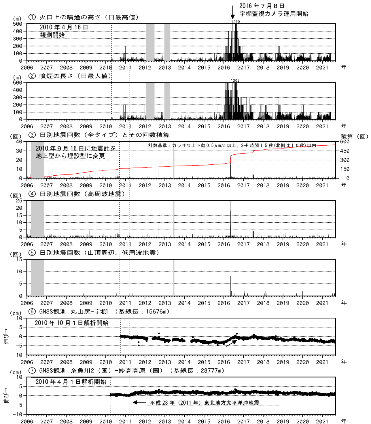
図2 新潟焼山 火山活動経過図（2006年1月1日～2021年8月31日）
