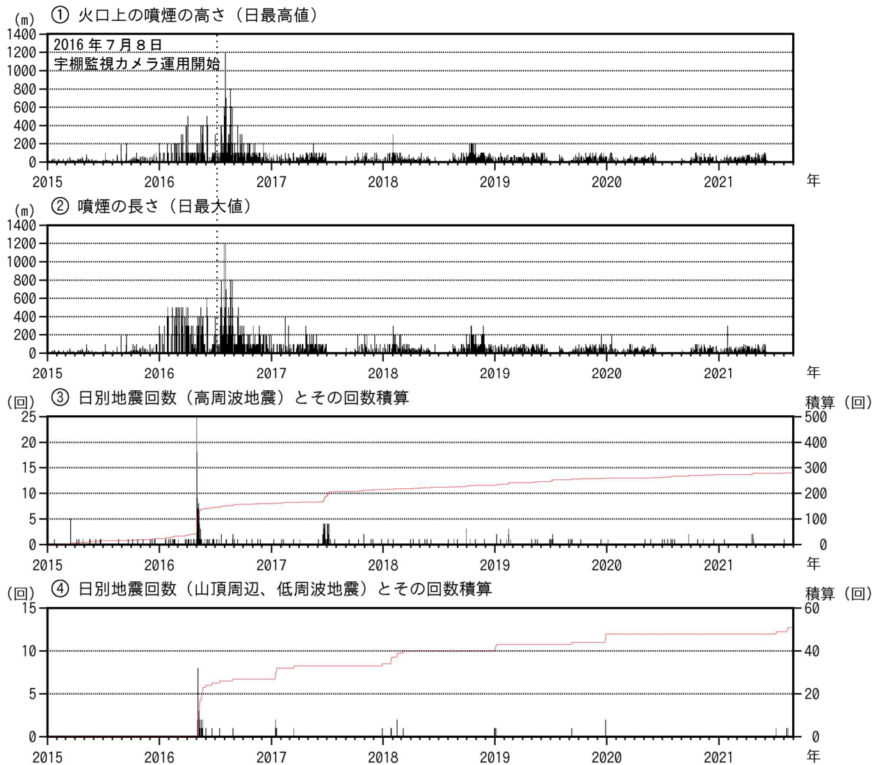
図3 新潟焼山 火山活動経過図（短期）（2015年1月1日～2021年8月31日）
