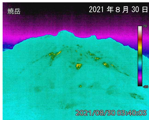
図3 焼岳 中尾峠赤外熱映像カメラによる焼岳の北側斜面の地表面温度分布と可視画像 撮影場所と撮影方向は図15を参照下さい。
