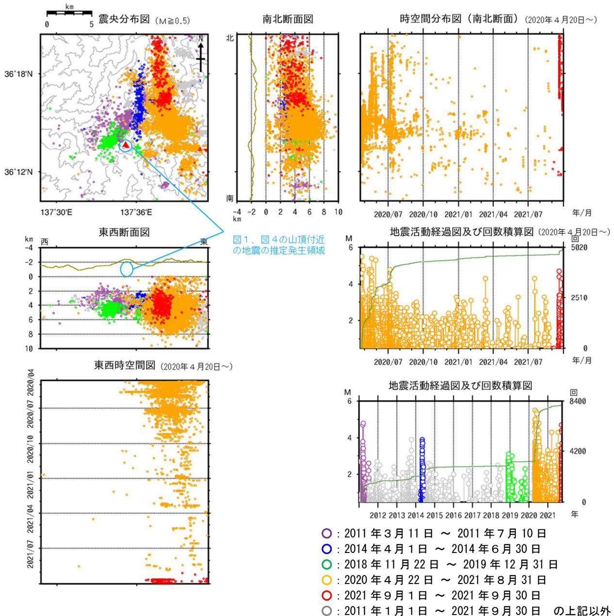
図8 焼岳 広域地震観測網による山体及び周辺の地震活動(2011年1月1日～2021年9月30日)
