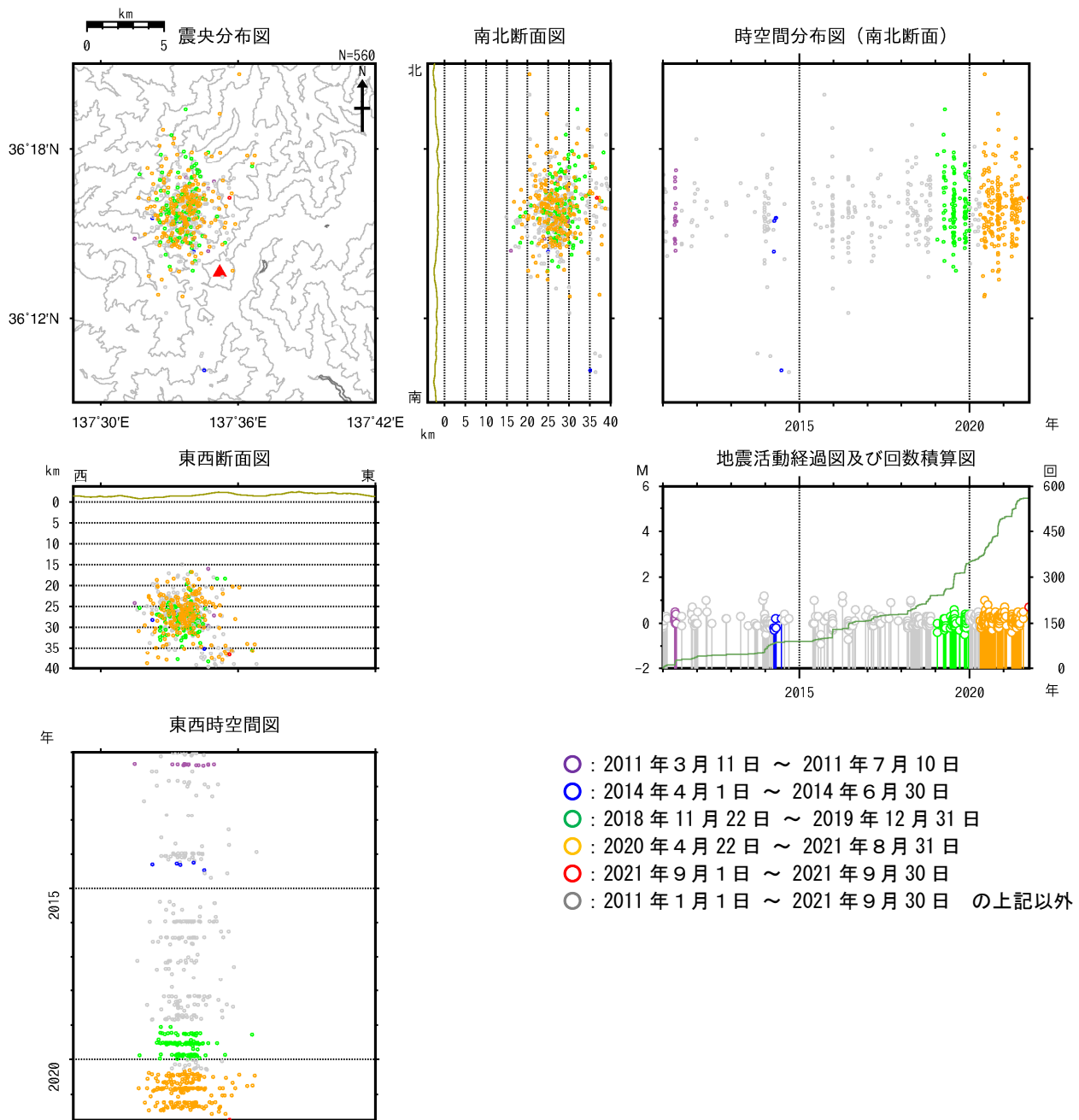
図9 焼岳 広域地震観測網による深部低周波地震の震源分布図（2011年1月1日～2021年9月30日） 広域地震観測網により震源決定したもので、深さは全て海面以下として決定しています。そのため、山頂付近の浅い地震の震源も海面下に決定されています。
