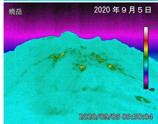
図3 焼岳 中尾峠赤外熱映像カメラによる焼岳の北側斜面の地表面温度分布と可視画像 撮影場所と撮影方向は図15を参照下さい。
