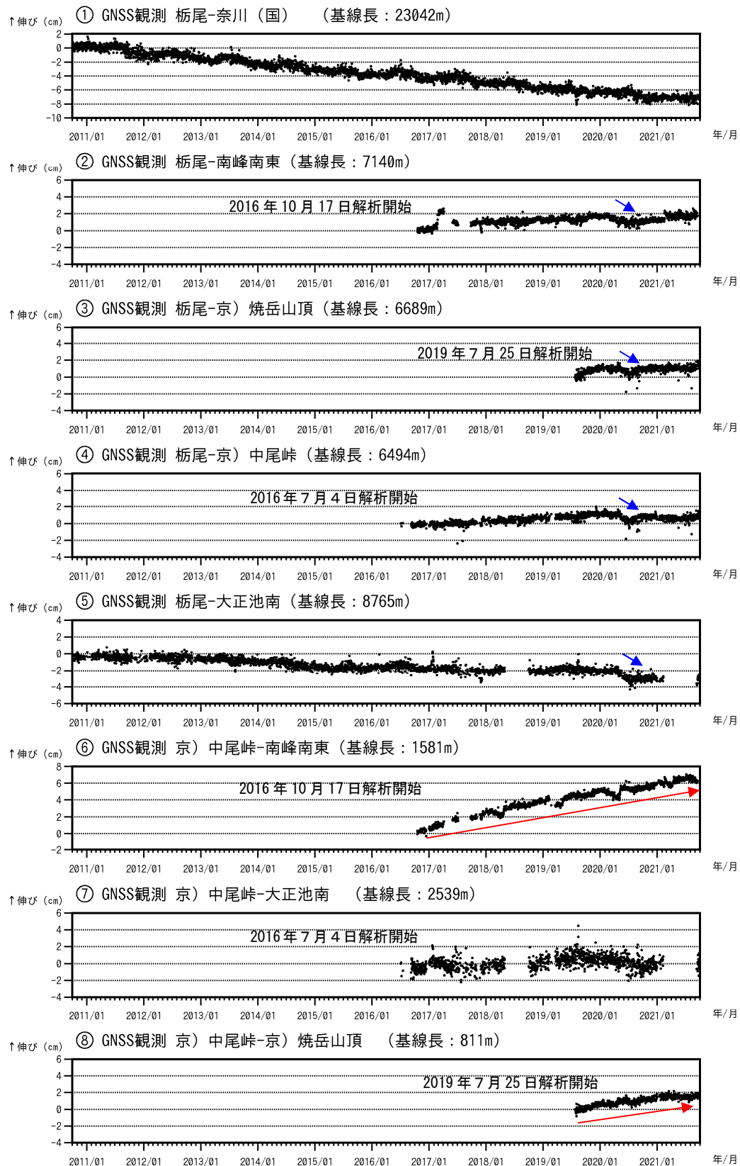
図5 焼岳 GNSS連続観測による基線長変化（2010年10月1日～2021年9月30日）
