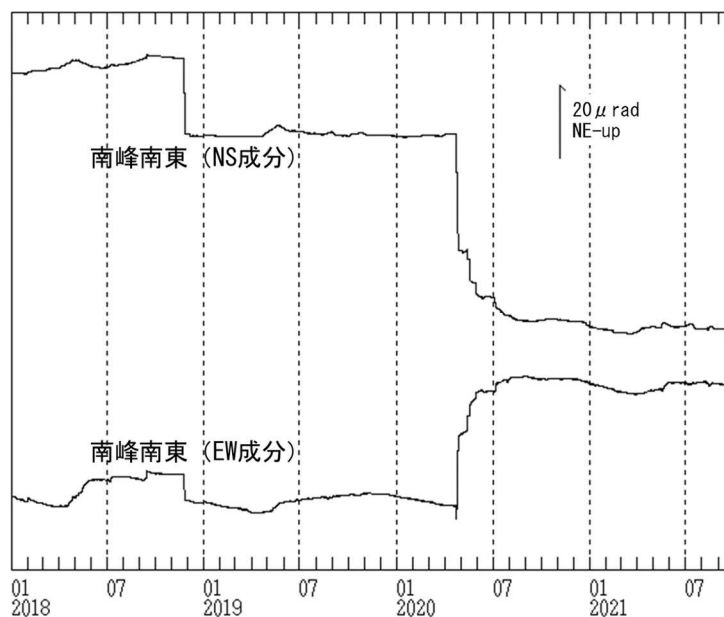
図7 焼岳 南峰南東観測点における傾斜データ（2018年1月1日～2021年9月30日）
