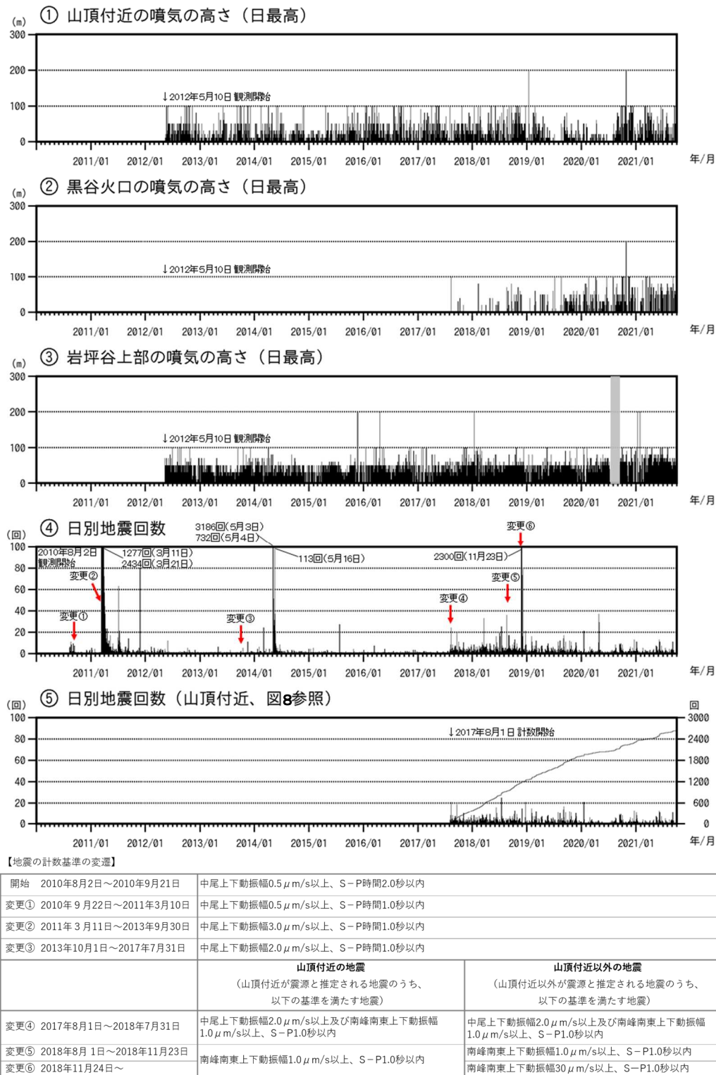
図4 焼岳 噴気の高さと地震回数の推移(2010年8月2日～2021年9月30日)
