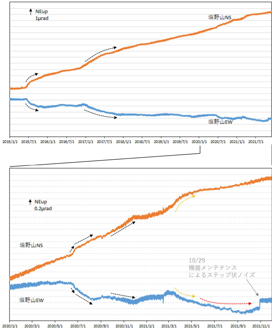
図8 浅間山 塩野山観測点における傾斜データ（2015年1月1日～2021年11月30日） データは時間平均値を使用しており、長期にわたるトレンドを補正しています。 下段は上段に比べて縦軸を拡大しています。
