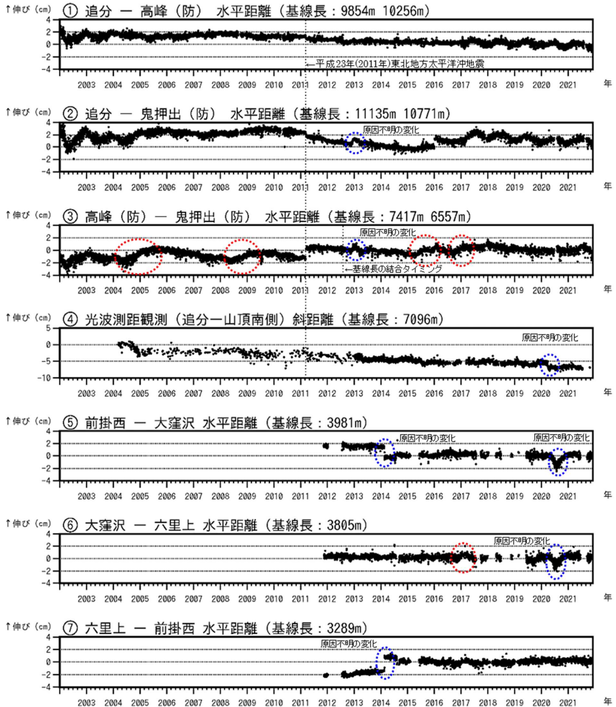
図6-1 浅間山 GNSS 連続観測及び光波測距観測の結果(2002年1月1日～2021年11月30日) 2010年10月及び2016年1月に解析方法を変更しています。
