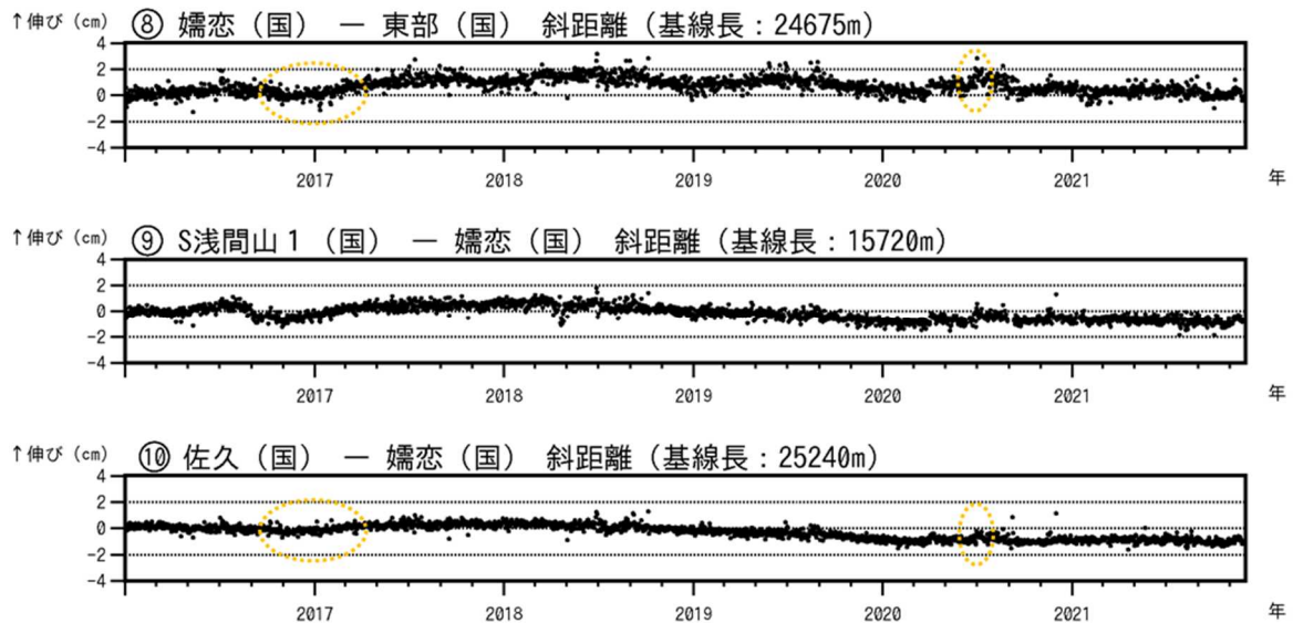
図6-2 浅間山 GNSS 連続観測結果(2016年1月1日~2021年11月30日)
