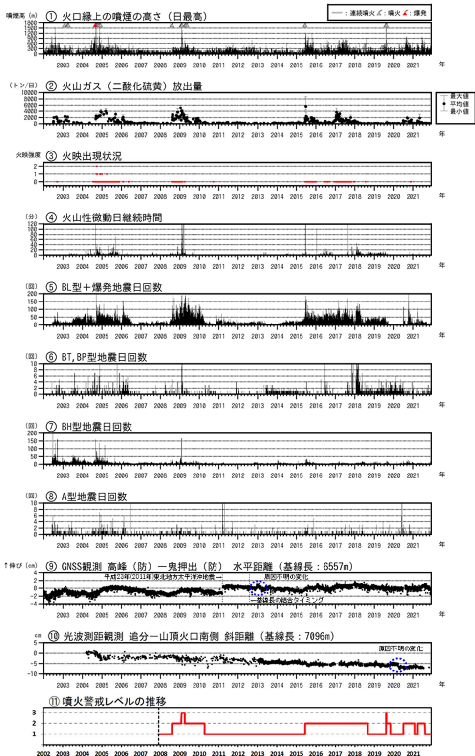
図4 浅間山 火山活動経過図（2002年1月1日～2021年11月30日）
