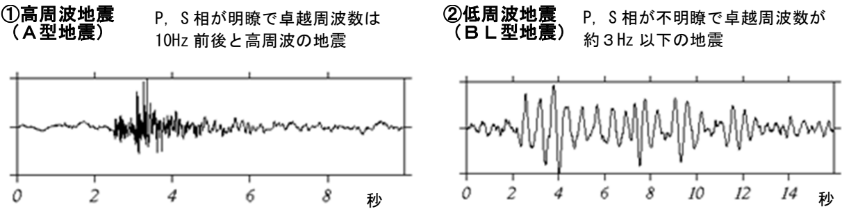
図6 新潟焼山 火山性地震の特徴と波形例
