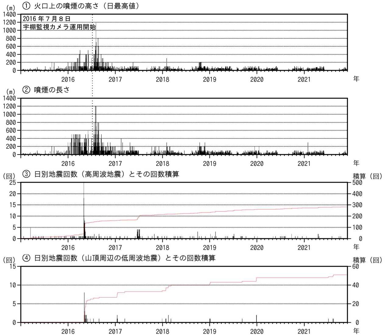
図3 新潟焼山 火山活動経過図（短期）（2015年1月1日～2021年11月30日）
