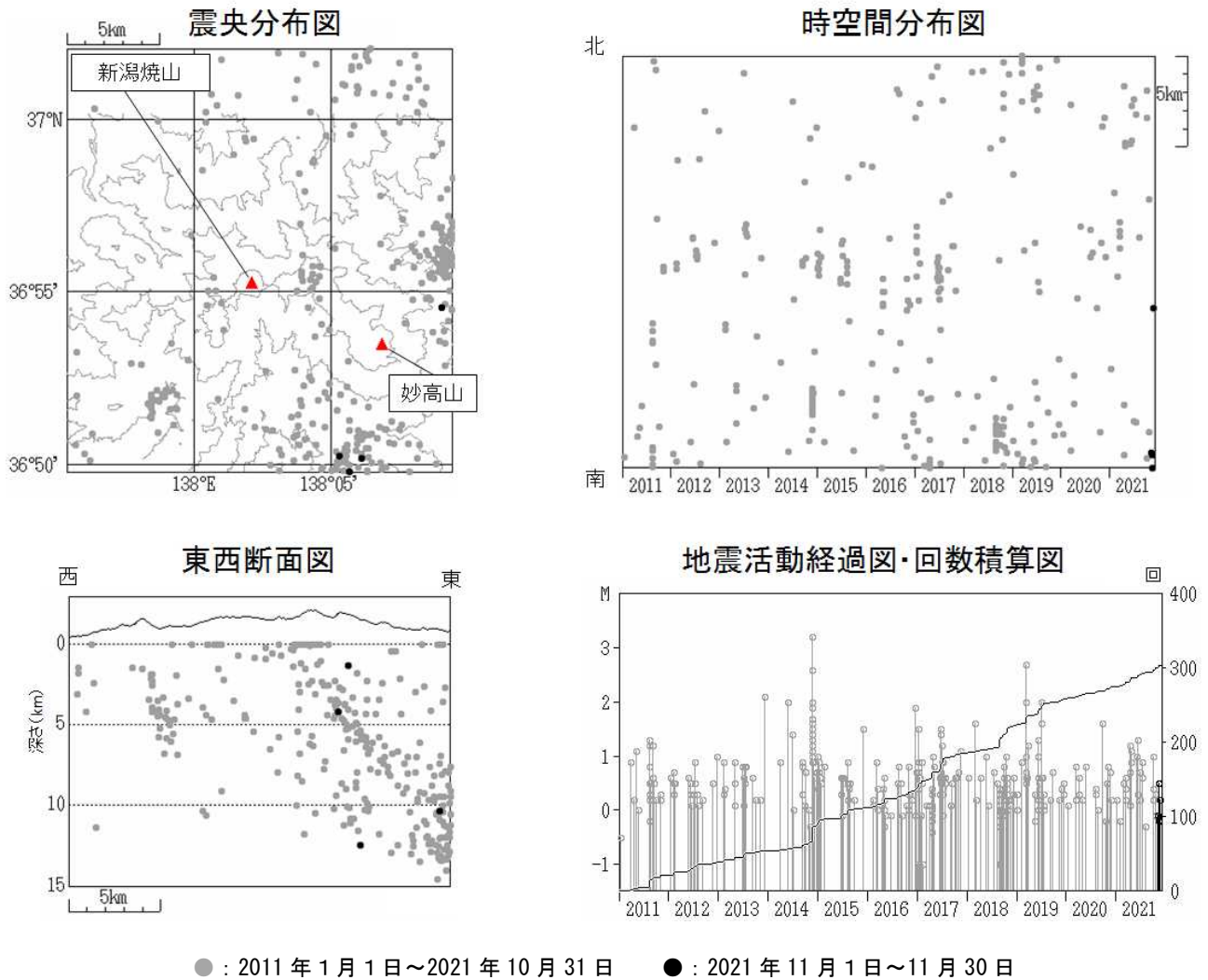
図4 新潟焼山 広域地震観測網による山体・周辺の地震活動(2011年1月1日～2021年11月30日)
