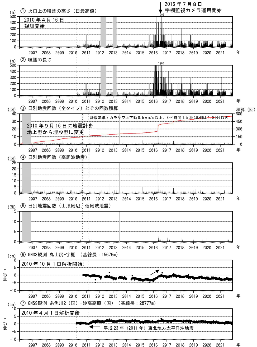
図2 新潟焼山 火山活動経過図（2006年1月1日～2021年11月30日）
