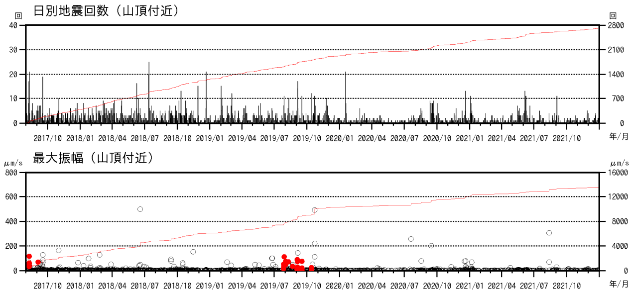
図1 焼岳 山頂付近の地震回数、及び南峰南東観測点上下動最大振幅 (2017年8月1日～2021年12月31日)
