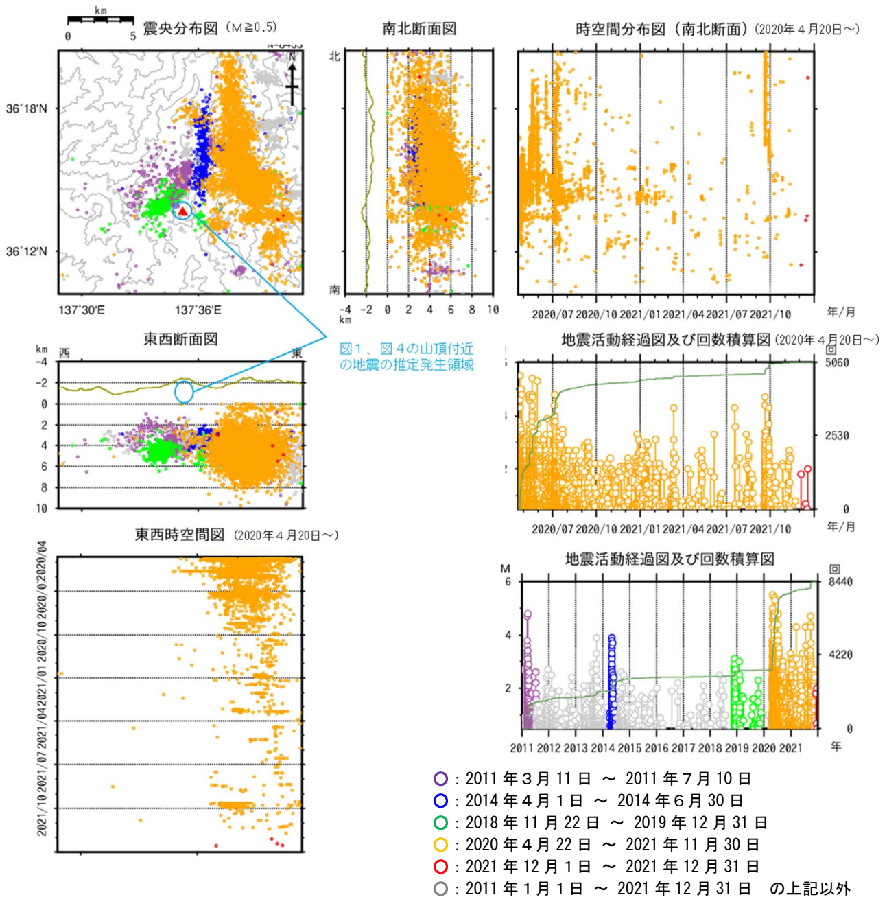
図8 焼岳 広域地震観測網による山体及び周辺の地震活動(2011年1月1日～2021年12月31日)
