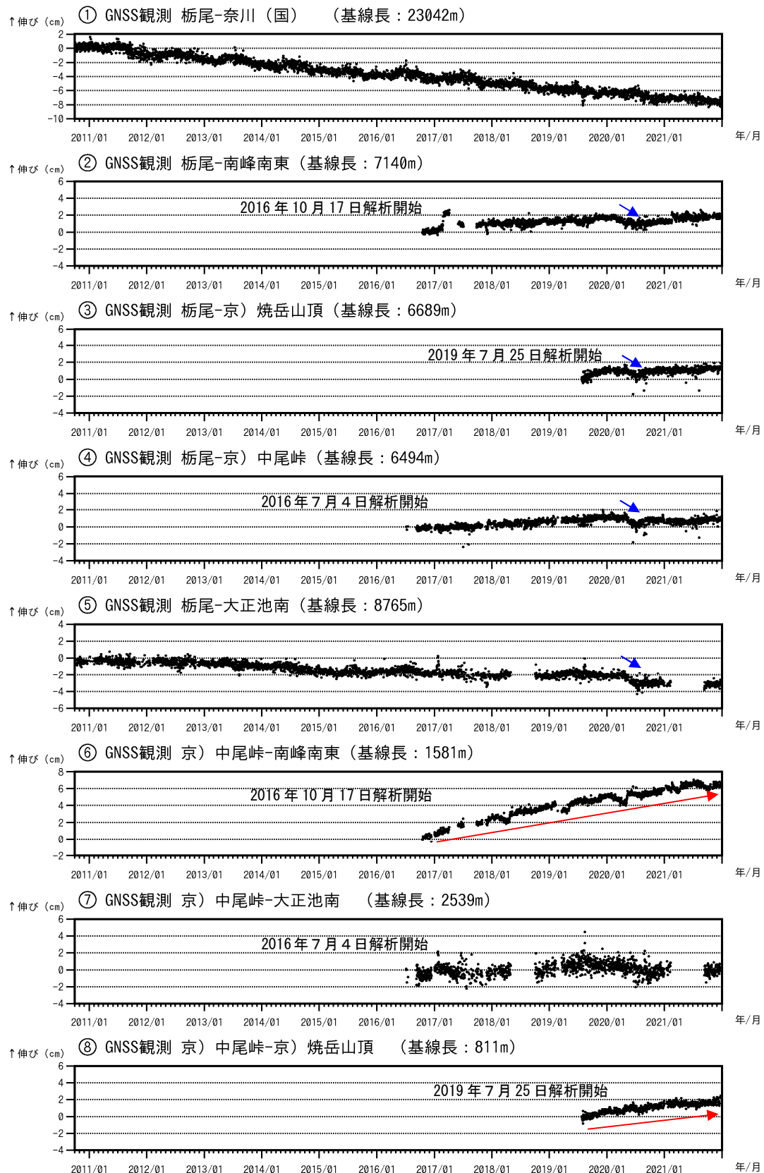
図5 焼岳 GNSS連続観測による基線長変化 (2010年10月1日~2021年12月31日)
