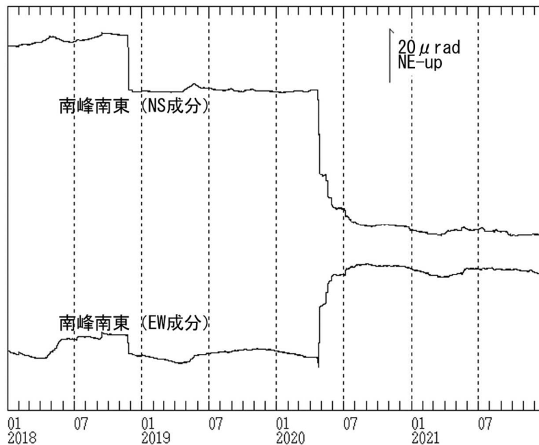
図7 焼岳 南峰南東観測点における傾斜データ（2018年1月1日～2021年12月31日）
