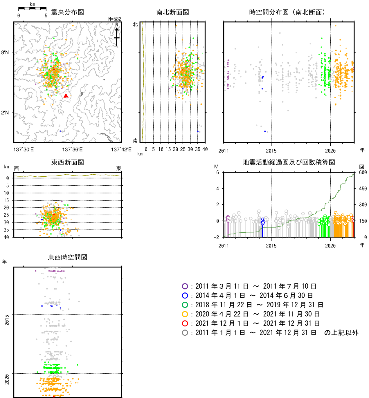
図9 焼岳 広域地震観測網による深部低周波地震の震源分布図（2011年1月1日～2021年12月31日） 広域地震観測網により震源決定したもので、深さは全て海面以下として決定しています。そのため、山頂付近の浅い地震の震源も海面下に決定されています。 M（マグニチュード）は地震の規模を表します。 図中の震源要素は一部暫定値が含まれており、後日変更することがあります。 2022年1月12日現在、次の期間の地震について、暫定的に震源精査の基準を変更しているため、その前後の期間と比較して微小な地震での震源決定数の変化（増減）が見られます。 (1)2020年9月1日から10月23日まで、(2)2021年1月9日から3月7日まで、(3)2021年4月19日から12月5日
