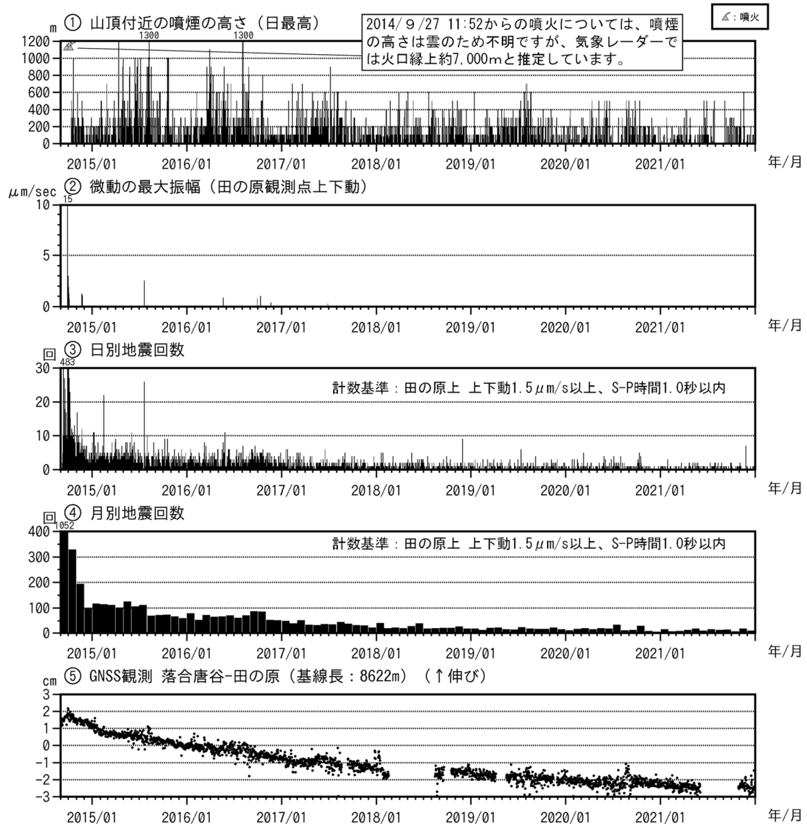
図4 御嶽山 最近の火山活動経過図（2014年9月1日～2021年12月31日）
