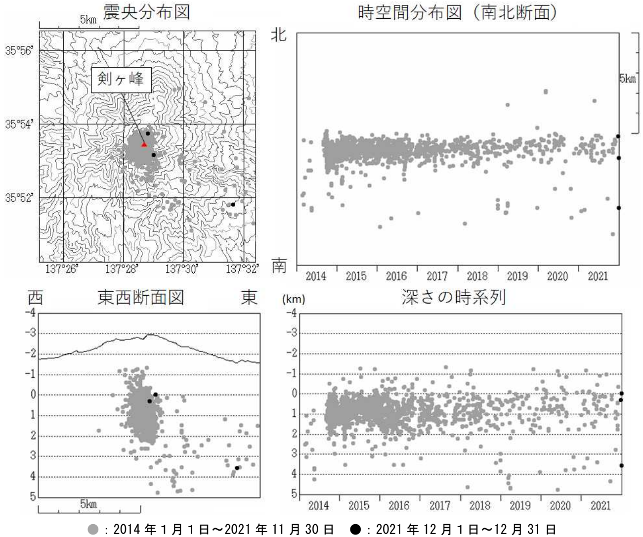
図3 御嶽山 震源分布図（2014年1月1日～2021年12月31日）
