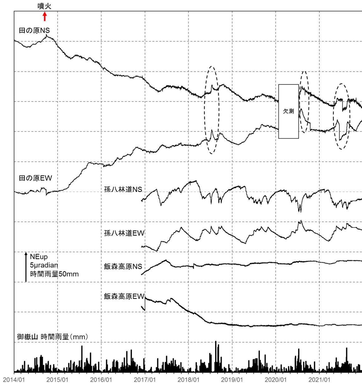
図7 御嶽山 傾斜変動（2014年1月1日～2021年12月31日）
