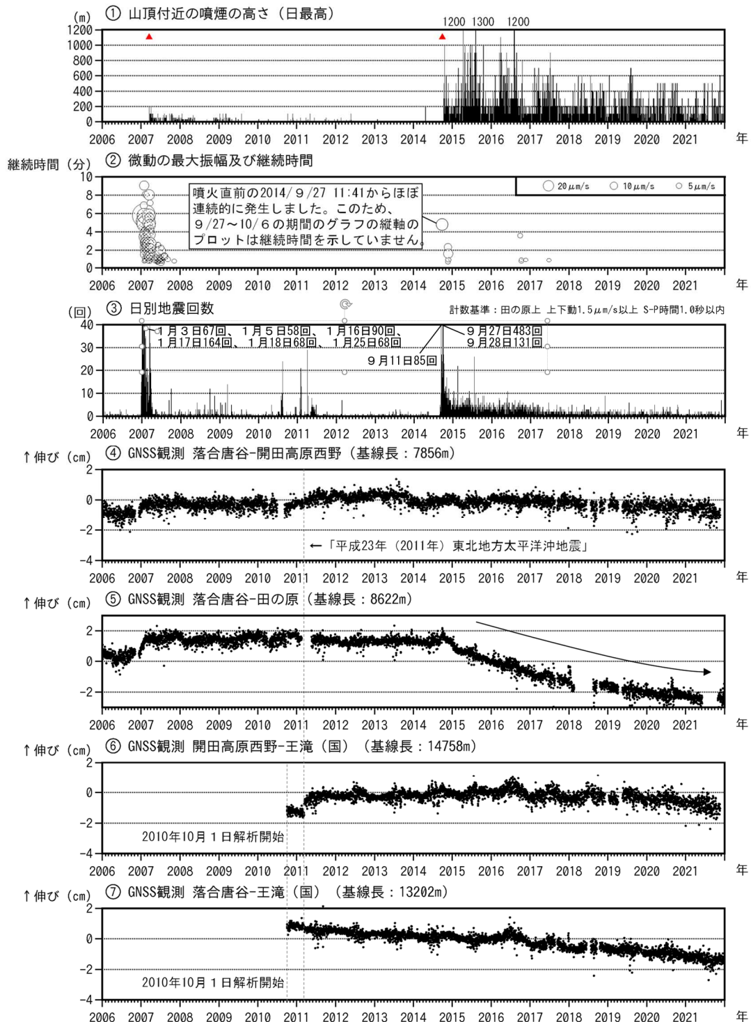
図5 御嶽山 長期間の火山活動経過図（2006年1月1日～2021年12月31日）
