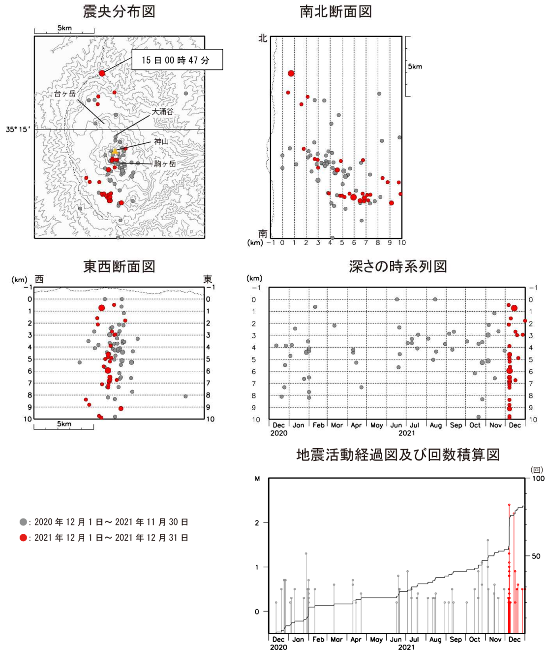
図4 箱根山 広域地震観測網による山体周辺の震源分布図（2020年12月1日～2021年12月31日）
