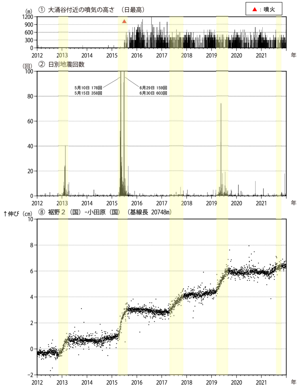
図3-1 箱根山 火山活動経過図（2012年1月1日～2021年12月31日）
