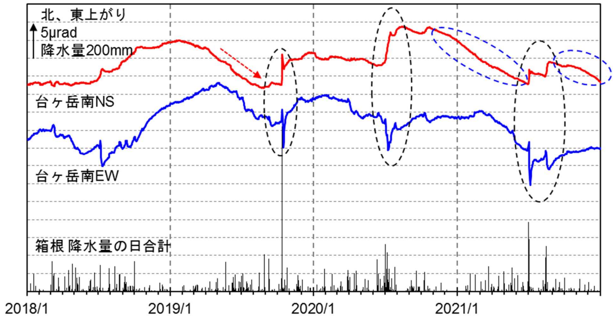
図5 箱根山 台ヶ岳南観測点における傾斜データ（2018年1月1日～2021年12月31日）
