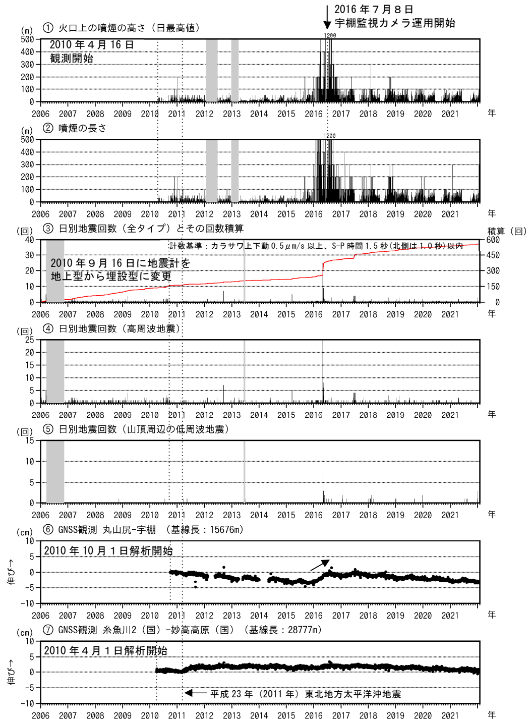
図2 新潟焼山 火山活動経過図（2006年1月1日～2022年1月31日）
