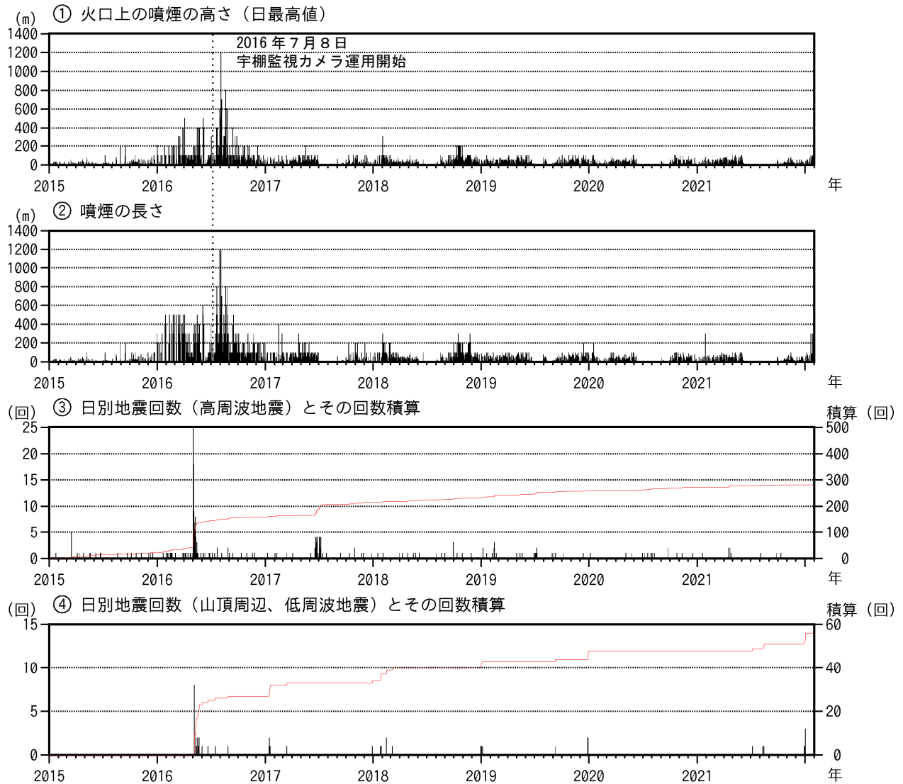
図3 新潟焼山 火山活動経過図（短期）（2015年1月1日～2022年1月31日）
