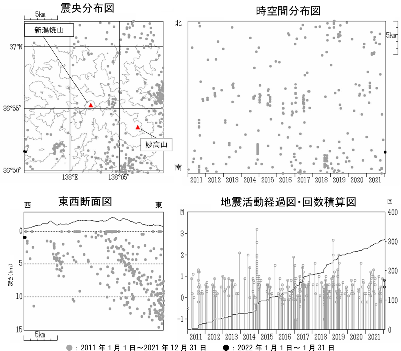
図4 新潟焼山 広域地震観測網による山体・周辺の地震活動（2011 年 1 月 1 日～2022 年 1 月 31 日）
