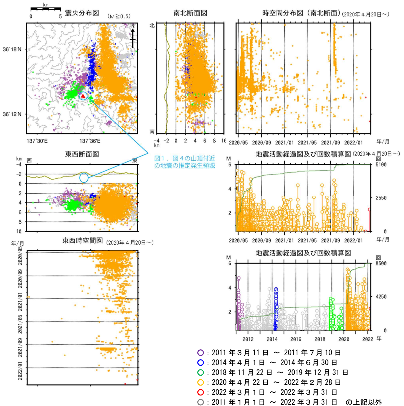
図8 焼岳 広域地震観測網による山体及び周辺の地震活動(2011年1月1日～2022年3月31日)
