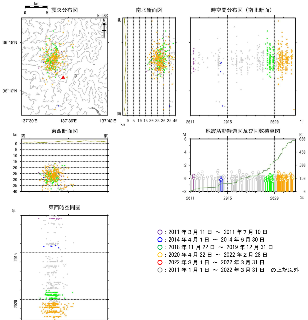
図9 焼岳 広域地震観測網による深部低周波地震の震源分布図（2011年1月1日～2022年3月31日） 広域地震観測網により震源決定したもので、深さは全て海面以下として決定しています。そのため、山頂付近の浅い地震の震源も海面下に決定されています。 M（マグニチュード）は地震の規模を表します。 図中の震源要素は一部暫定値が含まれており、後日変更することがあります。
