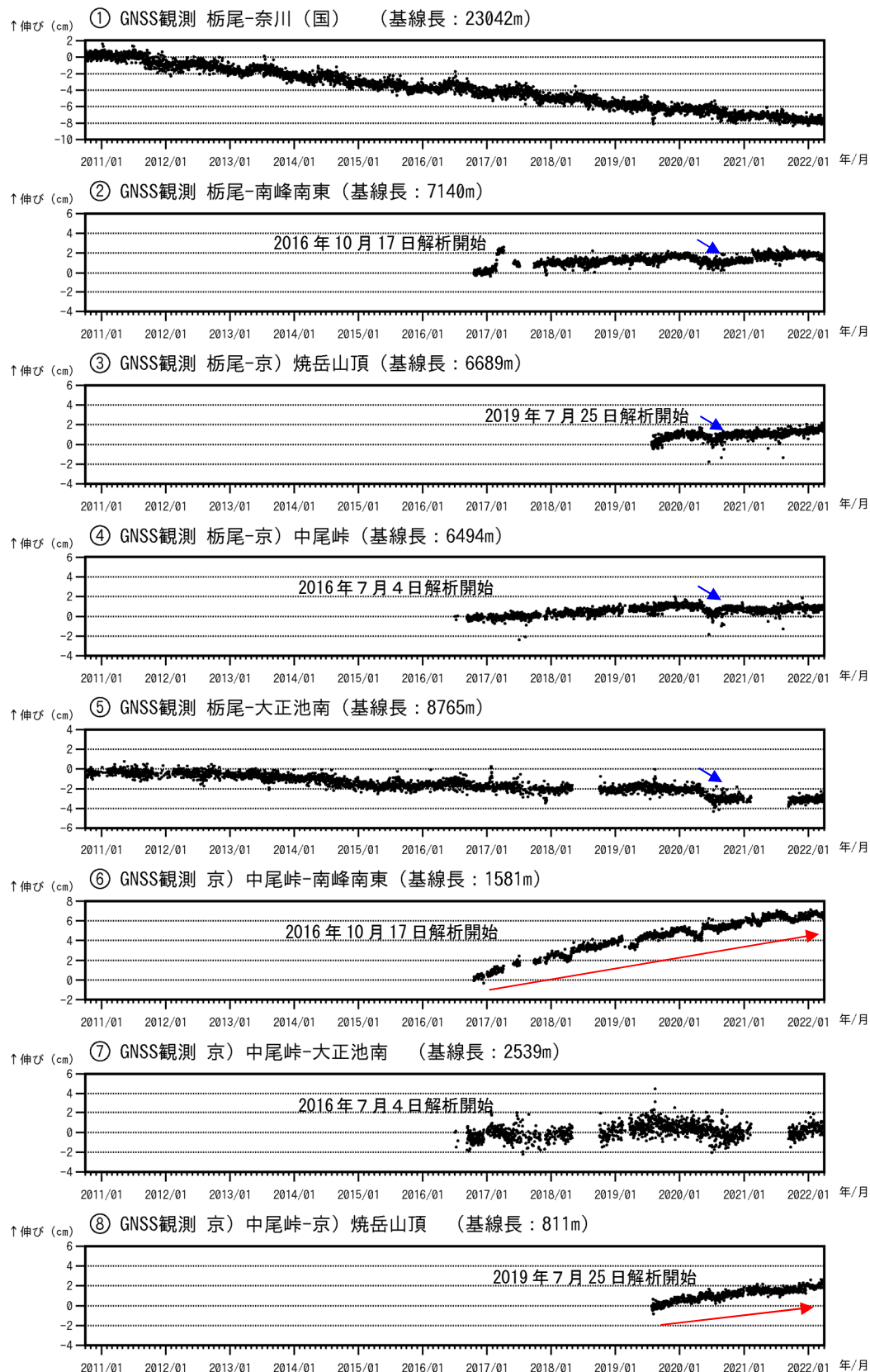
図5 焼岳 GNSS連続観測による基線長変化（2010年10月1日～2022年3月31日）
