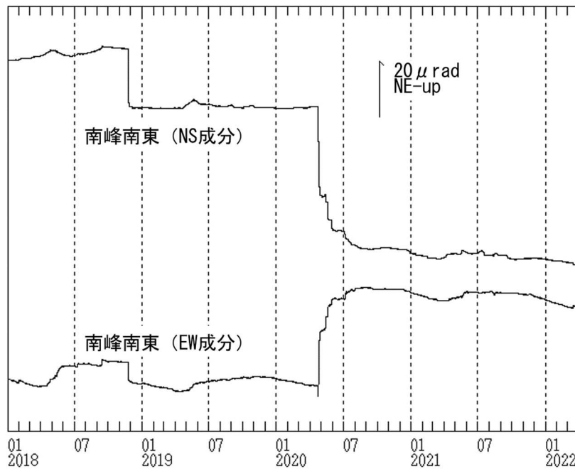
図7 焼岳 南峰南東観測点における傾斜データ（2018年1月1日～2022年3月31日）
