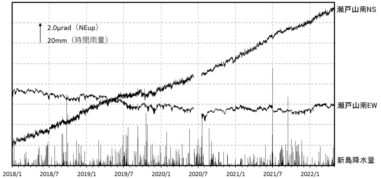
図4 新島 瀬戸山南観測点の傾斜変動（2018年1月1日～2022年4月30日）
