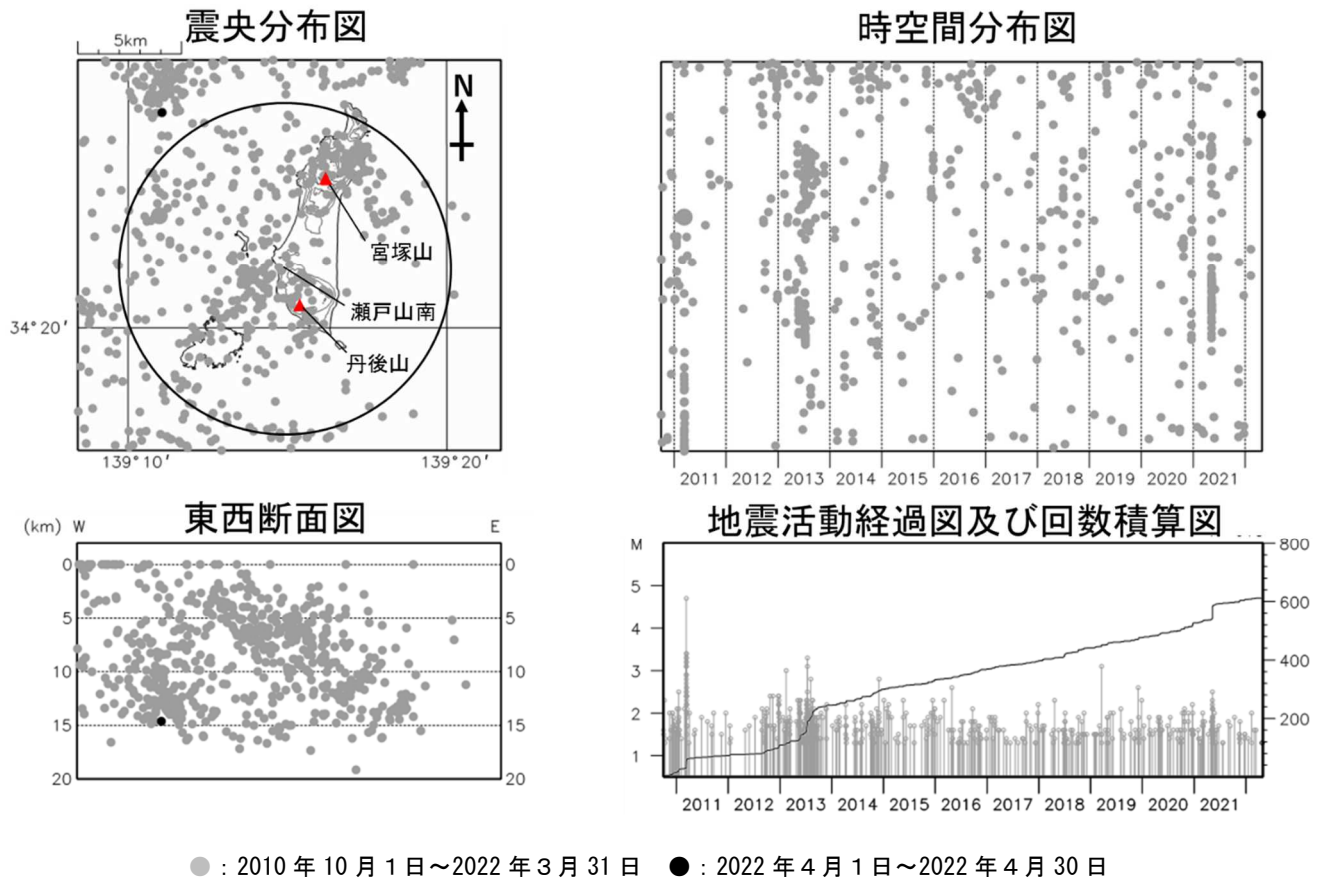
図3 新島 広域地震観測網による山体・周辺の地震活動（2010年10月1日～2022年4月30日） 広域地震観測網により震源決定したもので、深さは全て海面以下として決定しています。 M（マグニチュード）は地震の規模を表し、M1.3以上の地震を示しています。 図中の震源要素は一部暫定値が含まれており、後日変更することがあります。 計数対象（瀬戸山南から半径約8km、深さ約20km以内）以外の地震が含まれるため、図2-①の日別A型地震回数とは異なります。 震央分布図中の円は火山性地震の回数の計数対象（瀬戸山南から半径8km、深さ20km以内）の範囲を示しています。 この図では、関係機関の地震波形を一元的に処理し、地震観測点の標高を考慮する等した手法で得られた震源を用いています（ただし、2020年8月以前の地震については火山活動評価のための参考震源です）。
