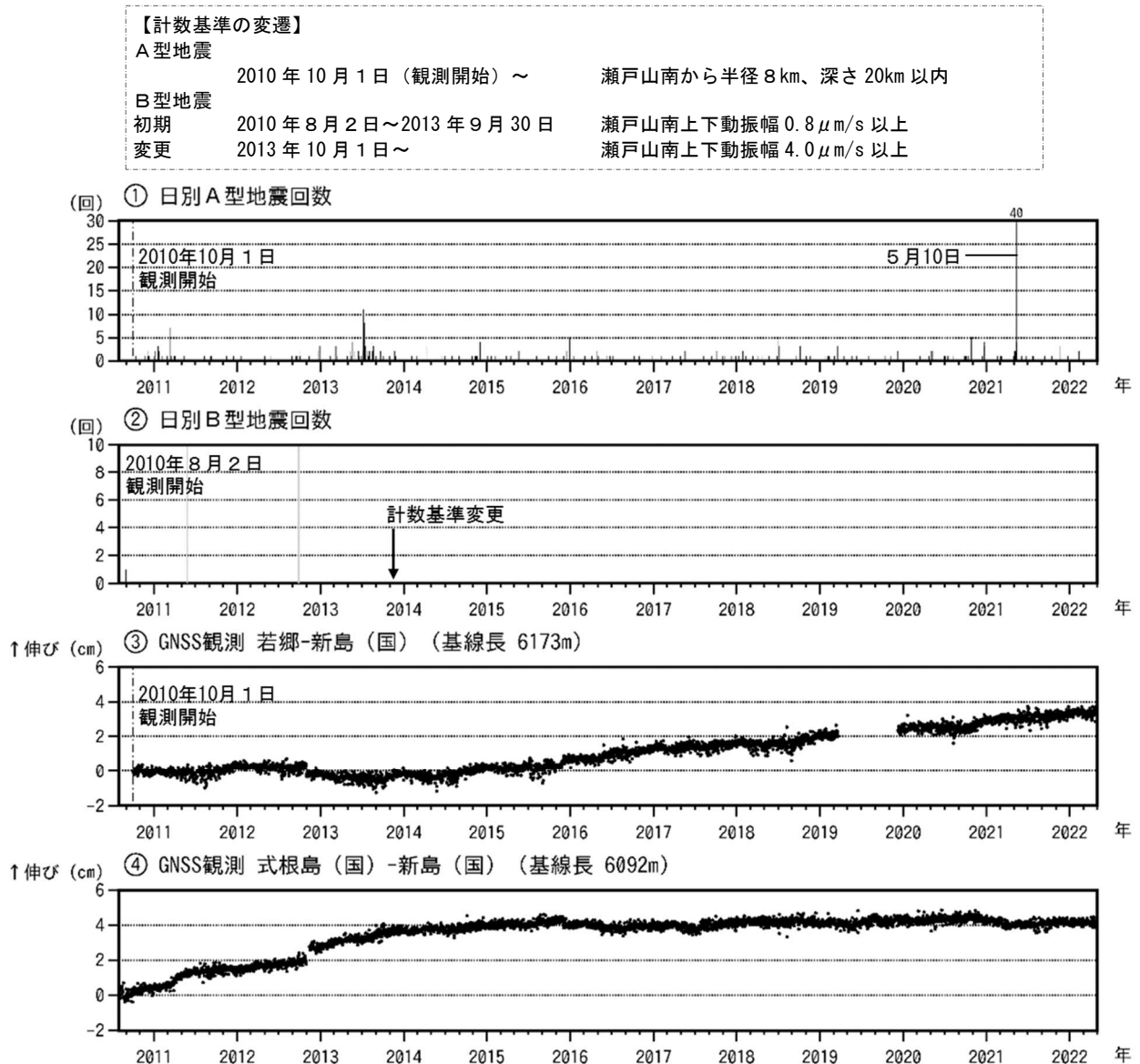
図2 新島 火山活動経過図(2010年8月2日～2022年4月30日)
