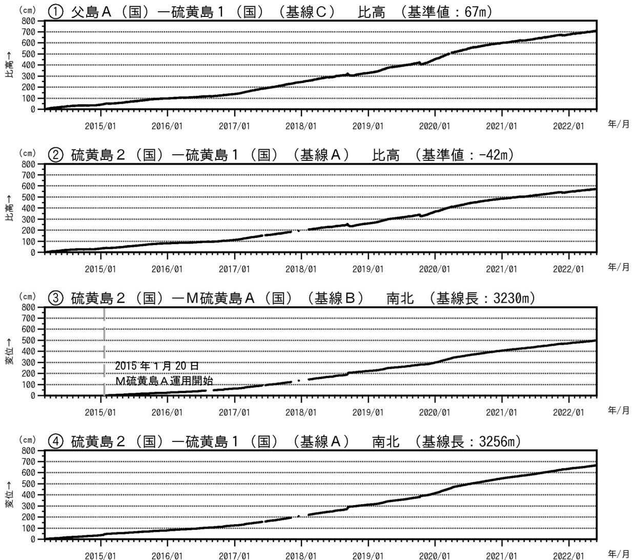
図5 硫黄島 GNSS 連続観測結果 (2014年3月1日~2022年5月31日)
