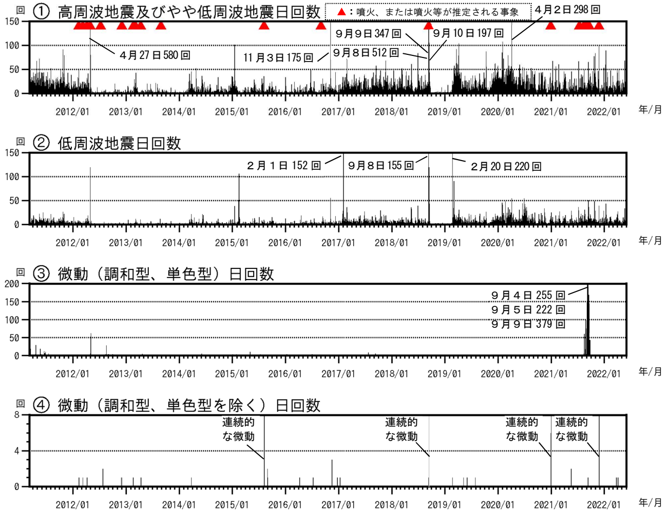
図4 硫黄島 長期火山活動経過図（2011年3月8日～2022年5月31日）
