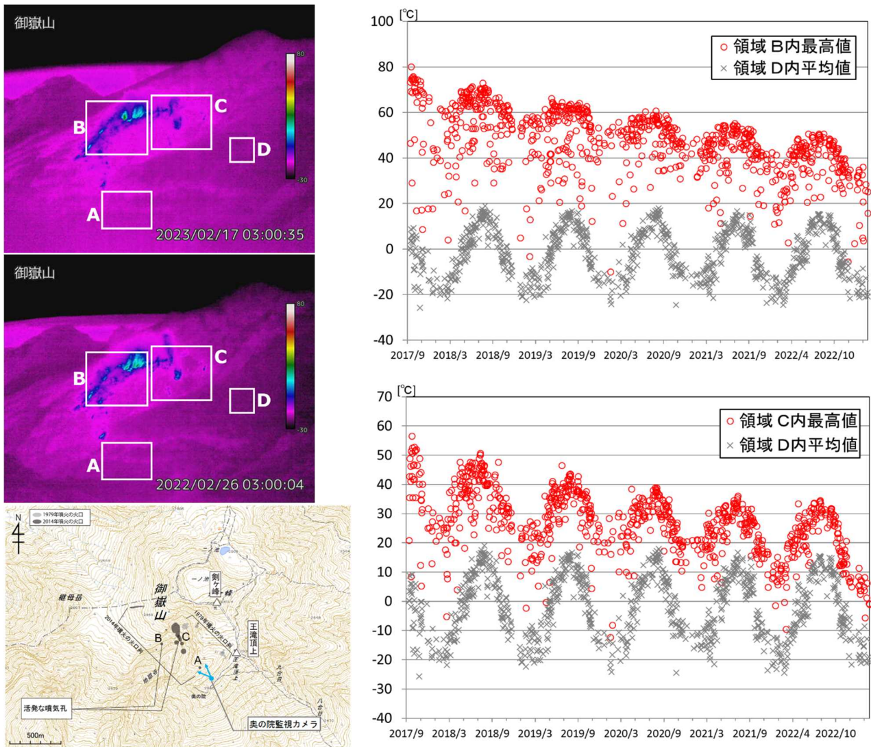
図6 御嶽山 奥の院赤外熱映像カメラによる剣ヶ峰南西側における最高温度の推移 (2017年9月13日～2023年2月28日)
