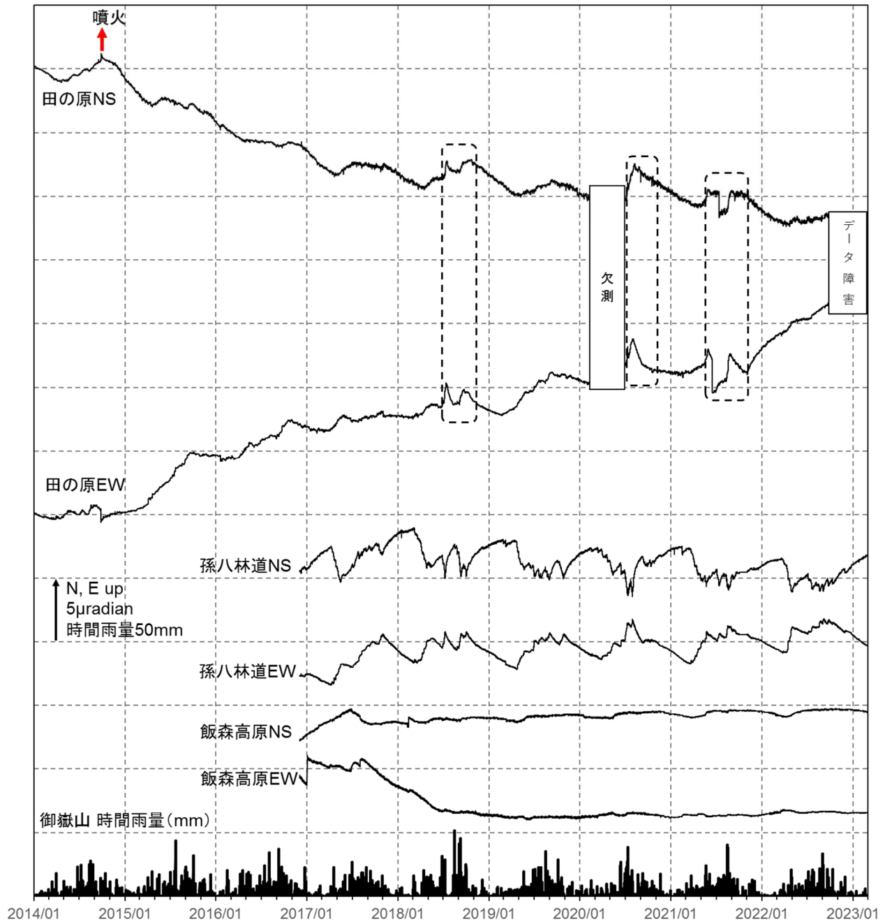
図4 御嶽山 傾斜変動（2014年1月1日～2023年2月28日）
