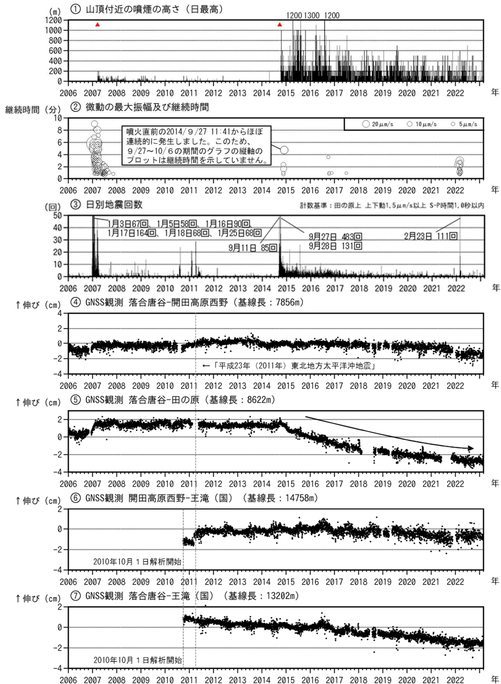
図1 御嶽山 長期間の火山活動経過図（2006年1月1日～2023年2月28日）
