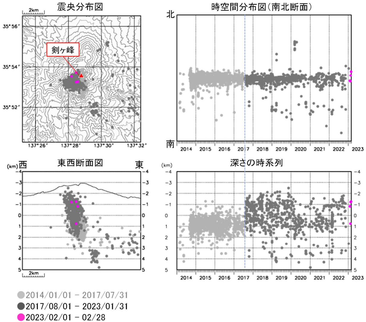
図2 御嶽山 震源分布図（2014年1月1日～2023年2月28日）
