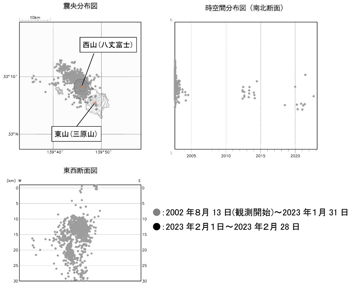
図3 八丈島 震源分布図（2002 年8 月 13 日～2023 年2 月 28 日）
