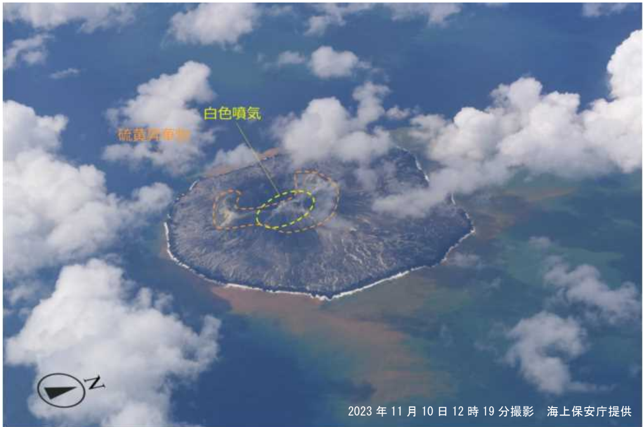
図2 西之島 上空からの観測による西之島の状況（11月10日 海上保安庁による観測）
