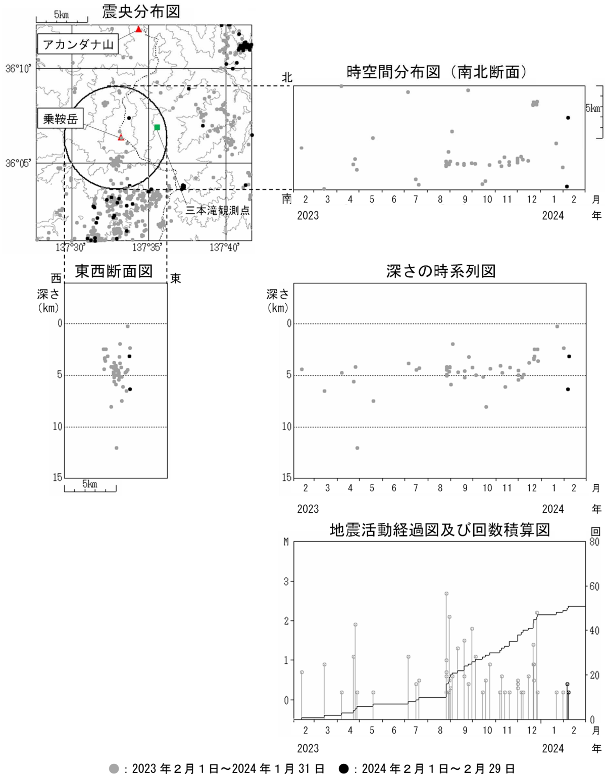
図3 乗鞍岳 広域地震観測網による山体・周辺の地震活動(2023年2月1日～2024年2月29日)
