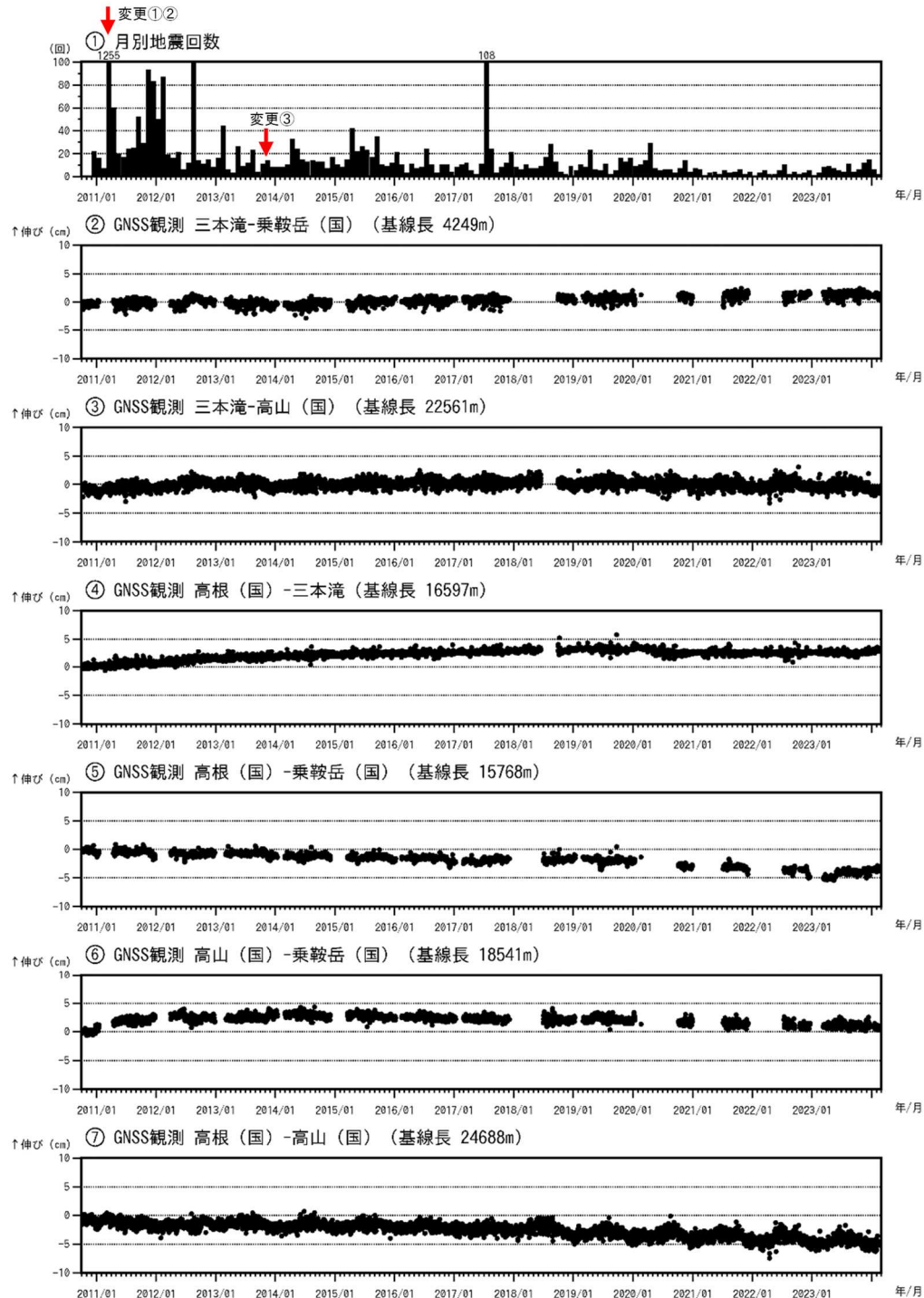
図2 乗鞍岳 火山活動経過図（2010年10月1日～2024年2月29日）
