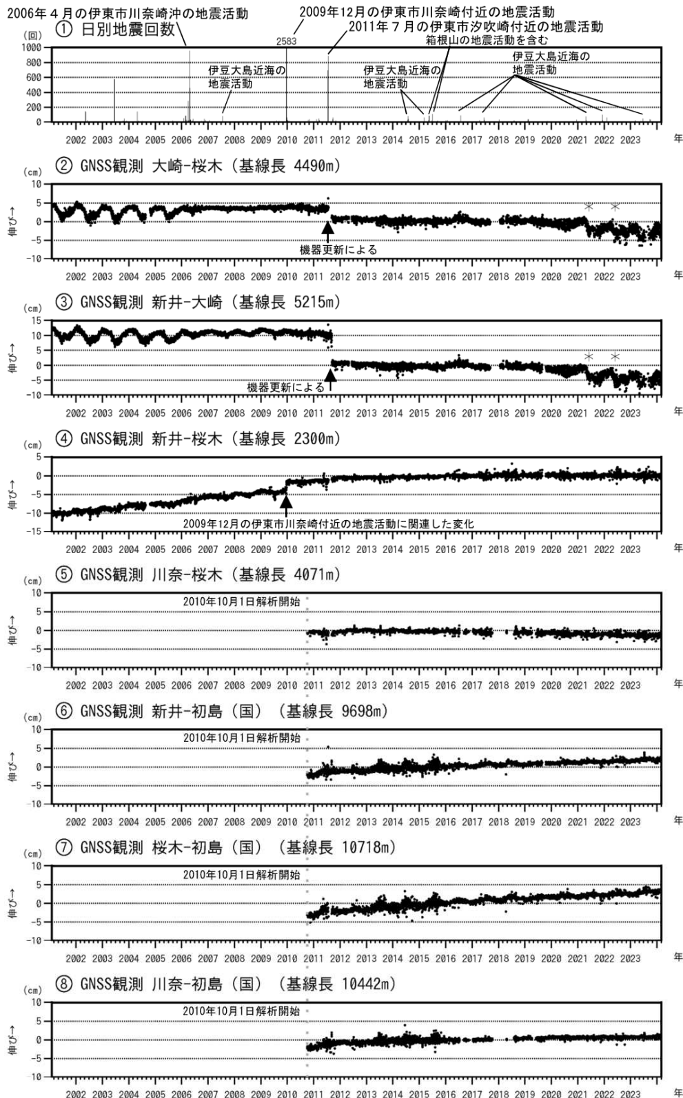
図3 伊豆東部火山群 火山活動経過図（2001年2月1日～2024年2月29日）
