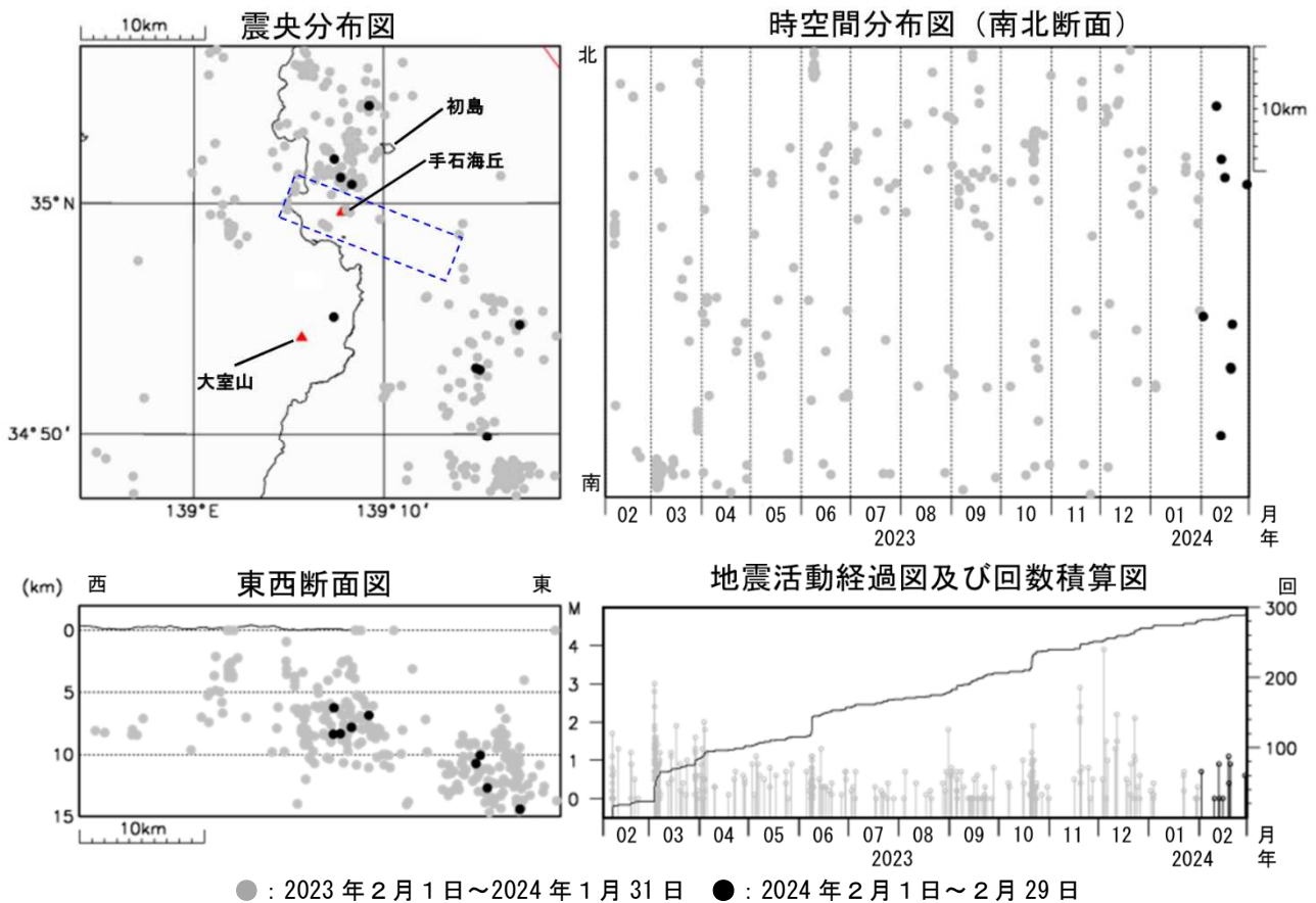
図2 伊豆東部火山群 広域地震観測網による震源分布図（2023 年 2 月 1 日～2024 年 2 月 29 日） □ の領域は群発地震活動の発生する可能性がある範囲（火口が出現する可能性のある範囲）を示しています。 https://www.data.jma.go.jp/vois/data/tokyo/STOCK/level/PDF/level_316.pdf 広域地震観測網により震源決定したもので、深さは全て海面以下として決定しています。 M（マグニチュード）は地震の規模を表し、M0.0 以上を表示しています。 図中の震源要素は一部暫定値が含まれており、後日変更することがあります。 この図では、関係機関の地震波形を一元的に処理し、地震観測点の標高を考慮する等した手法で得られた震源を用いています。
