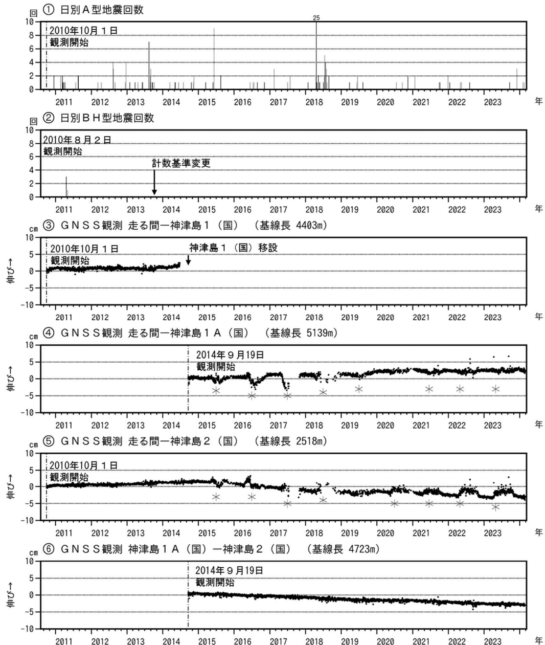
図2 神津島 火山活動経過図(2010年8月2日～2024年2月29日)
