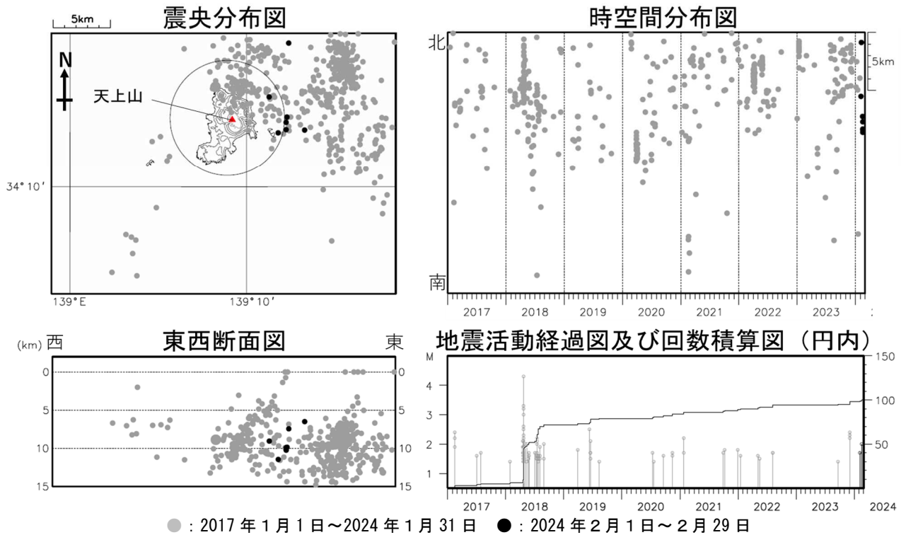
図3 神津島 広域地震観測網による山体・周辺の地震活動（2017年1月1日～2024年2月29日）
