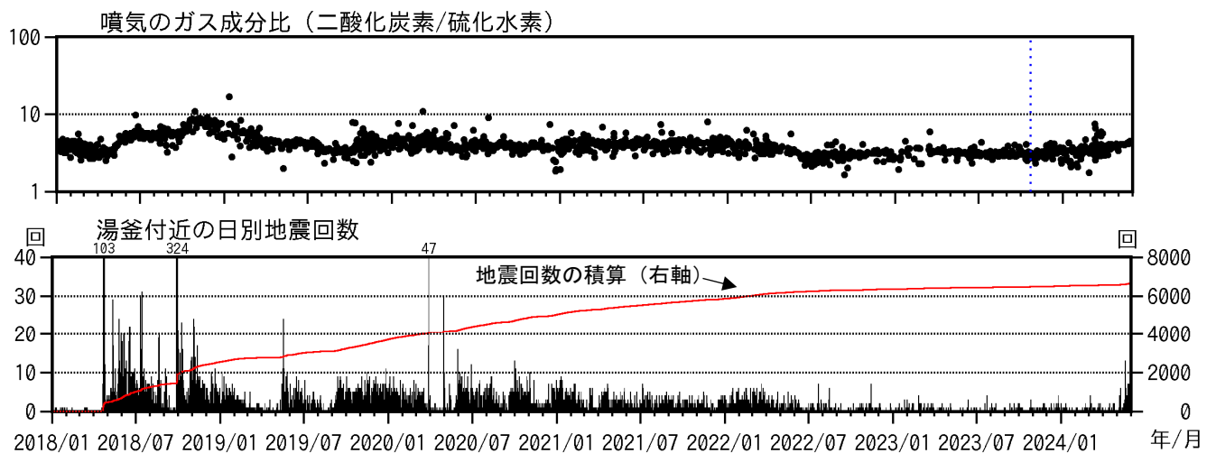
図8 草津白根山（白根山（湯釜付近）） 火山ガス観測結果（2018年1月～2024年5月）
