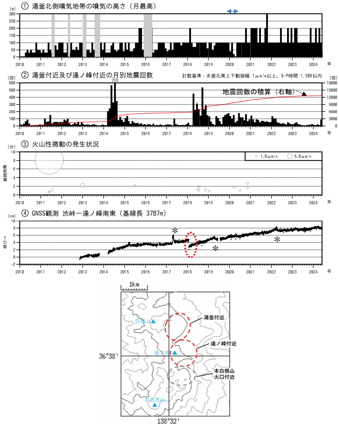
図3 草津白根山（白根山（湯釜付近）） 火山活動経過図（2010年1月1日～2024年5月31日）
