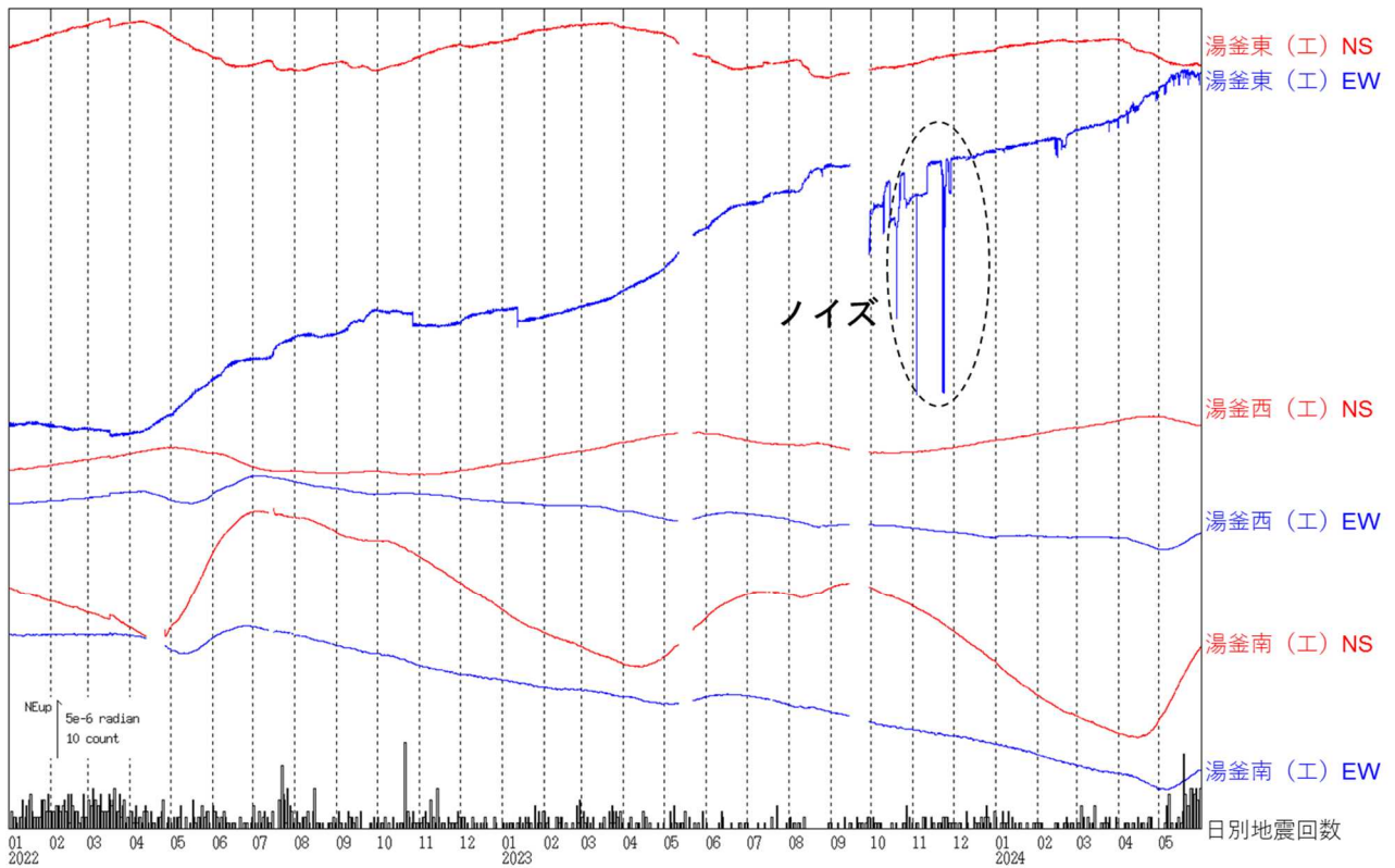
図5 草津白根山（白根山（湯釜付近）） 傾斜変動（2022年1月1日～2024年5月31日） （工）：東京工業大学
