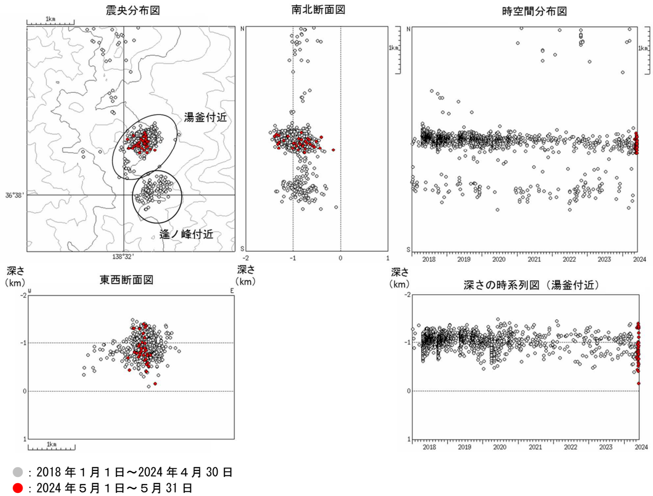
図4 草津白根山 震源分布図（2018 年 1 月 1 日～2024 年 5 月 31 日）
