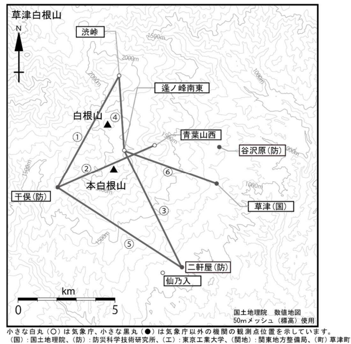
図7 草津白根山 GNSS 観測点配置図
