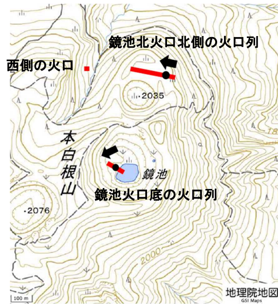
図 12－2 草津白根山（本白根山） 図 12－3 の撮影位置（黒丸）及び方向（矢印）。
