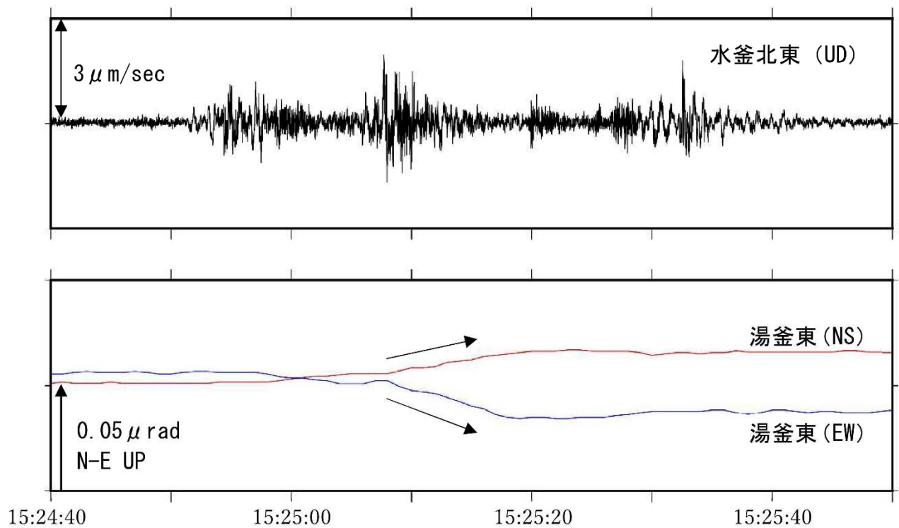
図 1-2 草津白根山（白根山（湯釜付近）） ごくわずかな傾斜変動を伴う低周波地震
