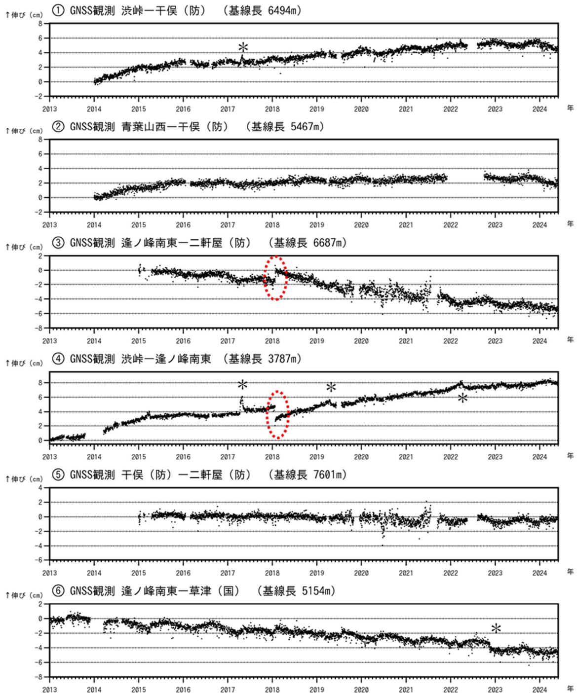
図6 草津白根山 GNSS 連続観測の結果（2013 年 1 月 1 日～2024 年 5 月 31 日）
