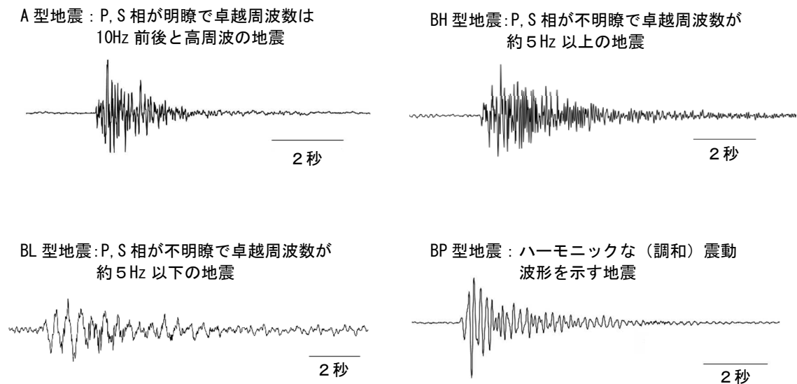
図 1-3 草津白根山（白根山（湯釜付近）） 主な火山性地震の特徴と波形例
