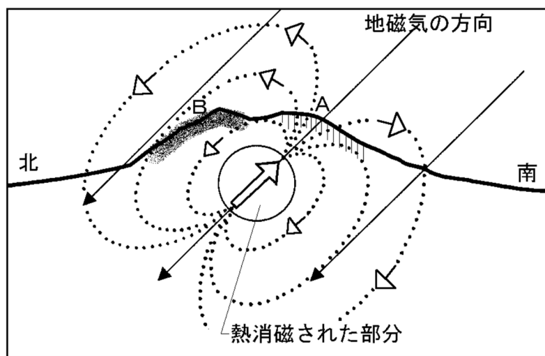
図 11 熱消磁に伴う全磁力変化のモデル
