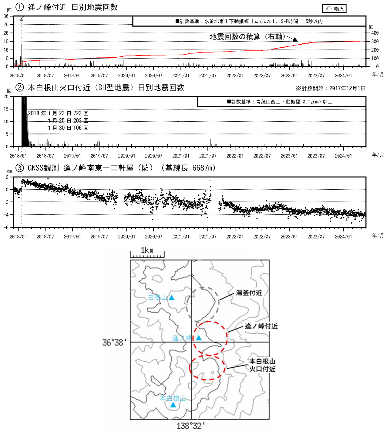
図13 草津白根山（本白根山） 火山活動経過図（2017年12月1日～2024年5月31日）
