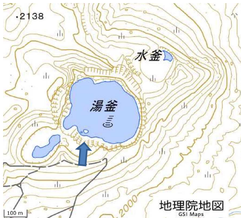
図2-2 草津白根山（白根山（湯釜付近）図2-3及び2-4の撮影位置及び方向（矢印）。
