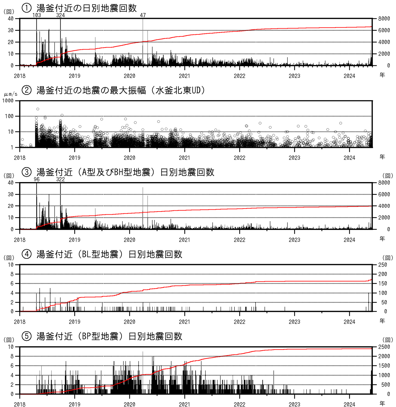
図1-1 草津白根山（白根山（湯釜付近）） 湯釜付近の地震活動の状況
