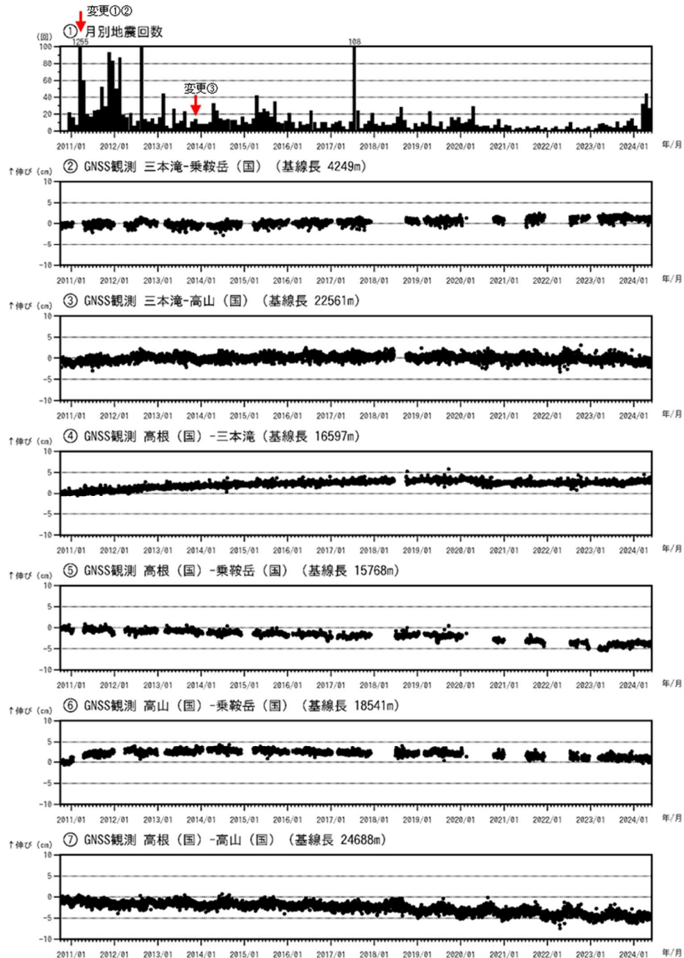
図2 乗鞍岳 火山活動経過図（2010年10月1日～2024年5月31日）
