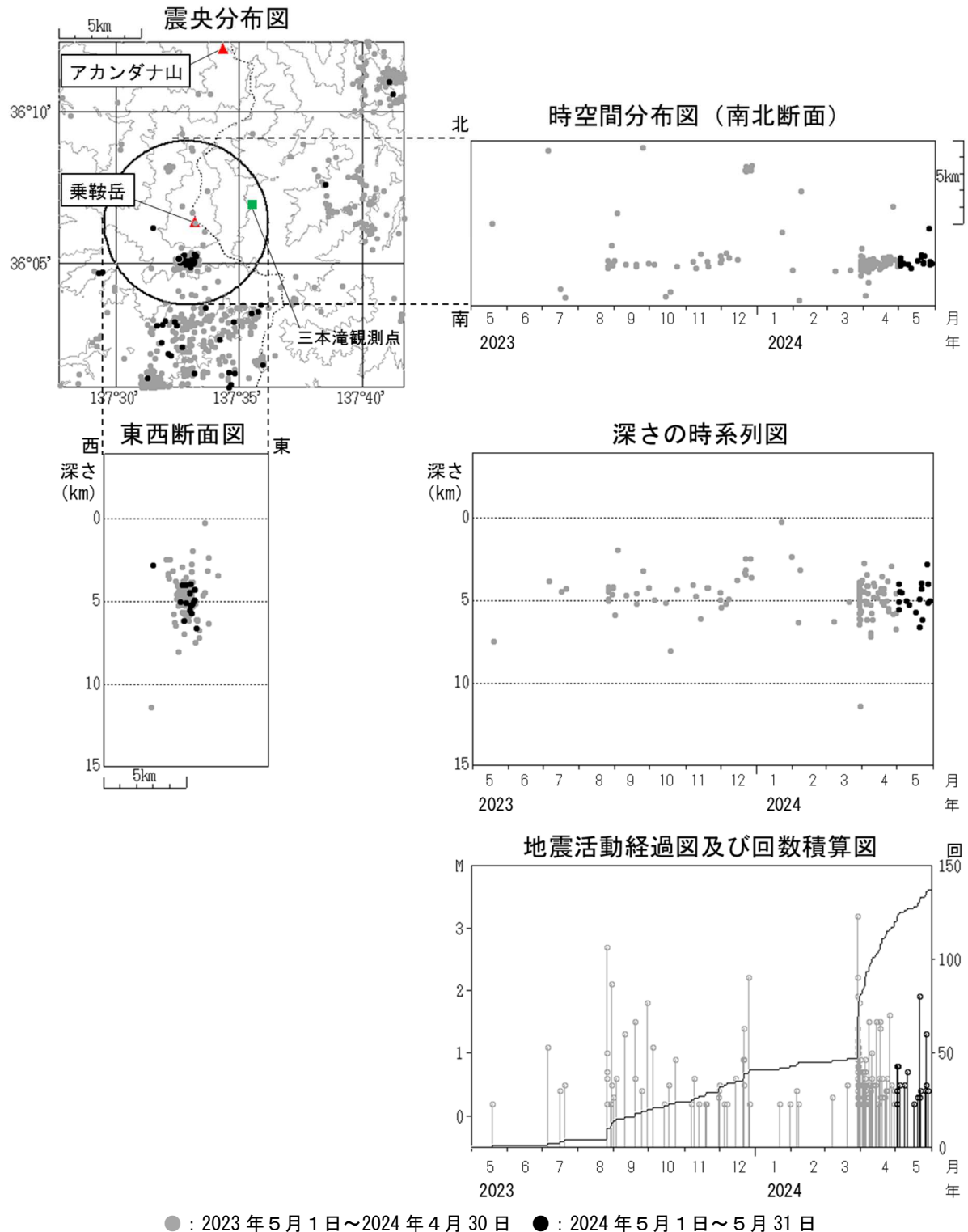
図3 乗鞍岳 広域地震観測網による山体・周辺の地震活動(2023年5月1日～2024年5月31日)
