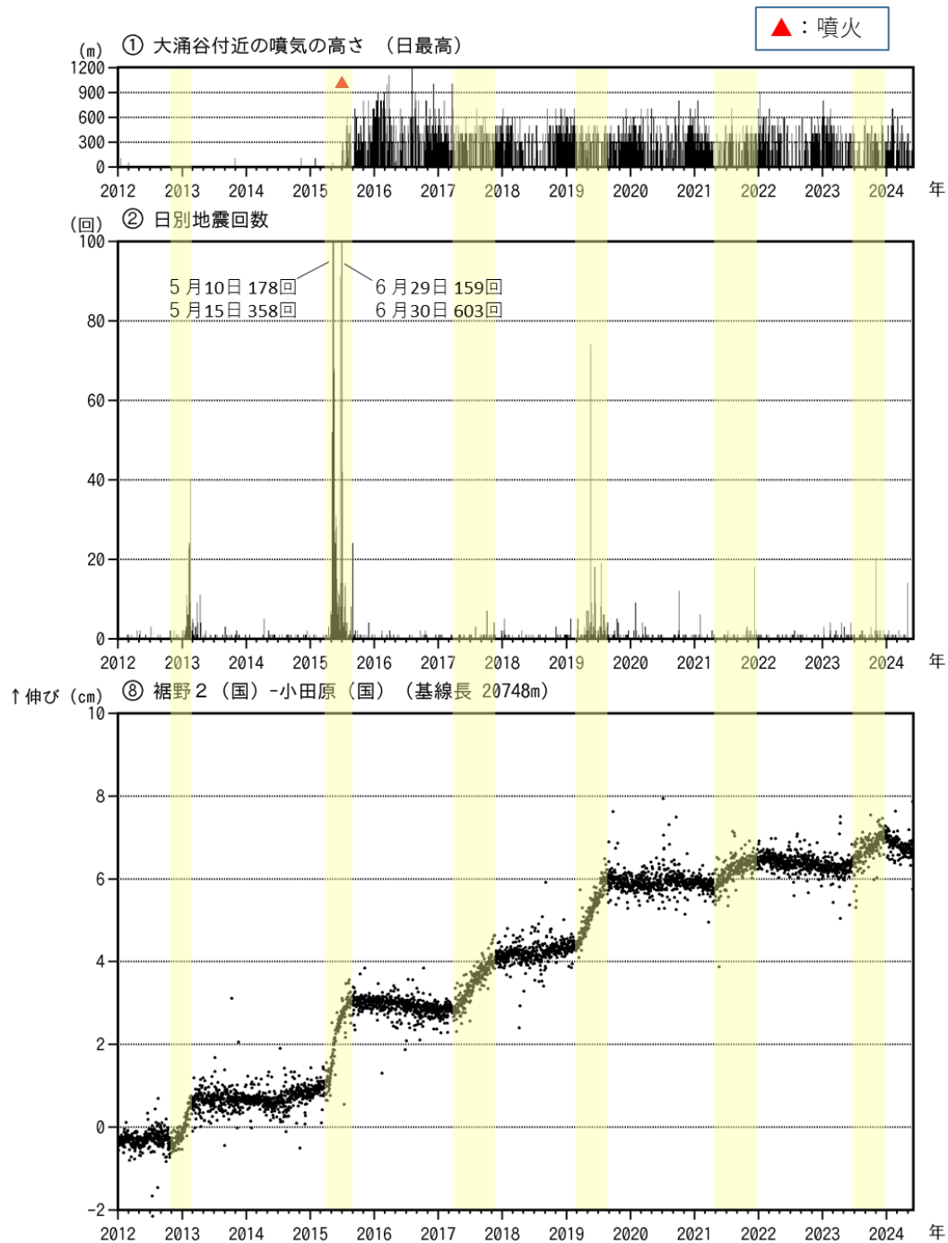
図3-1 箱根山 火山活動経過図（2012年1月1日～2024年5月31日）
