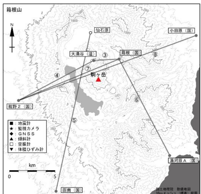
図3-2 箱根山 GNSS 連続観測による基線長変化及び観測点配置図 (2012年1月1日～2024年5月31日) (国): 国土地理院 (温): 神奈川県温泉地学研究所 空白部分は欠測を示します。
