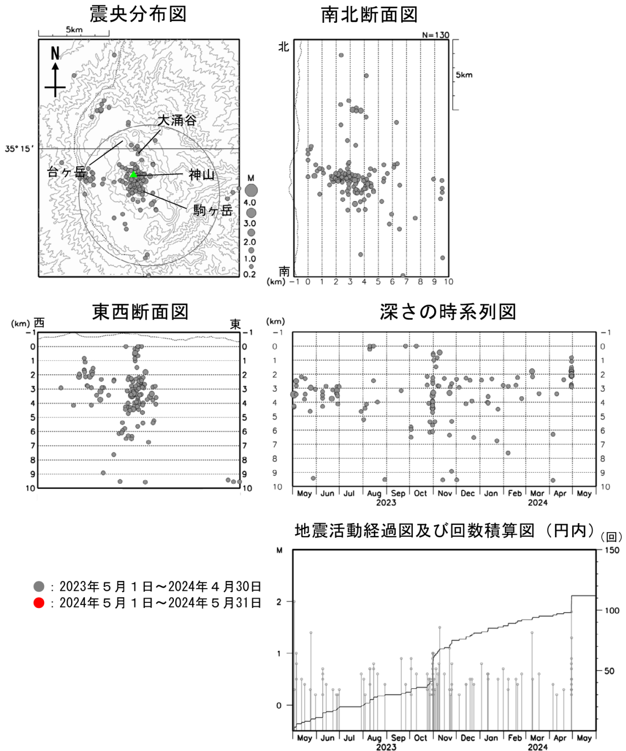
図4 箱根山 広域地震観測網による山体周辺の震源分布図（2023年5月1日～2024年5月31日）
