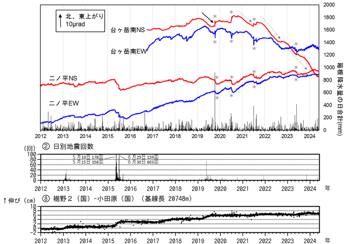
図5 箱根山 傾斜観測及び地震回数・GNSS観測（2012年1月1日～2024年5月31日）
