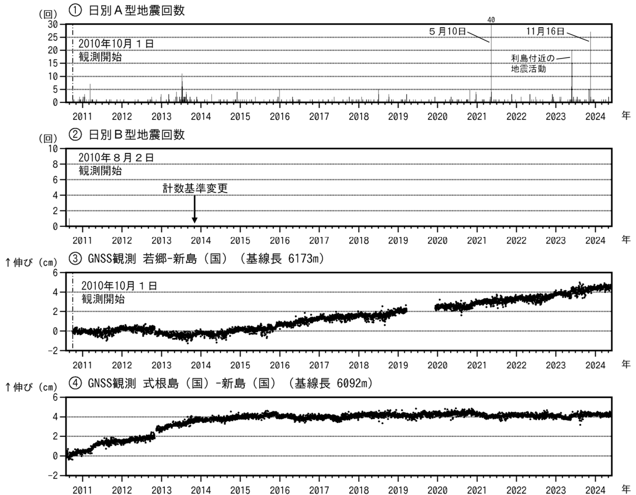
図2 新島 火山活動経過図(2010年8月2日～2024年5月31日) 、 のグラフは図4のGNSS基線、 に対応しています。また、グラフの空白部分は欠測を示しています。
