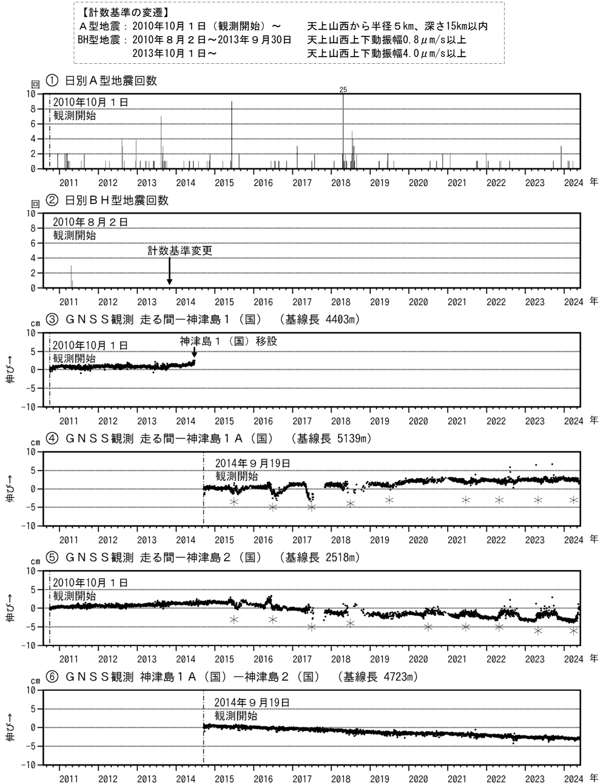
図2 神津島 火山活動経過図(2010年8月2日～2024年5月31日)
