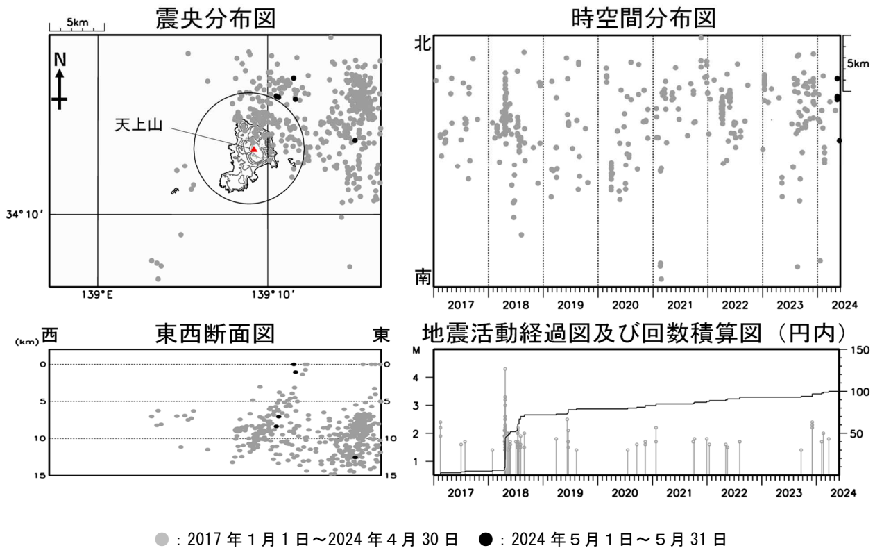
図3 神津島 広域地震観測網による山体・周辺の地震活動（2017年1月1日～2024年5月31日） 広域地震観測網により震源決定したもので、深さは全て海面以下として決定しています。 M（マグニチュード）は地震の規模を表し、M1.4以上の地震を示しています。 図中の震源要素は一部暫定値が含まれており、後日変更することがあります。 計数対象（天上山西から半径約5km、深さ約15km以内）以外の地震が含まれるため、図2-①の日別A型地震回数とは異なります。 震央分布図中の円は火山性地震の回数の計数対象（天上山西から半径5km、深さ15km以内）の範囲を示しています。 この図では、関係機関の地震波形を一元的に処理し、地震観測点の標高を考慮する等した手法で得られた震源を用いています（ただし、2020年8月以前の地震については火山活動評価のための参考震源です）。
