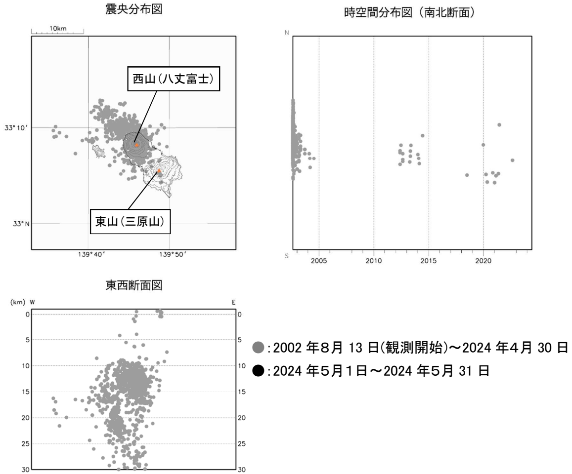
図3 八丈島 震源分布図（2002年8月13日～2024年5月31日）
