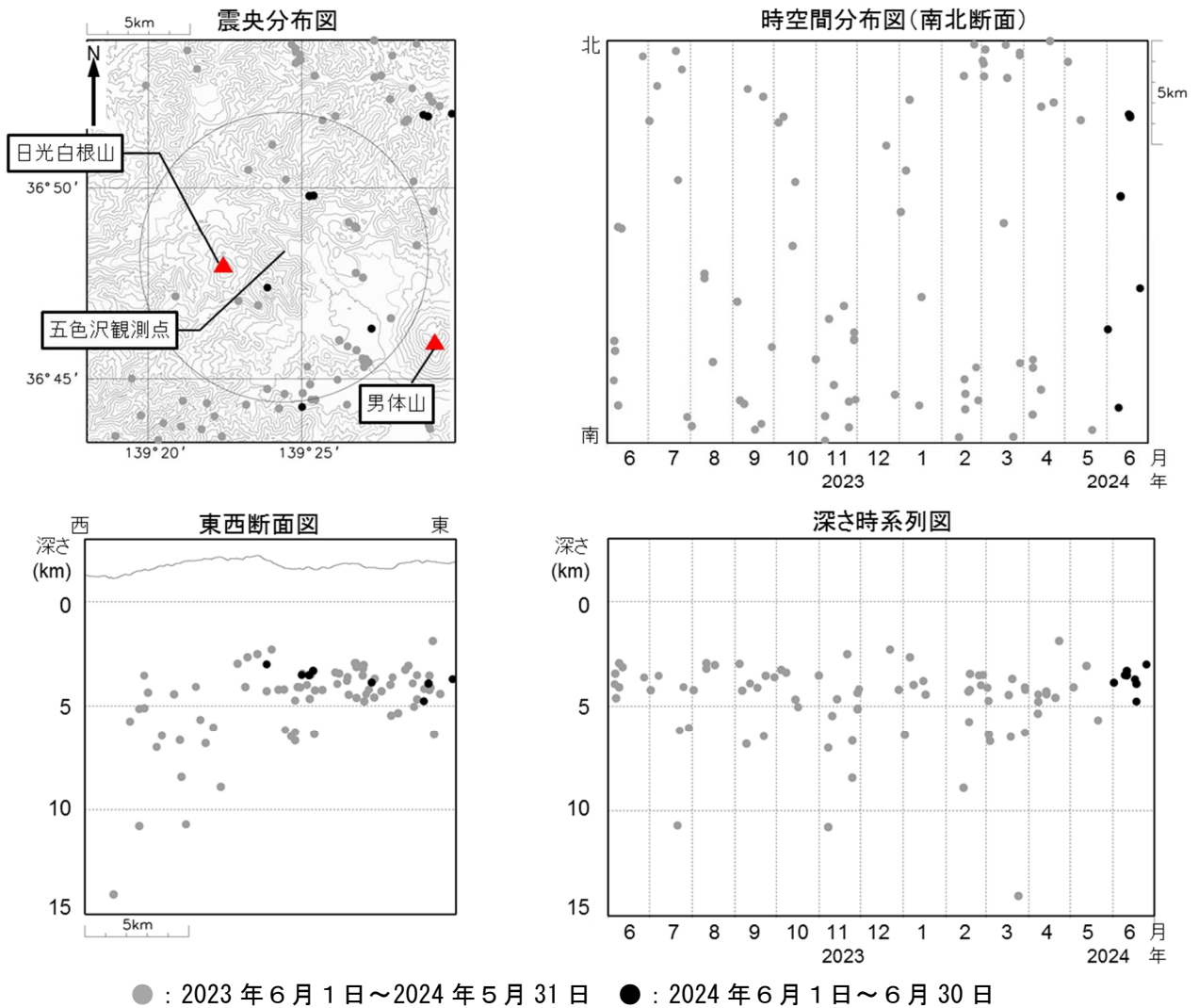
図3 日光白根山 広域地震観測網による山体周辺の地震活動 (2023 年 6 月 1 日～2024 年 6 月 30 日)
