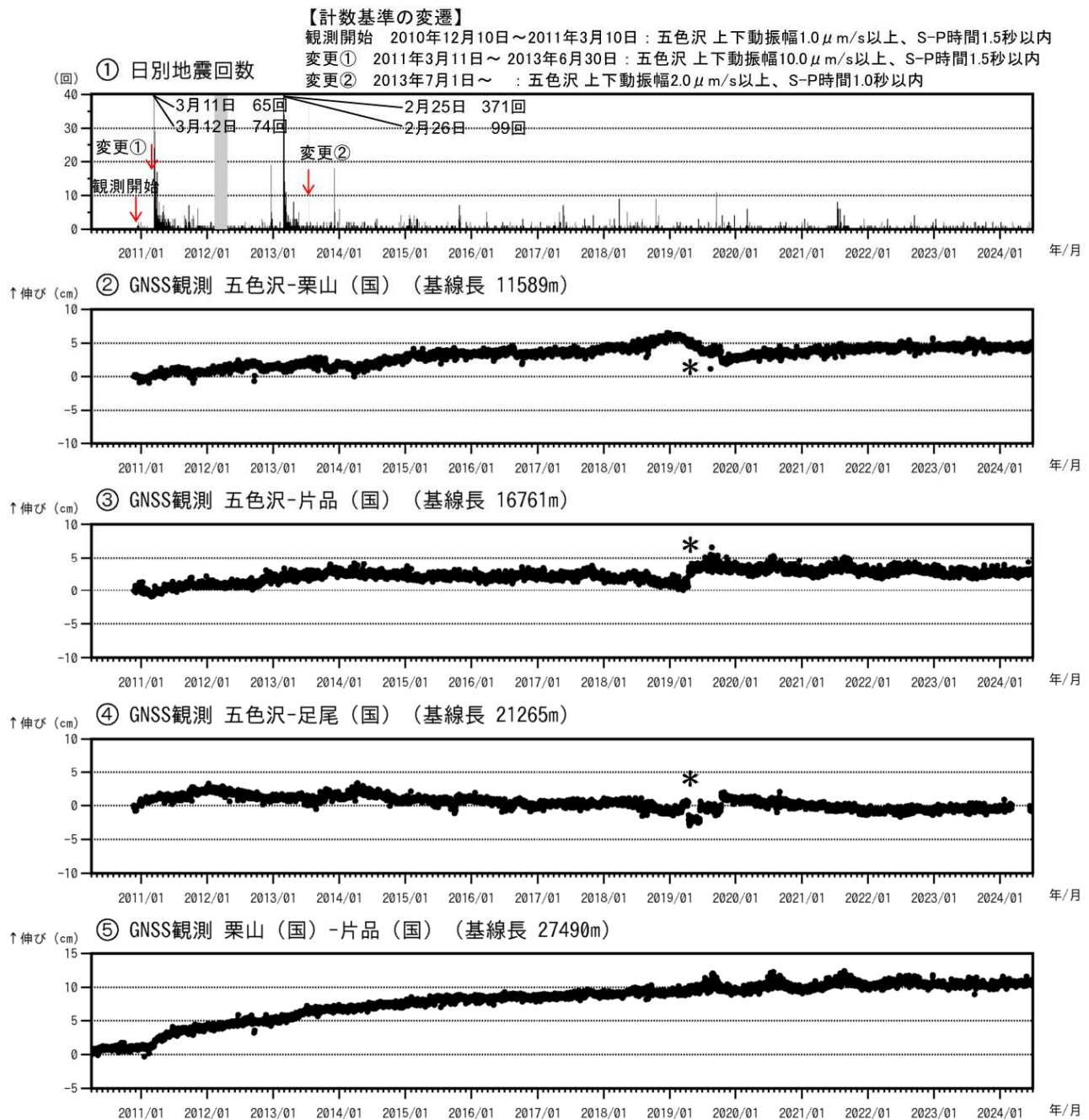
図2 日光白根山 火山活動経過図（2010年4月1日～2024年6月30日）
