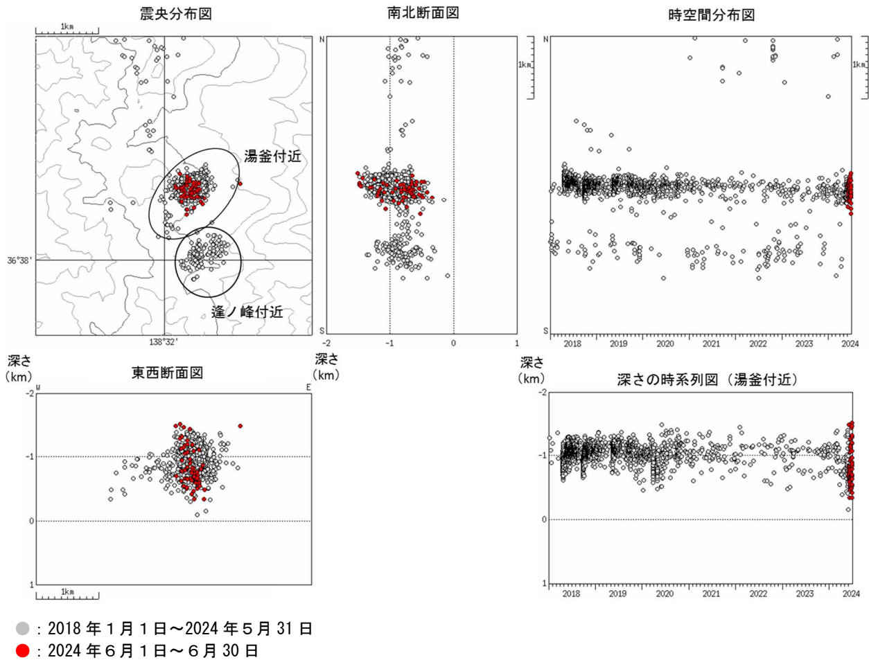
図4 草津白根山 震源分布図（2018 年 1 月 1 日～2024 年 6 月 30 日）
