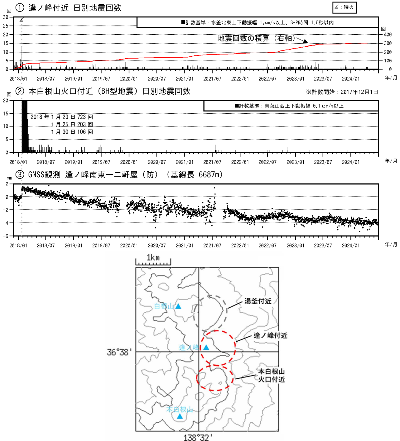
図13 草津白根山（本白根山） 火山活動経過図（2017年12月1日～2024年6月30日）
