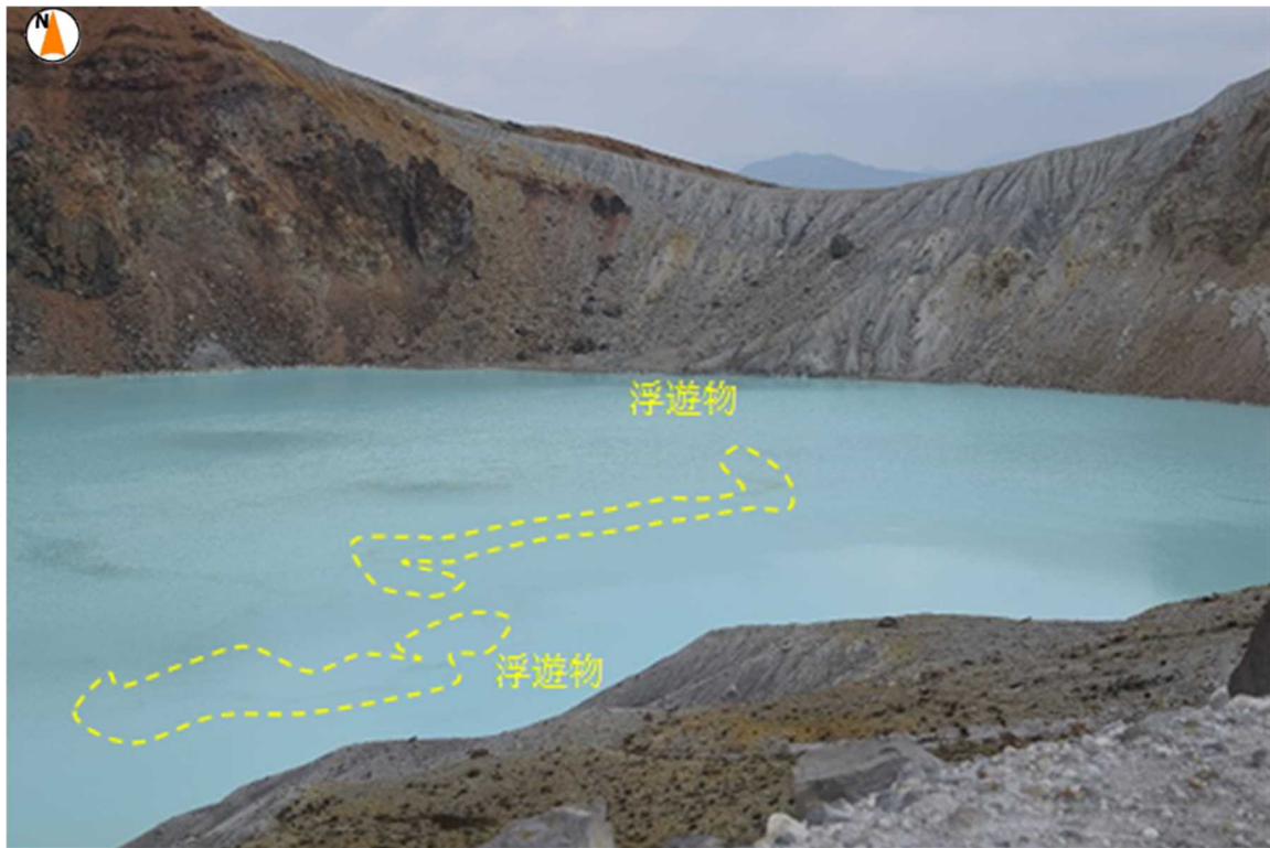
図2-3 草津白根山（白根山（湯釜付近））湯釜火口内の状況 ・20日に実施した現地調査観測では、湖面の南側から中央部にかけて浮遊物が認められました。
