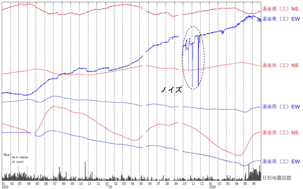
図5 草津白根山（白根山（湯釜付近）） 傾斜変動（2022年1月1日～2024年6月30日）
