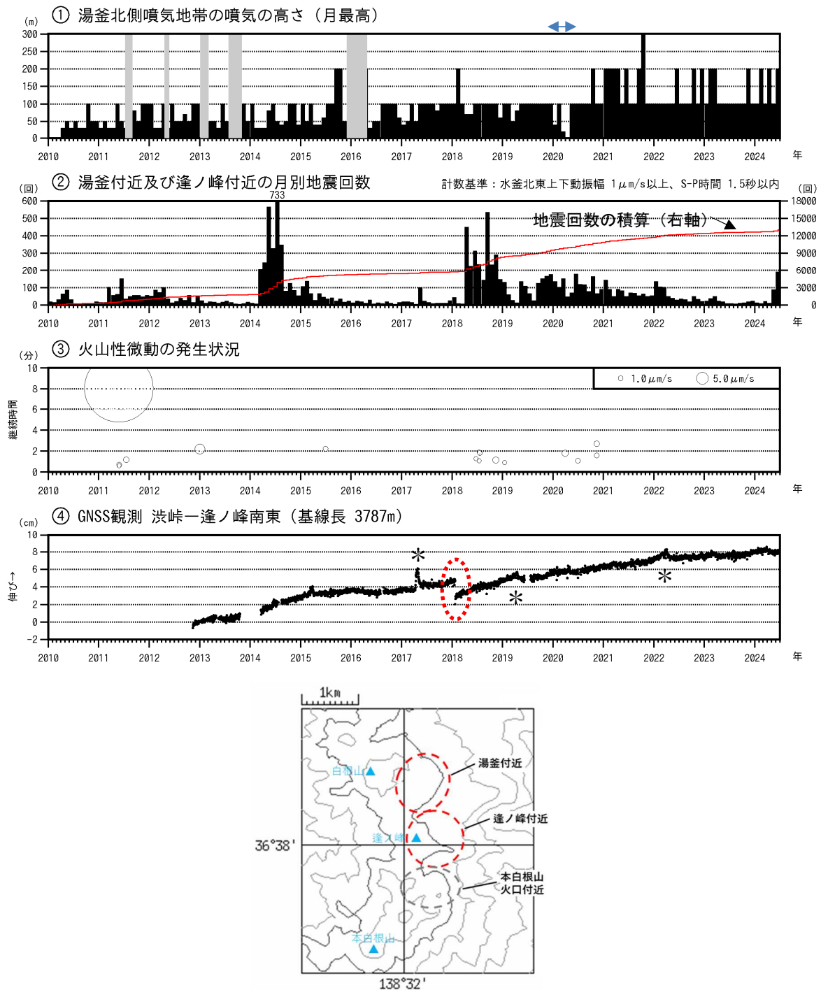
図3 草津白根山（白根山（湯釜付近）） 火山活動経過図（2010年1月1日～2024年6月30日）
