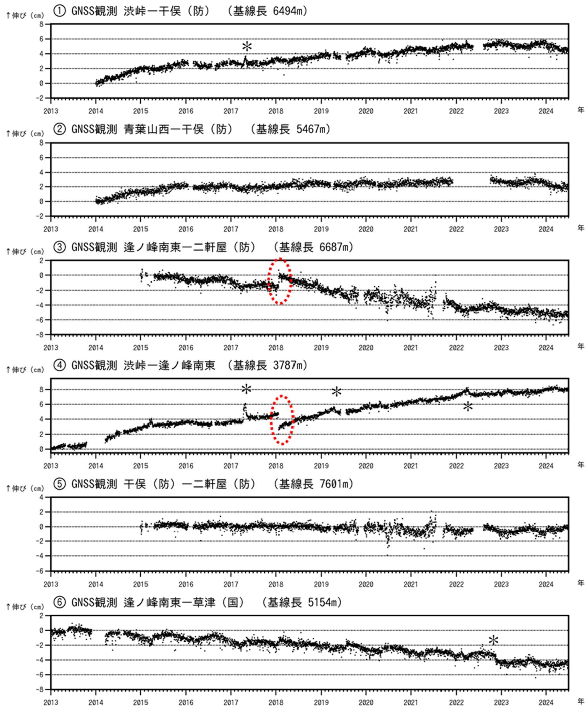
図6 草津白根山 GNSS 連続観測の結果（2013 年 1 月 1 日～2024 年 6 月 30 日）
