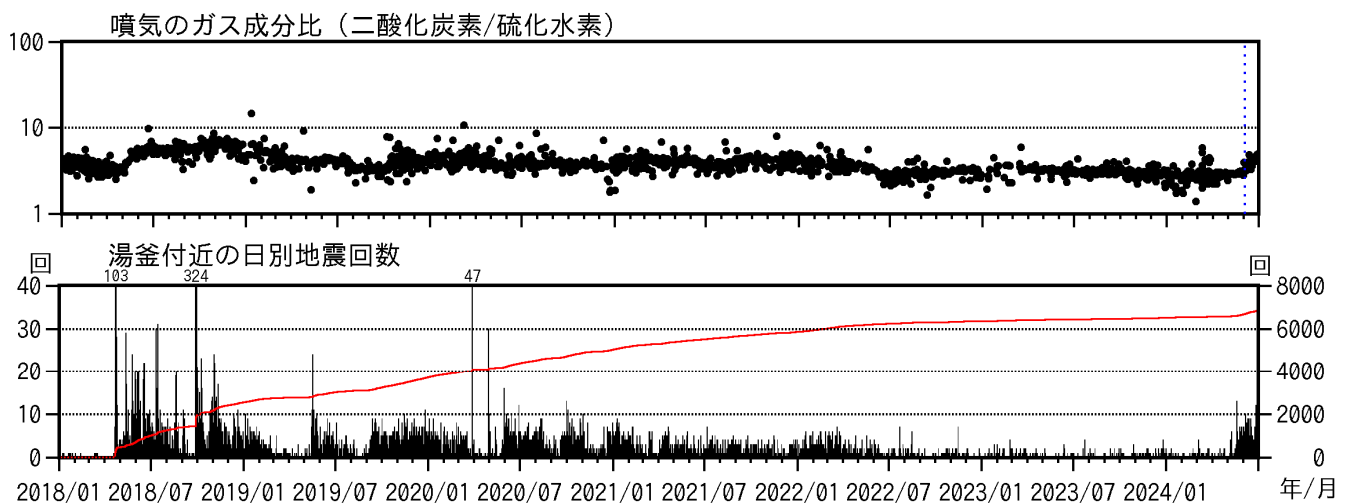
図8 草津白根山（白根山（湯釜付近）） 火山ガス観測結果（2018年1月～2024年6月）
