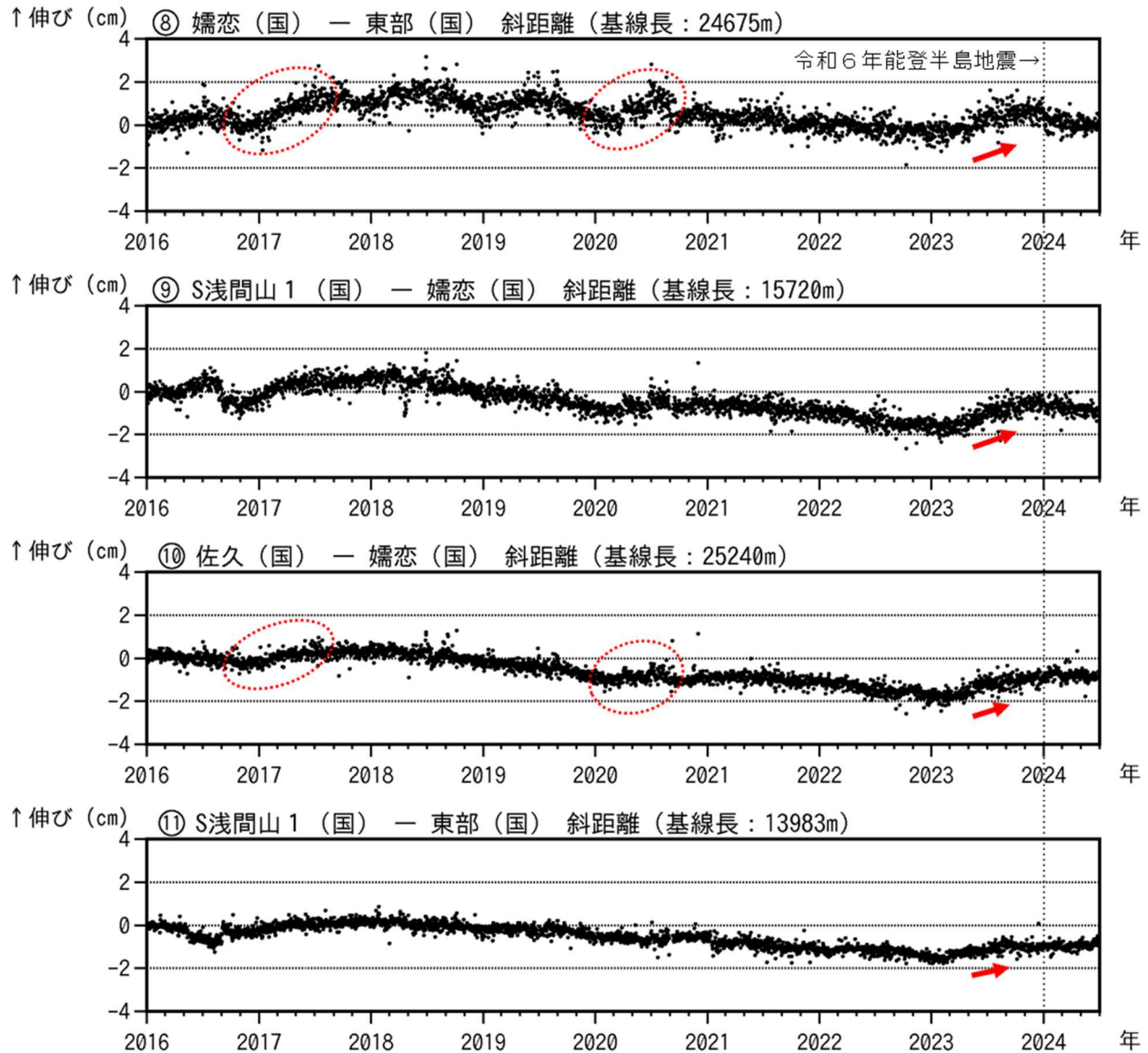
図7-2 浅間山 GNSS 連続観測結果(2016年1月1日～2024年6月30日)
