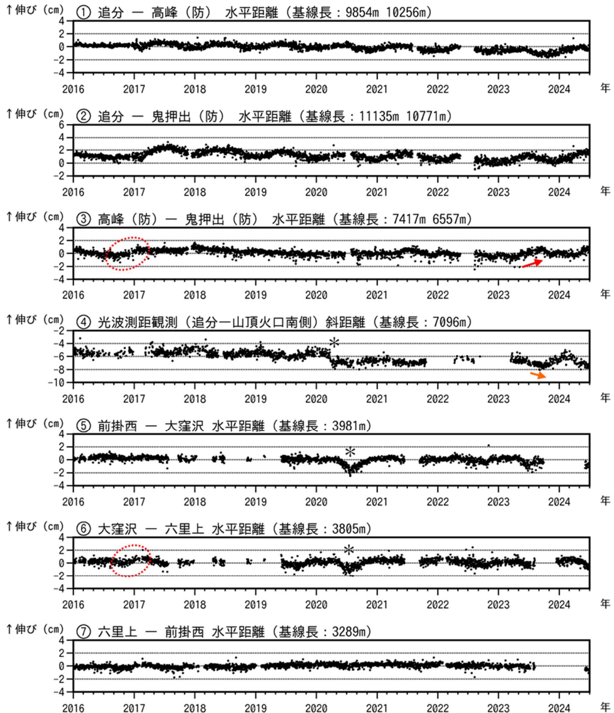
図7-1 浅間山 GNSS 連続観測及び光波測距観測結果(2016年1月1日~2024年6月30日)
