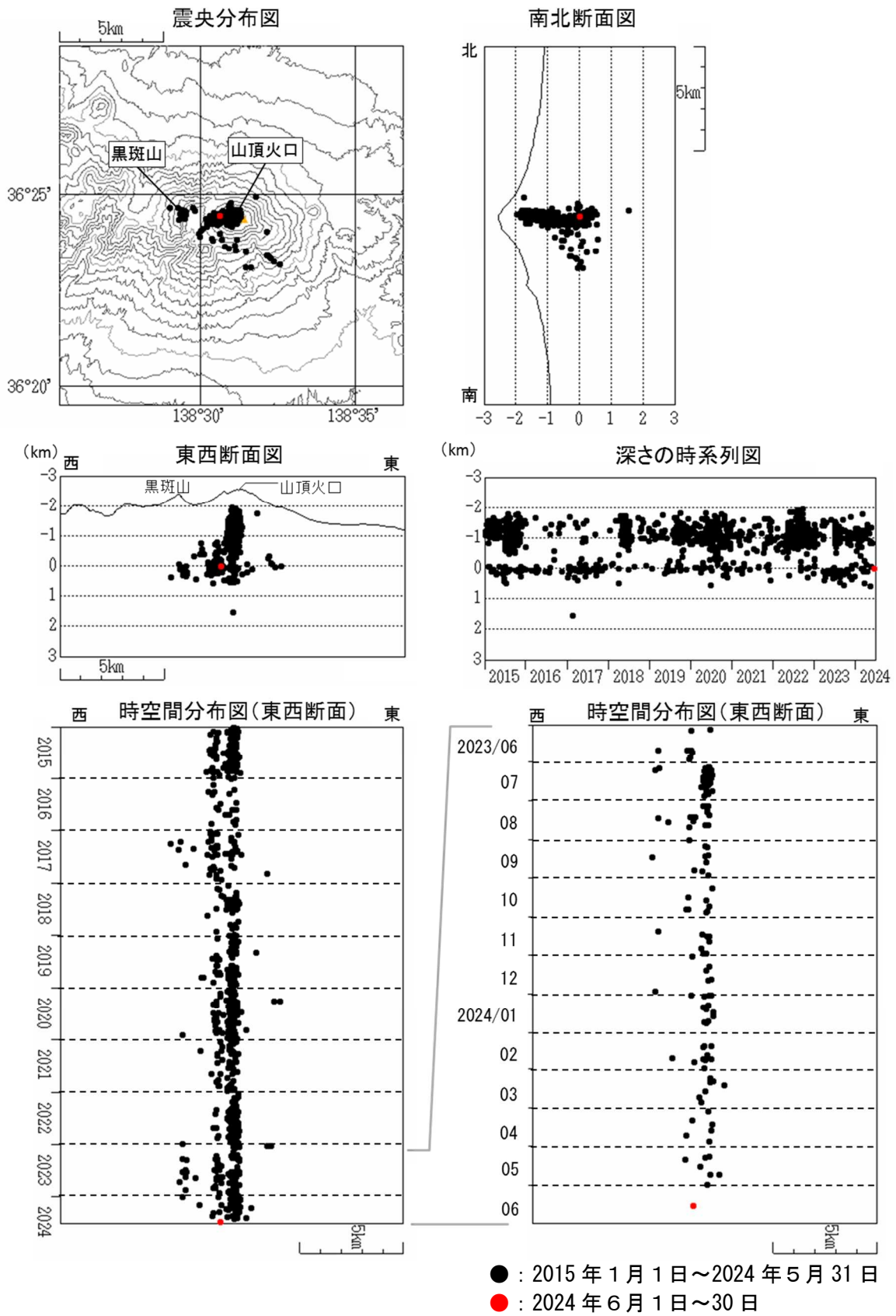
図5 浅間山 震源分布図（2015 年 1 月 1 日～2024 年 6 月 30 日）
