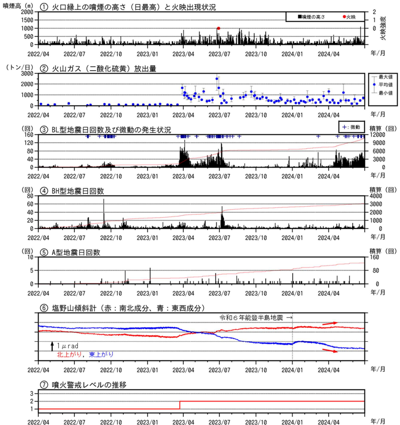
図2 浅間山 短期火山活動経過図（2022年4月1日～2024年6月30日）
