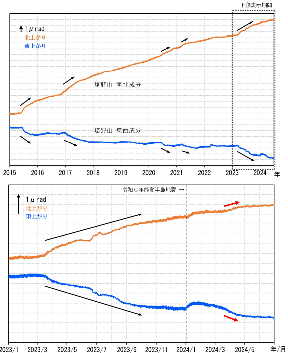
図6 浅間山 塩野山観測点における傾斜データ（2015年1月1日～2024年6月30日）
