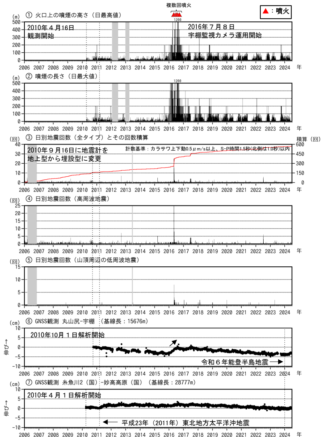
図2 新潟焼山 火山活動経過図（2006年1月1日～2024年6月30日）
