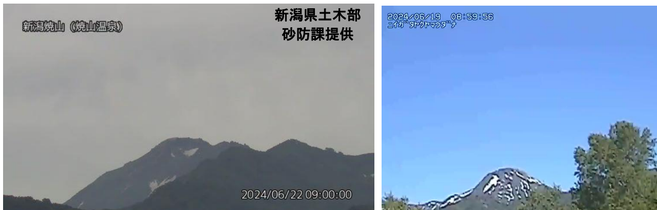
図1 新潟焼山 山頂部の噴煙の状況 （左：焼山温泉監視カメラ（6月22日）、右：宇棚監視カメラ（6月19日）による）
