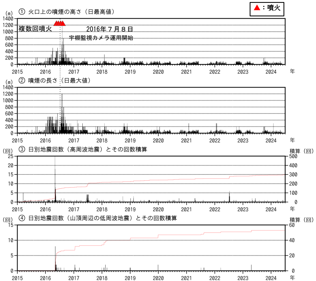
図3 新潟焼山 火山活動経過図（短期）（2015年1月1日～2024年6月30日）
