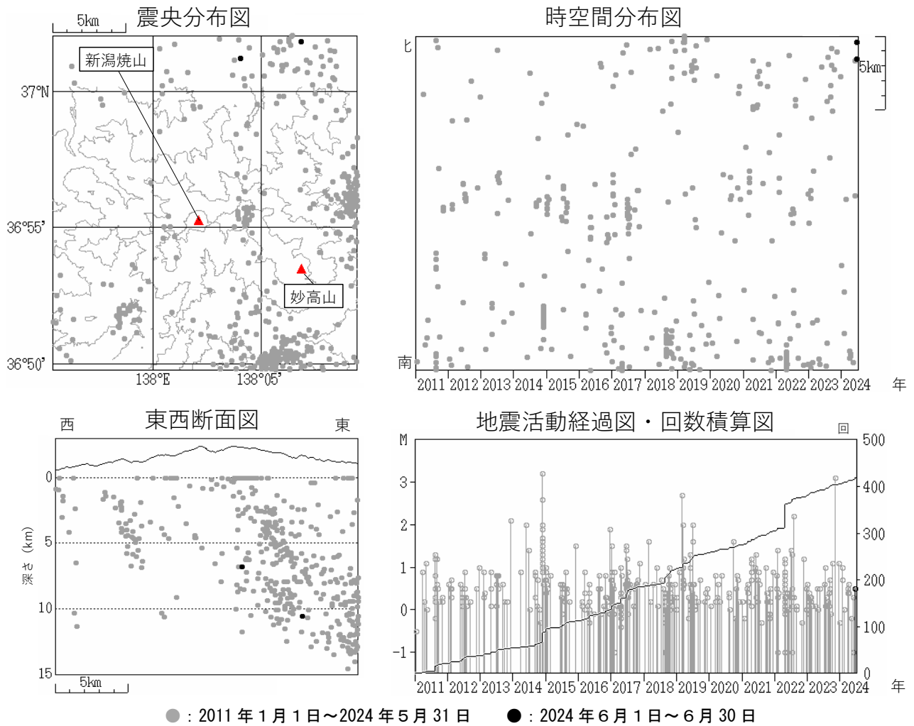
図4 新潟焼山 広域地震観測網による山体・周辺の地震活動（2011 年 1 月 1 日～2024 年 6 月 30 日）
