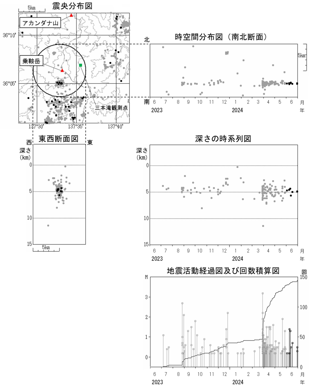
● : 2023 年 6 月 1 日～2024 年 5 月 31 日 ● : 2024 年 6 月 1 日～6 月 30 日 図3 乗鞍岳 広域地震観測網による山体・周辺の地震活動(2023 年 6 月 1 日～2024 年 6 月 30 日)
