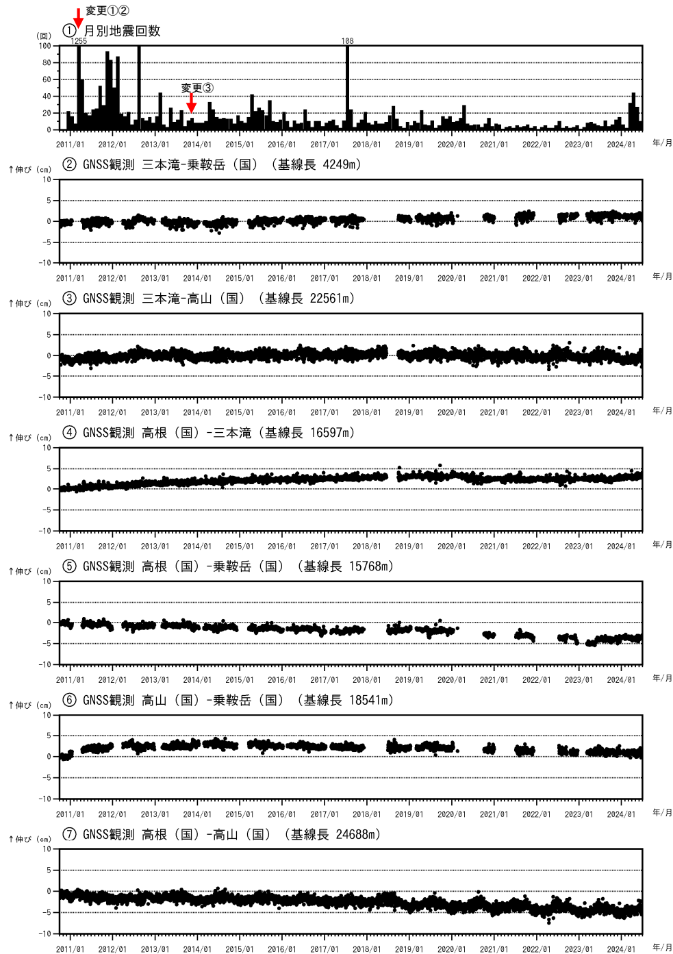
図2 乗鞍岳 火山活動経過図（2010年10月1日～2024年6月30日）
