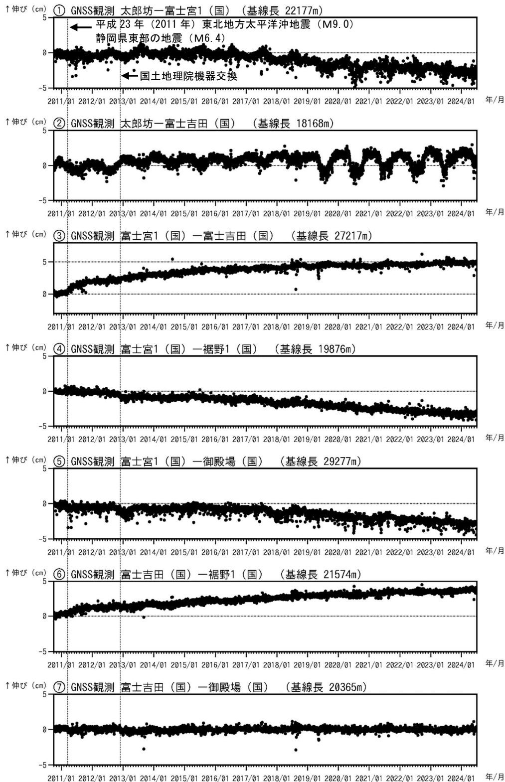
図4 富士山 GNSS 連続観測による基線長変化 (2010 年 10 月 1 日～2024 年 6 月 30 日) (国): 国土地理院 「平成 23 年 (2011 年) 東北地方太平洋沖地震」及び 2011 年 3 月 15 日に発生した静岡県東部の地震 (M 6.4) によるステップ状の変化を補正しています。 ①～⑦は図5の GNSS 基線①～⑦に対応しています。
