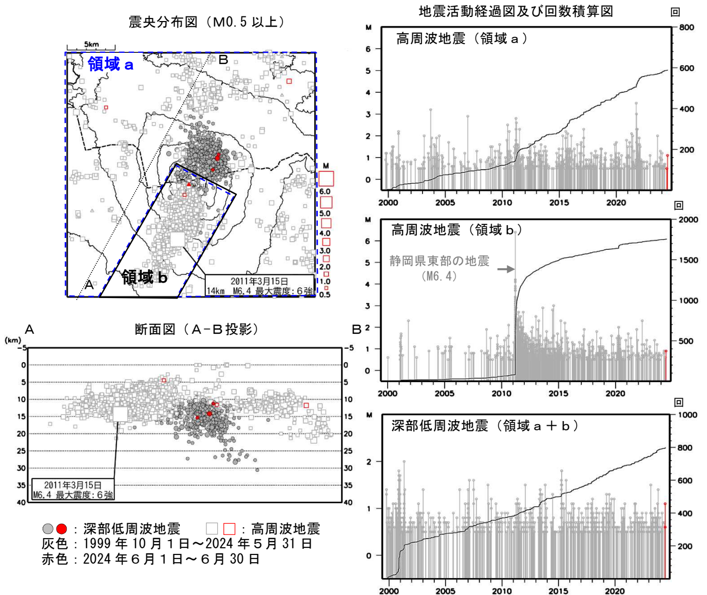
図3 富士山 広域地震観測網による山体及び周辺の地震活動（1999年10月1日～2024年6月30日）
