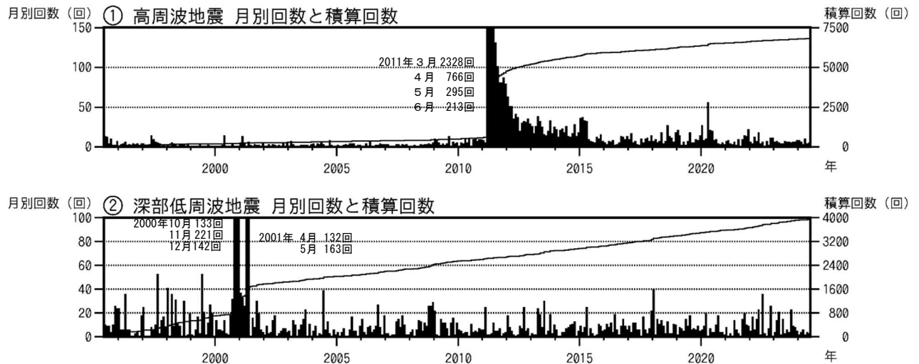
図2 富士山 月別地震回数（1995年6月1日～2024年6月30日）
