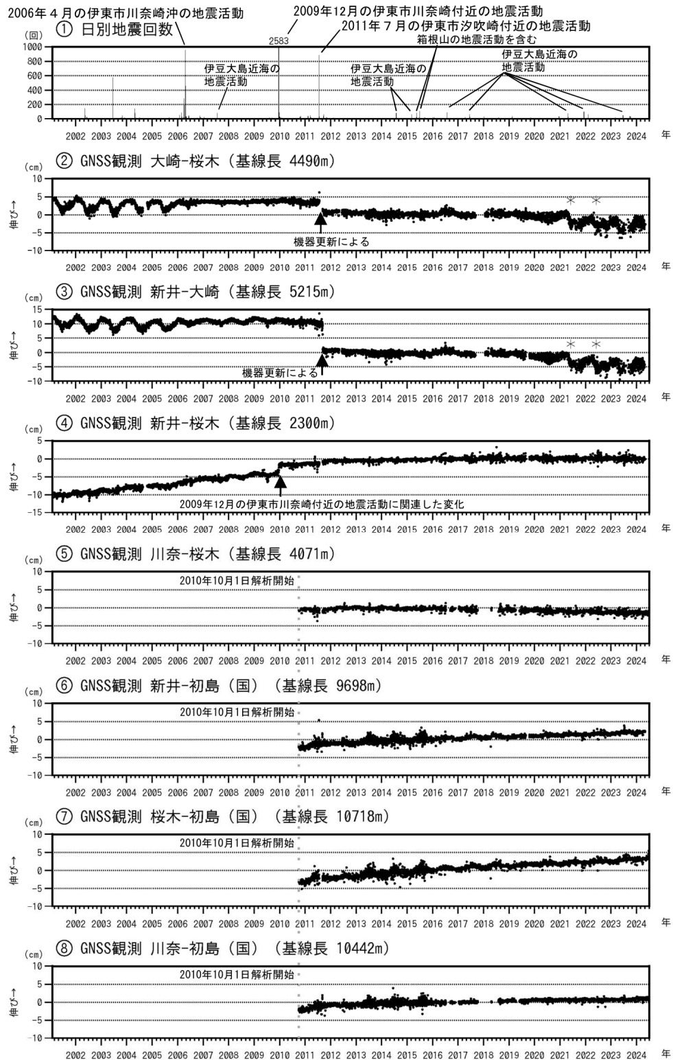
図3 伊豆東部火山群 火山活動経過図（2001年2月1日～2024年6月30日）
