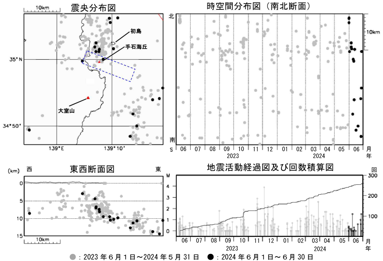
図2 伊豆東部火山群 広域地震観測網による震源分布図（2023 年 6 月 1 日～2024 年 6 月 30 日） □ の領域は群発地震活動の発生する可能性がある範囲（火口が出現する可能性のある範囲）を示しています。 https://www.data.jma.go.jp/vois/data/tokyo/STOCK/level/PDF/level_316.pdf 広域地震観測網により震源決定したもので、深さは全て海面以下として決定しています。 M（マグニチュード）は地震の規模を表し、M0.0 以上を表示しています。 図中の震源要素は一部暫定値が含まれており、後日変更することがあります。 この図では、関係機関の地震波形を一元的に処理し、地震観測点の標高を考慮する等した手法で得られた震源を用いています。
