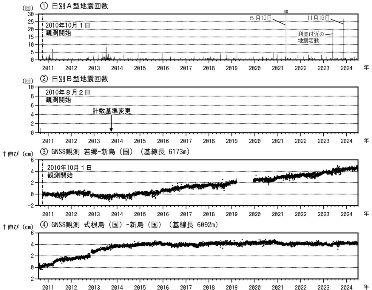
図2 新島 火山活動経過図(2010年8月2日～2024年6月30日)
