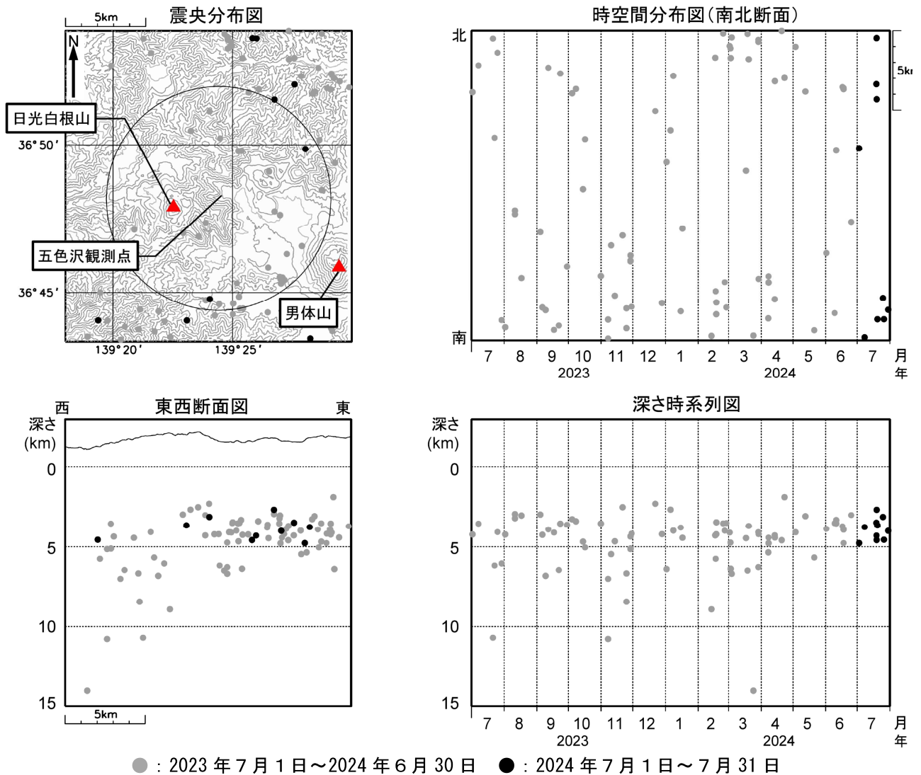
図3 日光白根山 広域地震観測網による山体周辺の地震活動(2023年7月1日～2024年7月31日)
