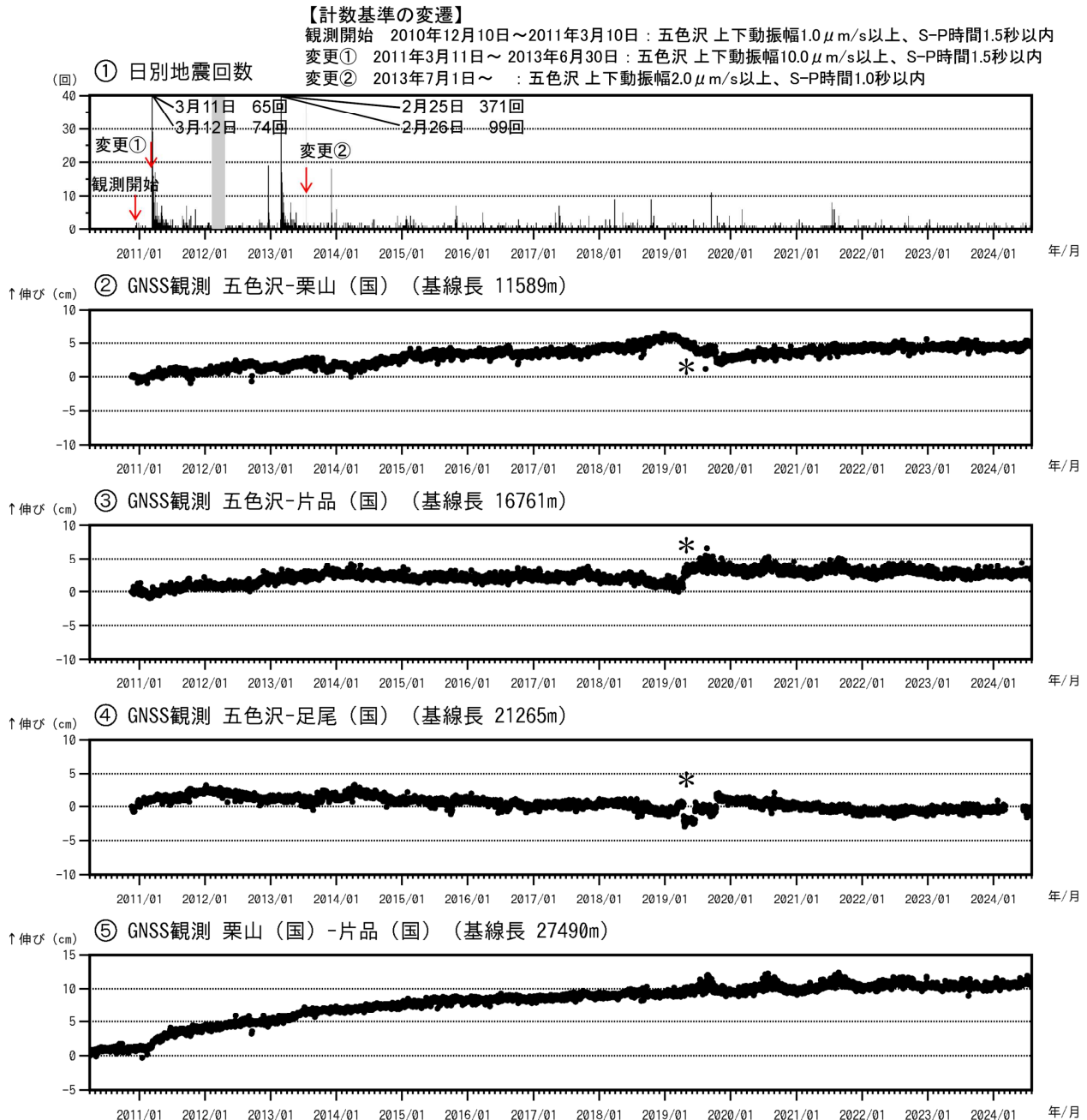
図2 日光白根山 火山活動経過図（2010年4月1日～2024年7月31日）
