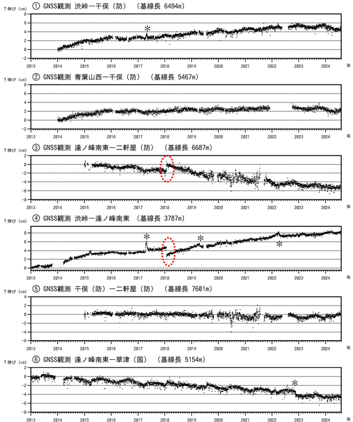
図6-2 草津白根山 GNSS 連続観測の結果（2013年1月1日～2024年7月31日）
