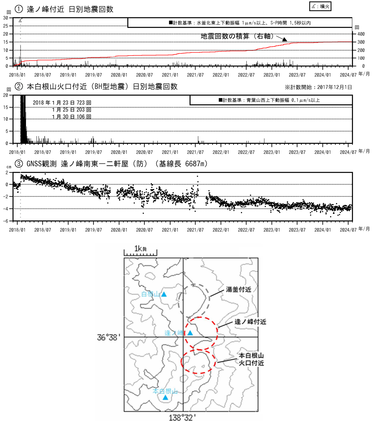
図13 草津白根山（本白根山） 火山活動経過図（2017年12月1日～2024年7月31日）
