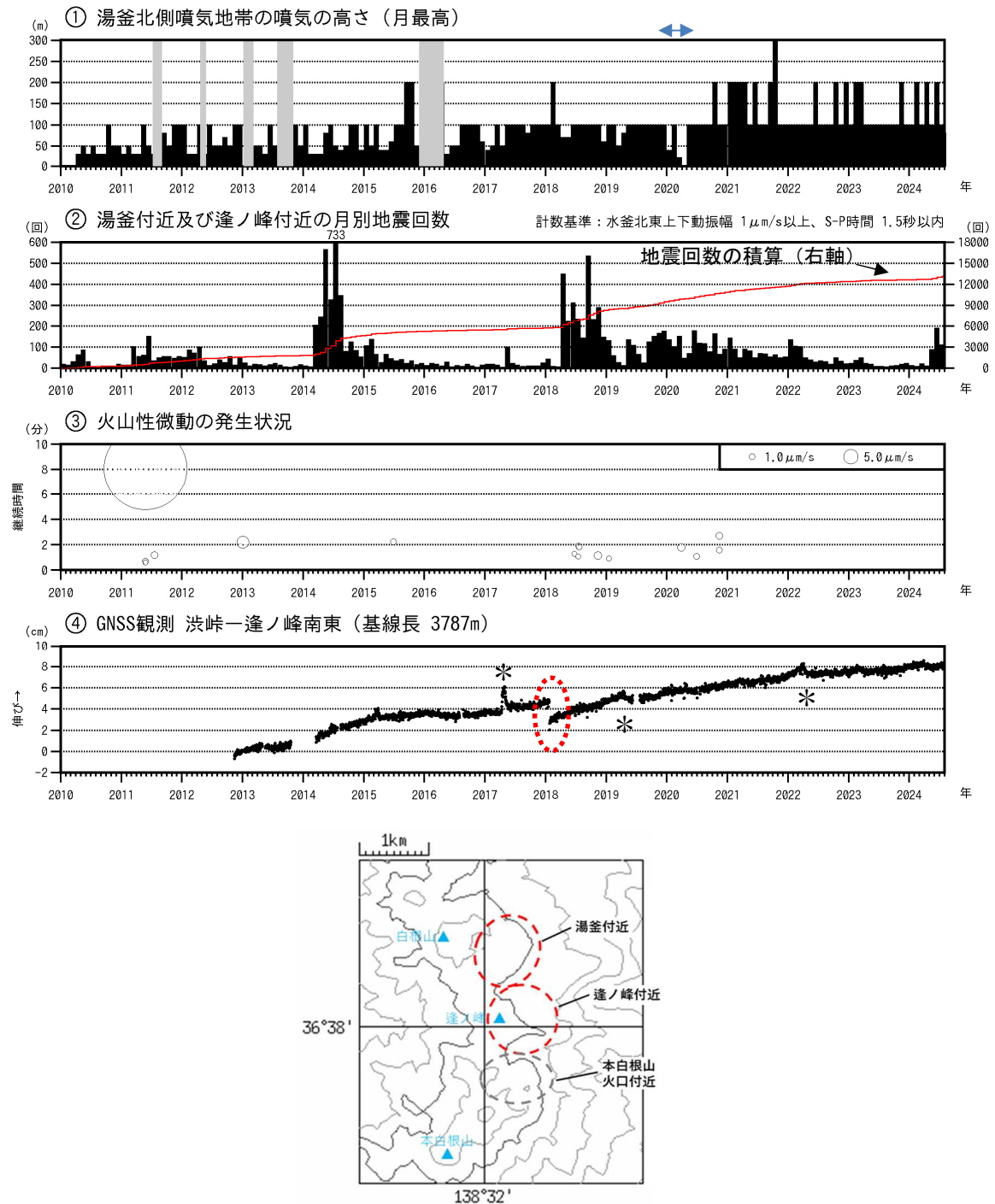
図3 草津白根山（白根山（湯釜付近）） 火山活動経過図（2010年1月1日～2024年7月31日）
