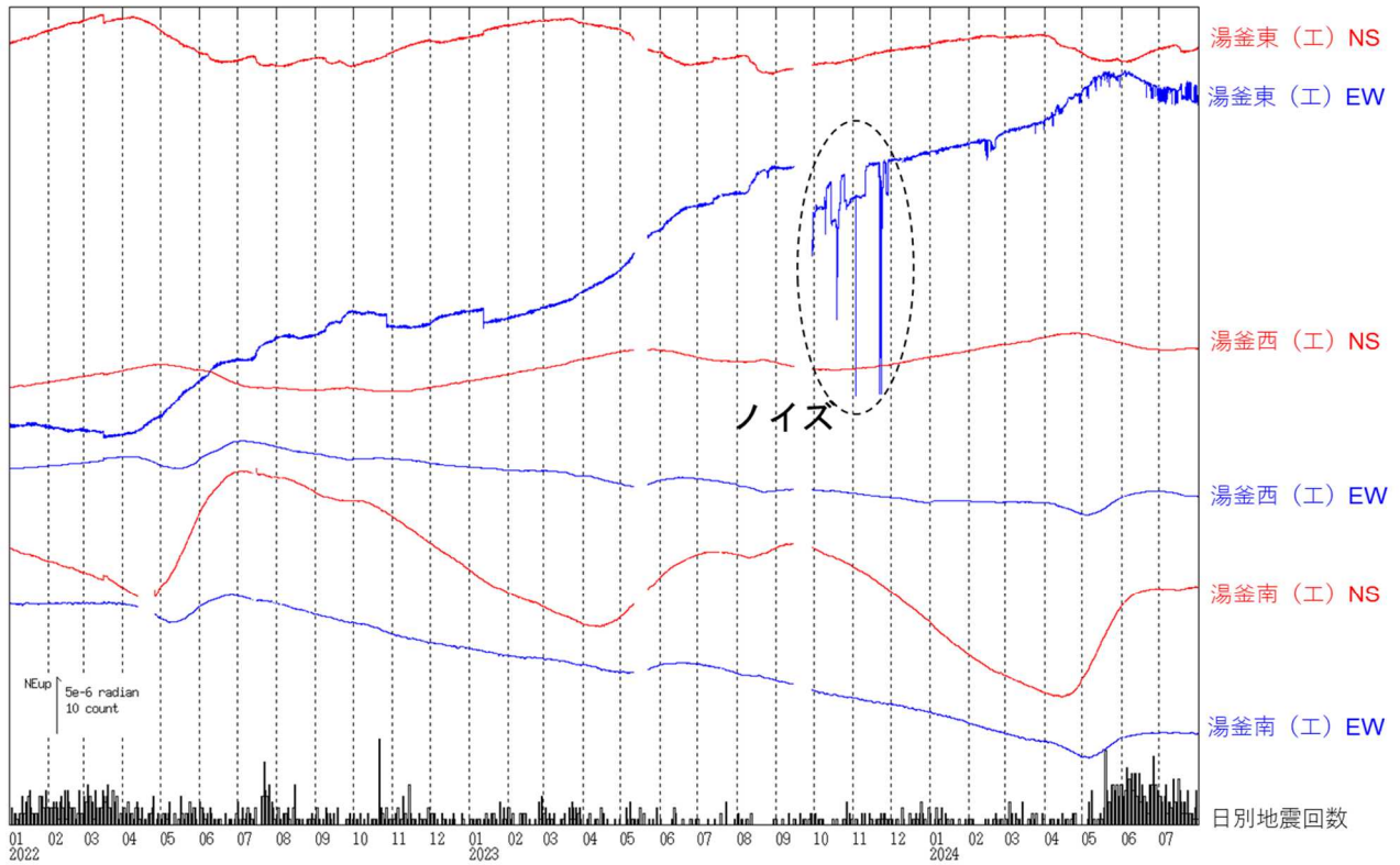
図5 草津白根山（白根山（湯釜付近）） 傾斜変動（2022年1月1日～2024年7月31日） （工）：東京工業大学
