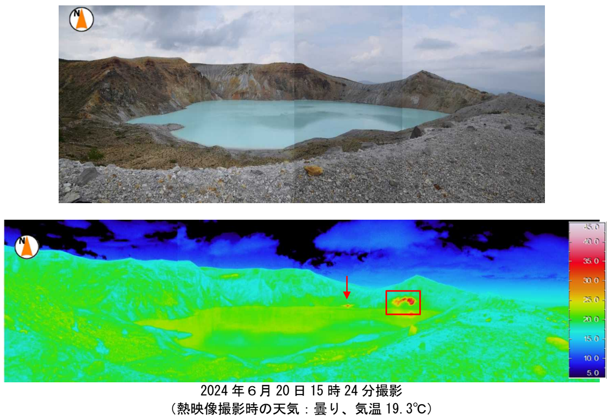
図 2－2 草津白根山（白根山（湯釜付近））湯釜火口内の状況
