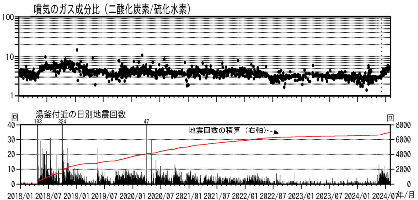
図8 草津白根山（白根山（湯釜付近）） 火山ガス観測結果（2018年1月～2024年7月）
