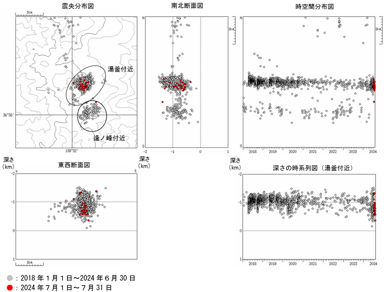
図4 草津白根山 震源分布図（2018 年 1 月 1 日～2024 年 7 月 31 日）
