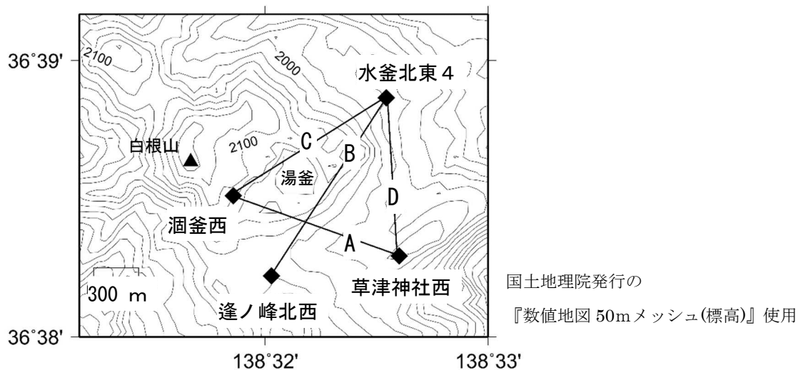
図6－1 草津白根山 湯釜近傍での臨時のGNSS連続観測結果(2024年5月29日～2024年7月31日) 下図の◆(水釜北東4、涸釜西、草津神社西及び逢ノ峰北西)は、臨時に設置したGNSS連続観測点を示します。 上図の①～④は下図のA～Dと対応しています。
