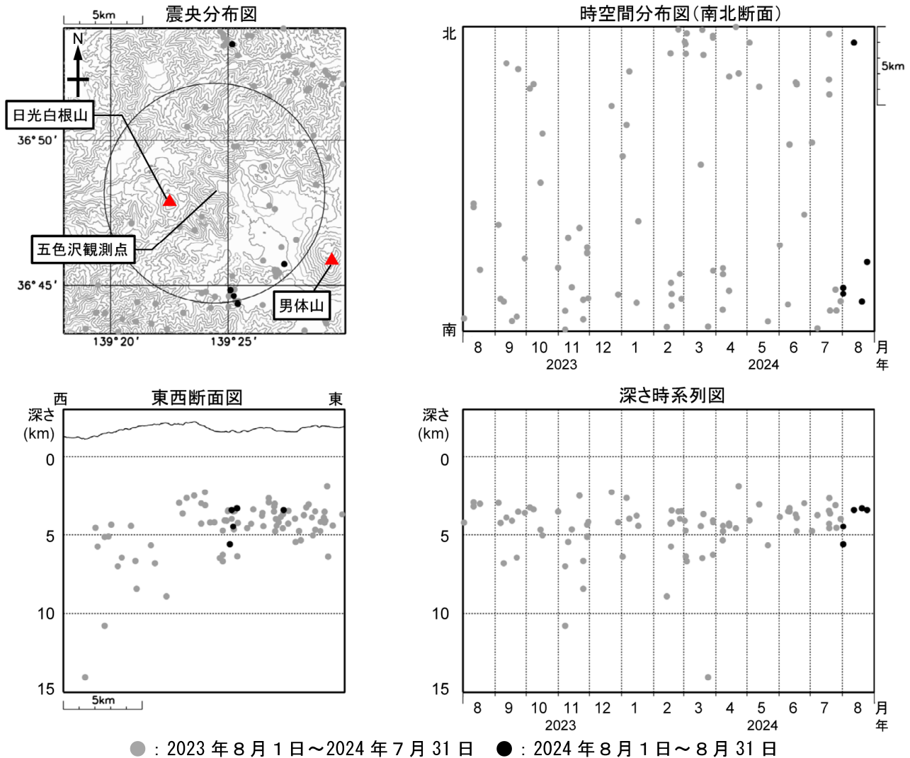
図3 日光白根山 広域地震観測網による山体周辺の地震活動(2023年8月1日～2024年8月31日)
