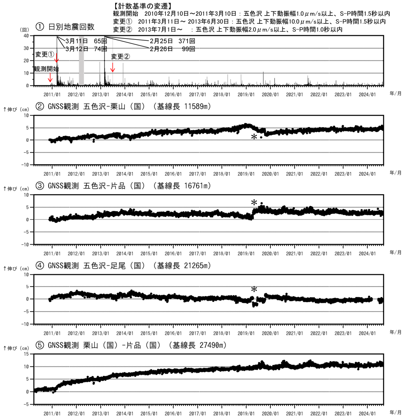
図2 日光白根山 火山活動経過図（2010年4月1日～2024年8月31日）
