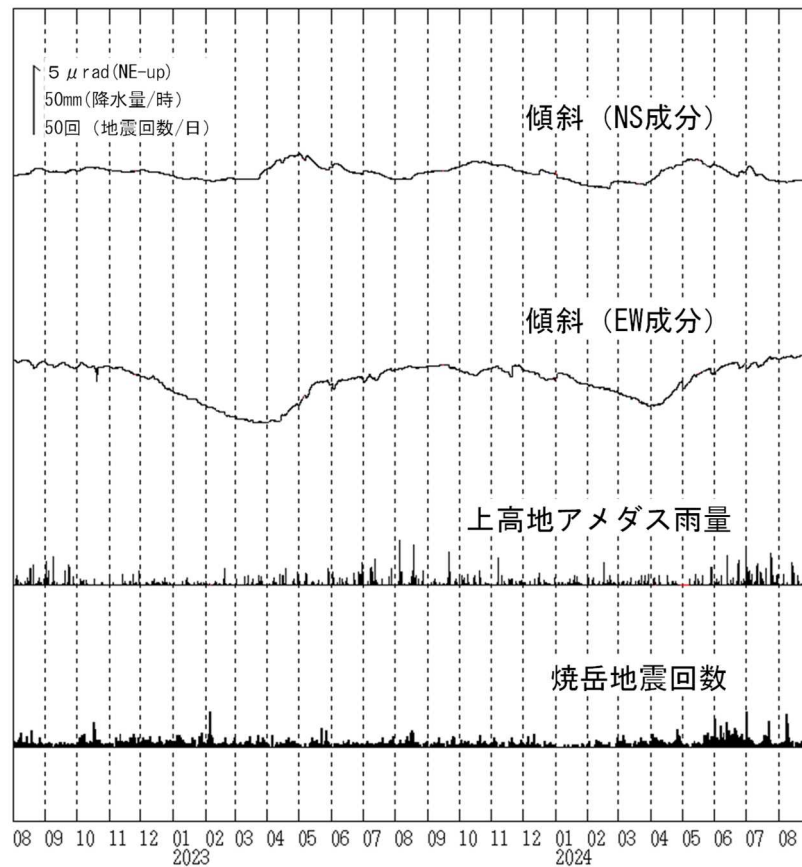
図8 焼岳 南峰南東観測点における傾斜データ（2022年8月1日～2024年8月31日）
