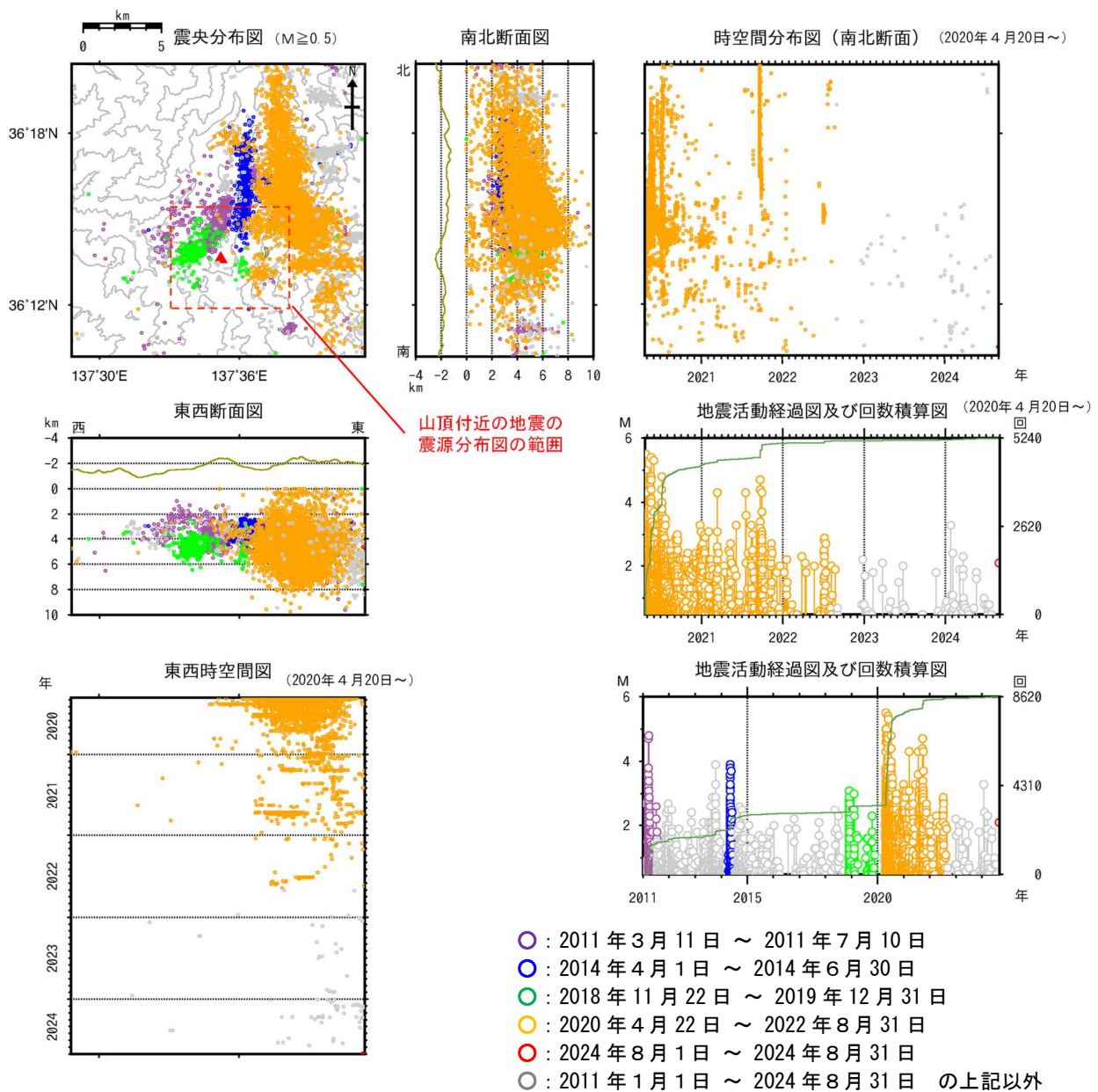
図9 焼岳 広域地震観測網による山体及び周辺の地震活動(2011年1月1日～2024年8月31日)
