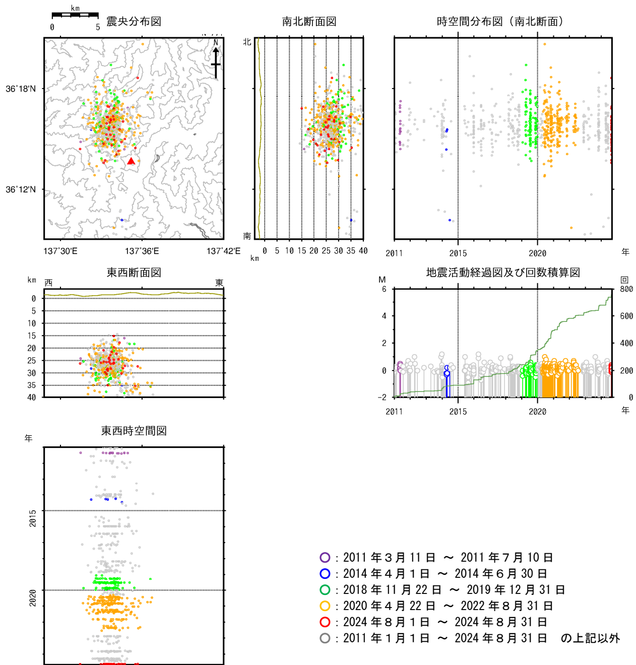
図10 焼岳 広域地震観測網による深部低周波地震の震源分布図（2011年1月1日～2024年8月31日） 広域地震観測網により震源決定したもので、深さは全て海面以下として決定しています。そのため、山頂付近の浅い地震の震源も海面下に決定されています。
