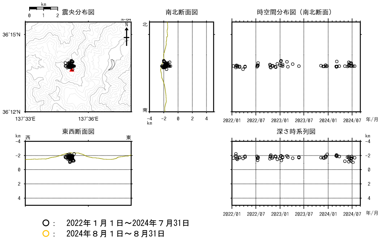
図2 焼岳 山頂付近の地震の震源分布図（2022年1月1日～2024年8月31日）
