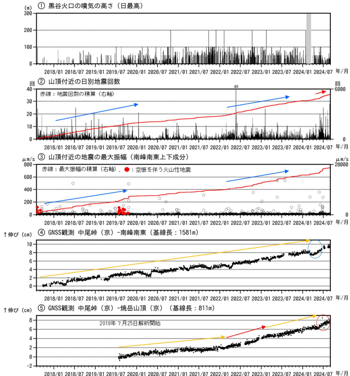
図1-1 焼岳 火山活動経過図（2017年8月1日～2024年8月31日）
