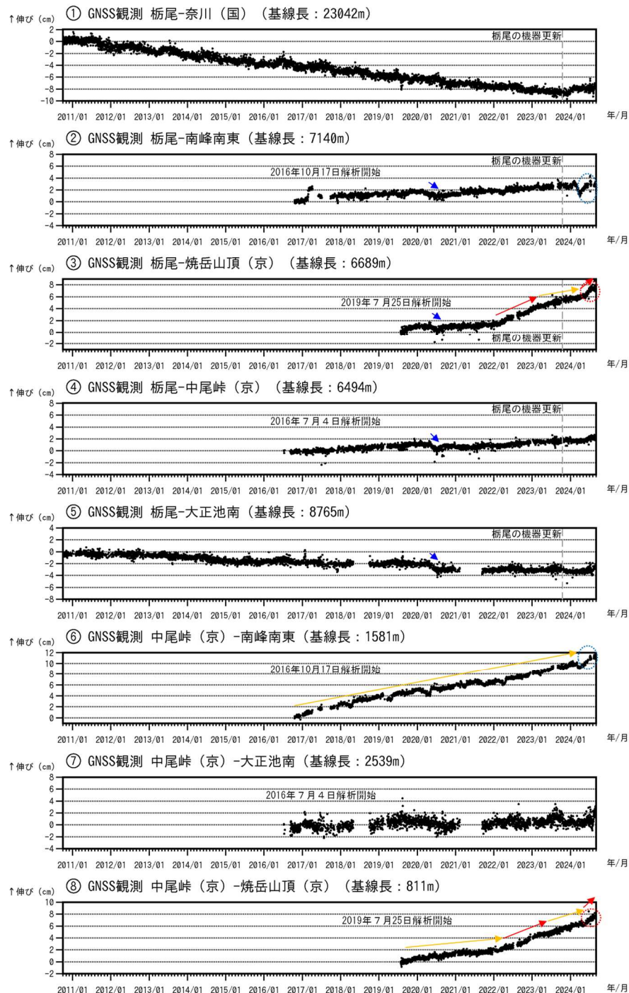
図6 焼岳 GNSS 連続観測による基線長変化（2010年10月1日～2024年8月31日）
