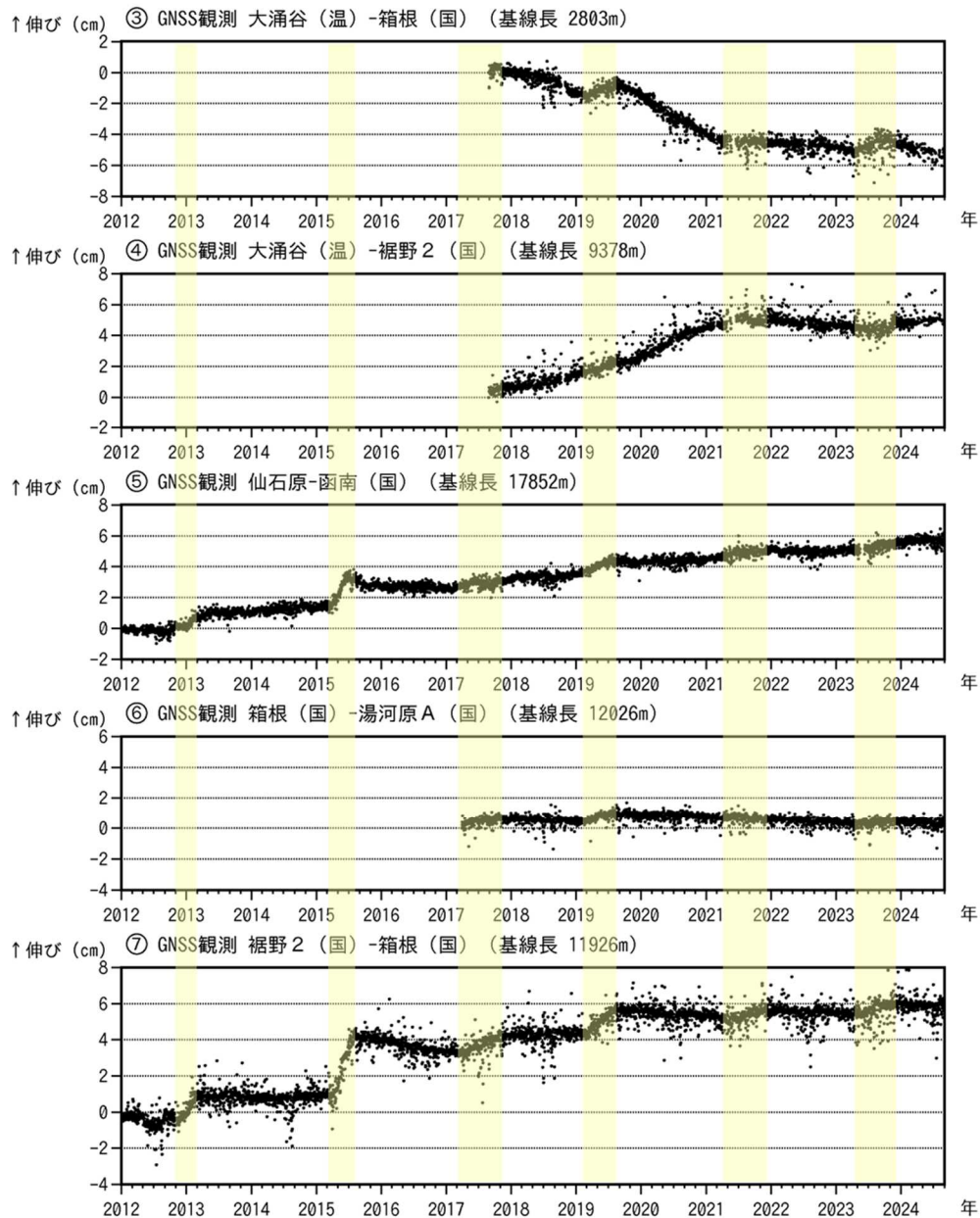
図3-2 箱根山 GNSS連続観測による 基線長変化及び観測点配置図 (2012年1月1日～2024年8月31日) (国): 国土地理院 (温): 神奈川県温泉地学研究所 空白部分は欠測を示します。
