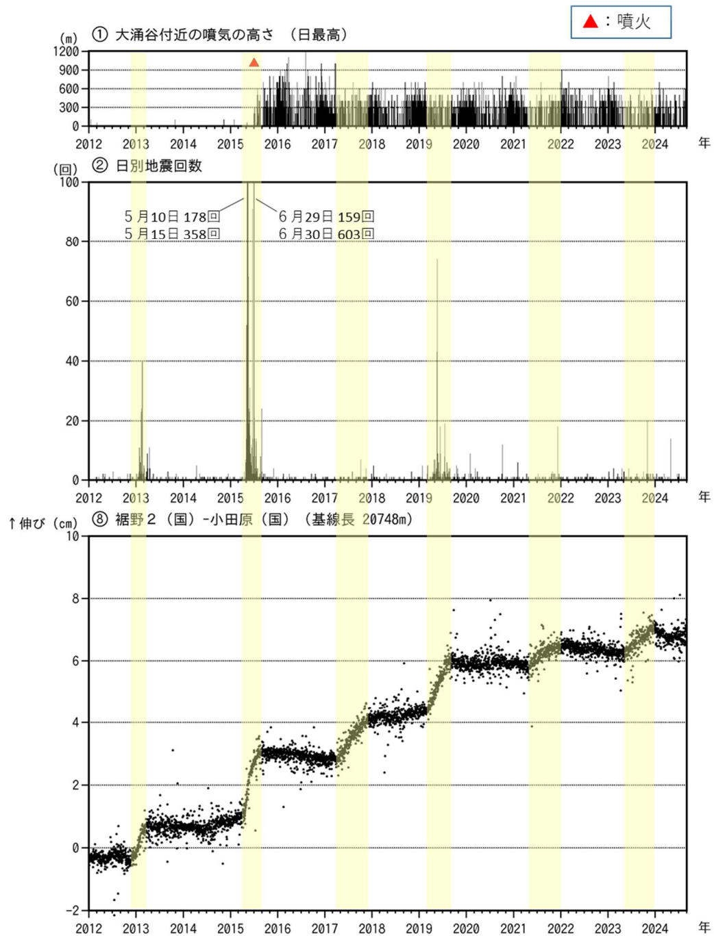
図3-1 箱根山 火山活動経過図（2012年1月1日～2024年8月31日）
