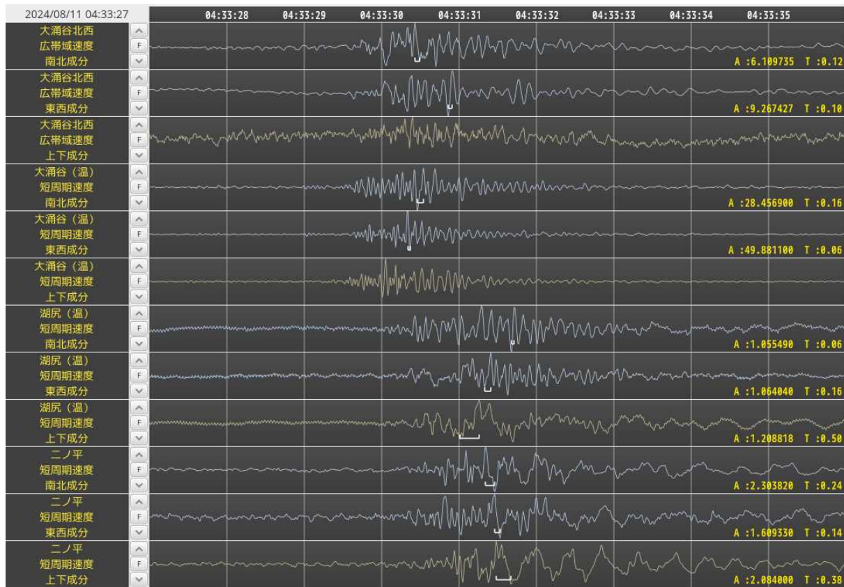
図5 箱根山 8月11日4時33分に大涌谷付近で発生した地震の波形図(大涌谷北西、大涌谷(温)、湖尻(温)、二ノ平)
