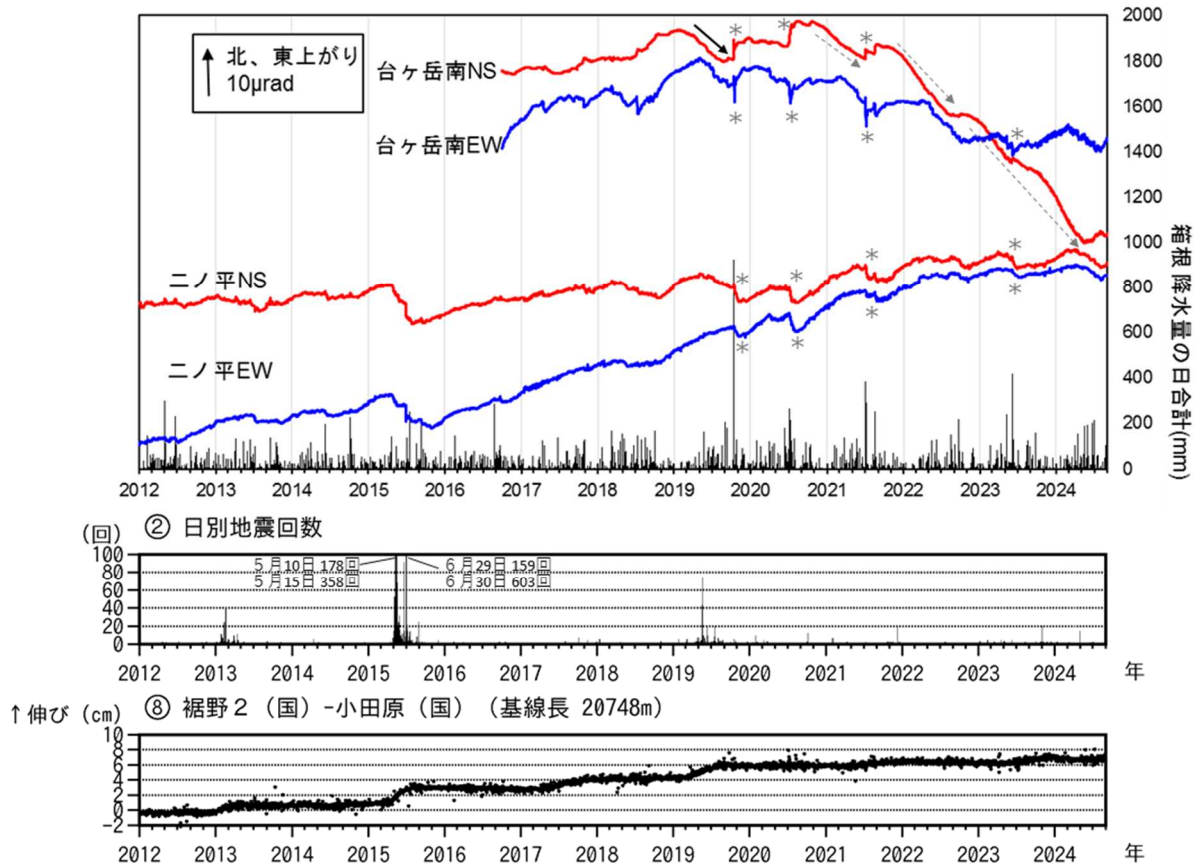
図6 箱根山 傾斜観測及び地震回数・GNSS観測（2012年1月1日～2024年8月31日）
