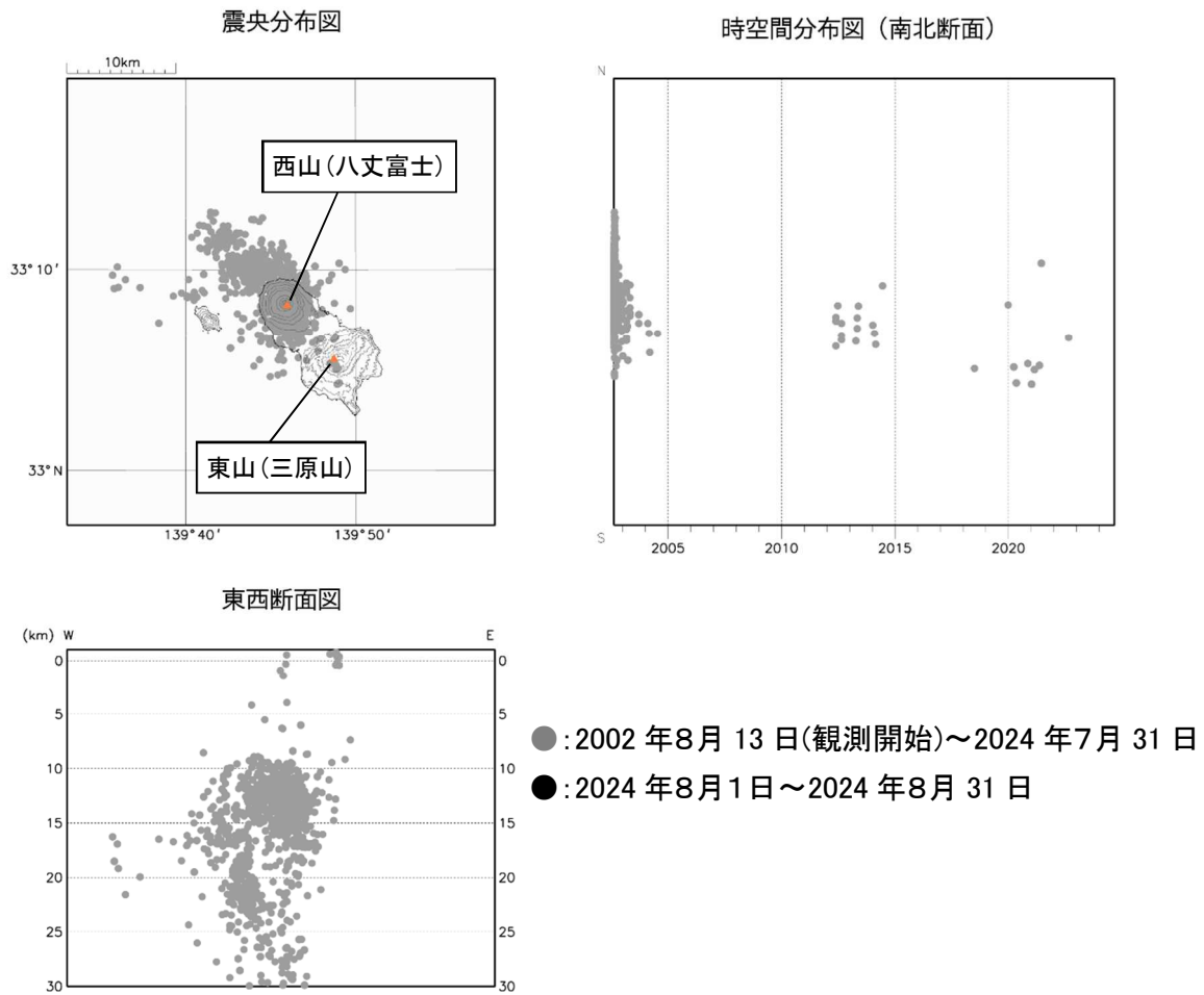
図3 八丈島 震源分布図（2002年8月13日～2024年8月31日）
