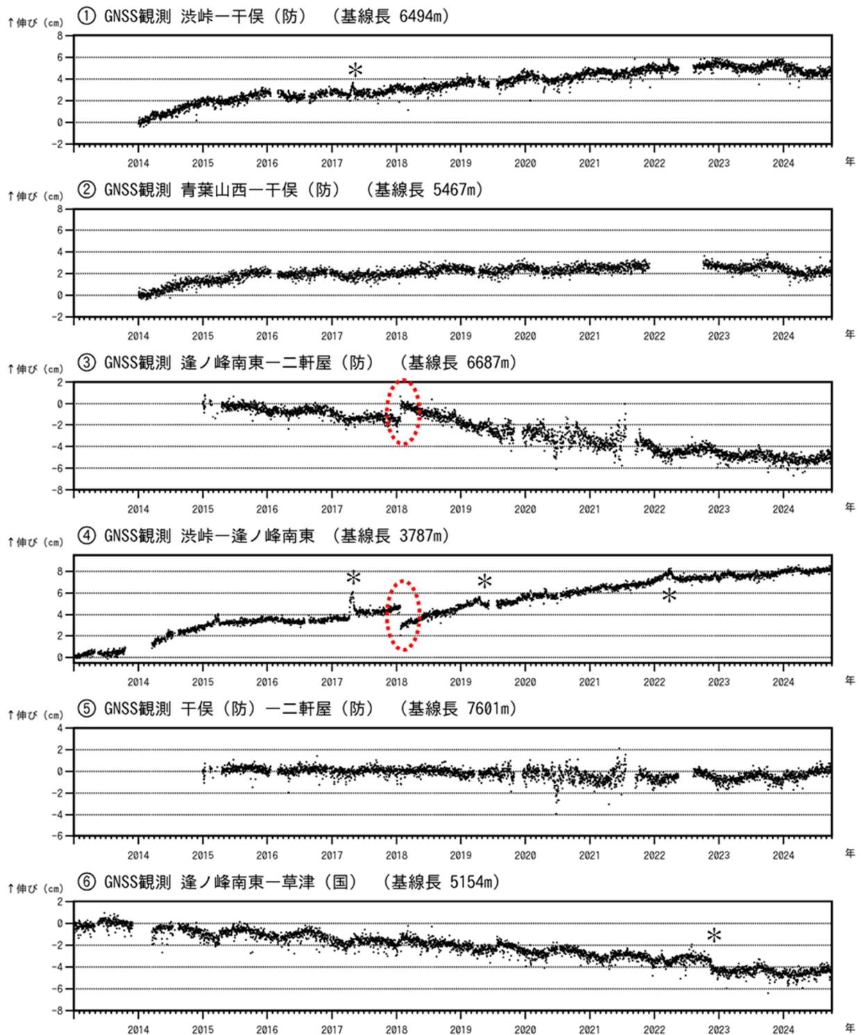
図6-2 草津白根山 GNSS 連続観測の結果（2013年1月1日～2024年8月31日）
