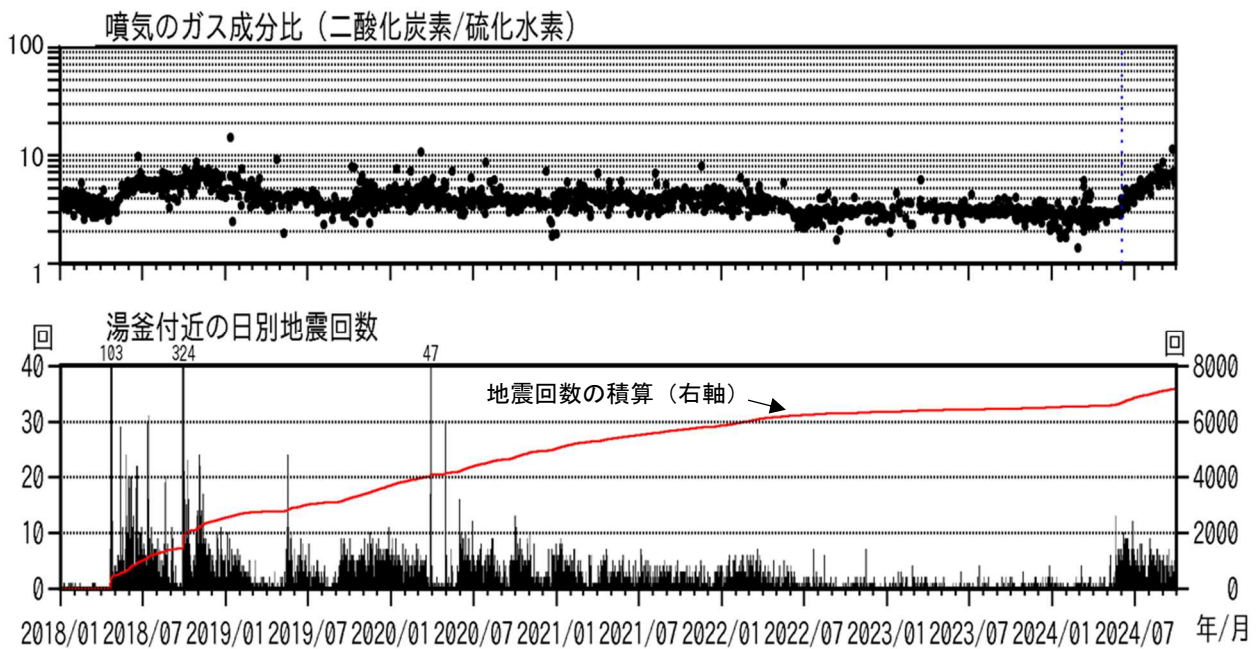
図8 草津白根山（白根山（湯釜付近）） 火山ガス観測結果（2018年1月～2024年9月）
