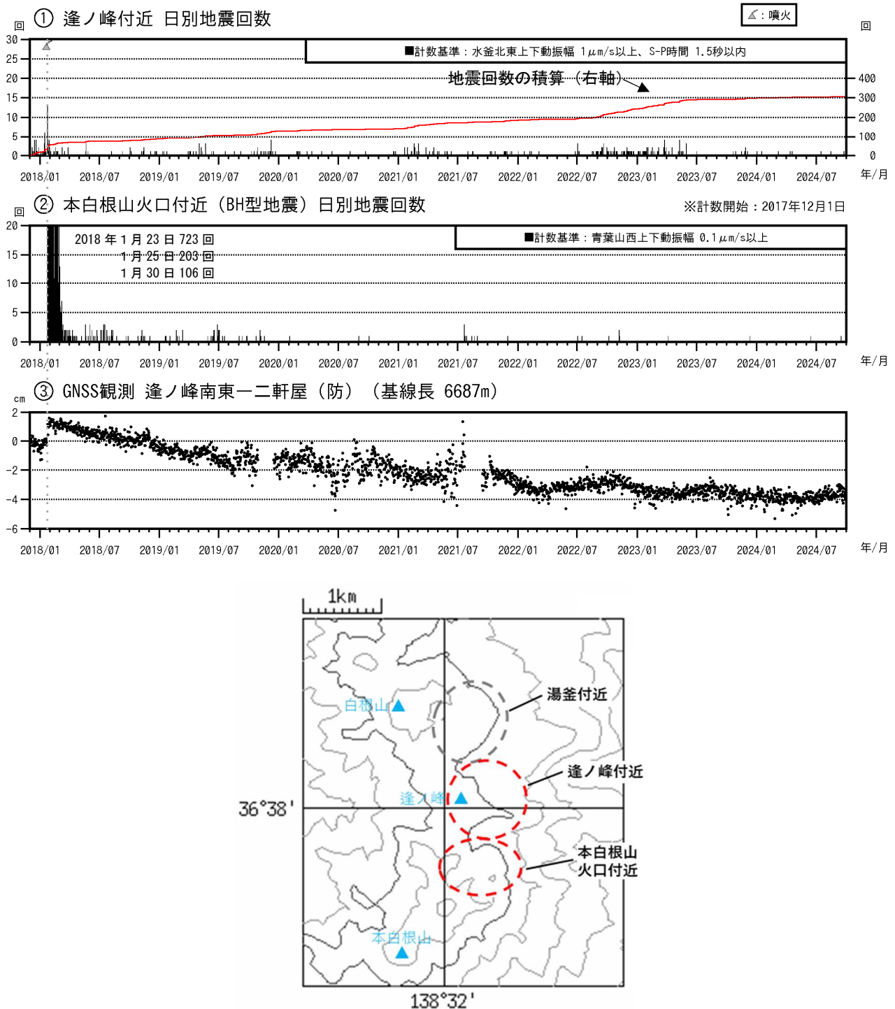
図13 草津白根山（本白根山） 火山活動経過図（2017年12月1日～2024年9月30日）
