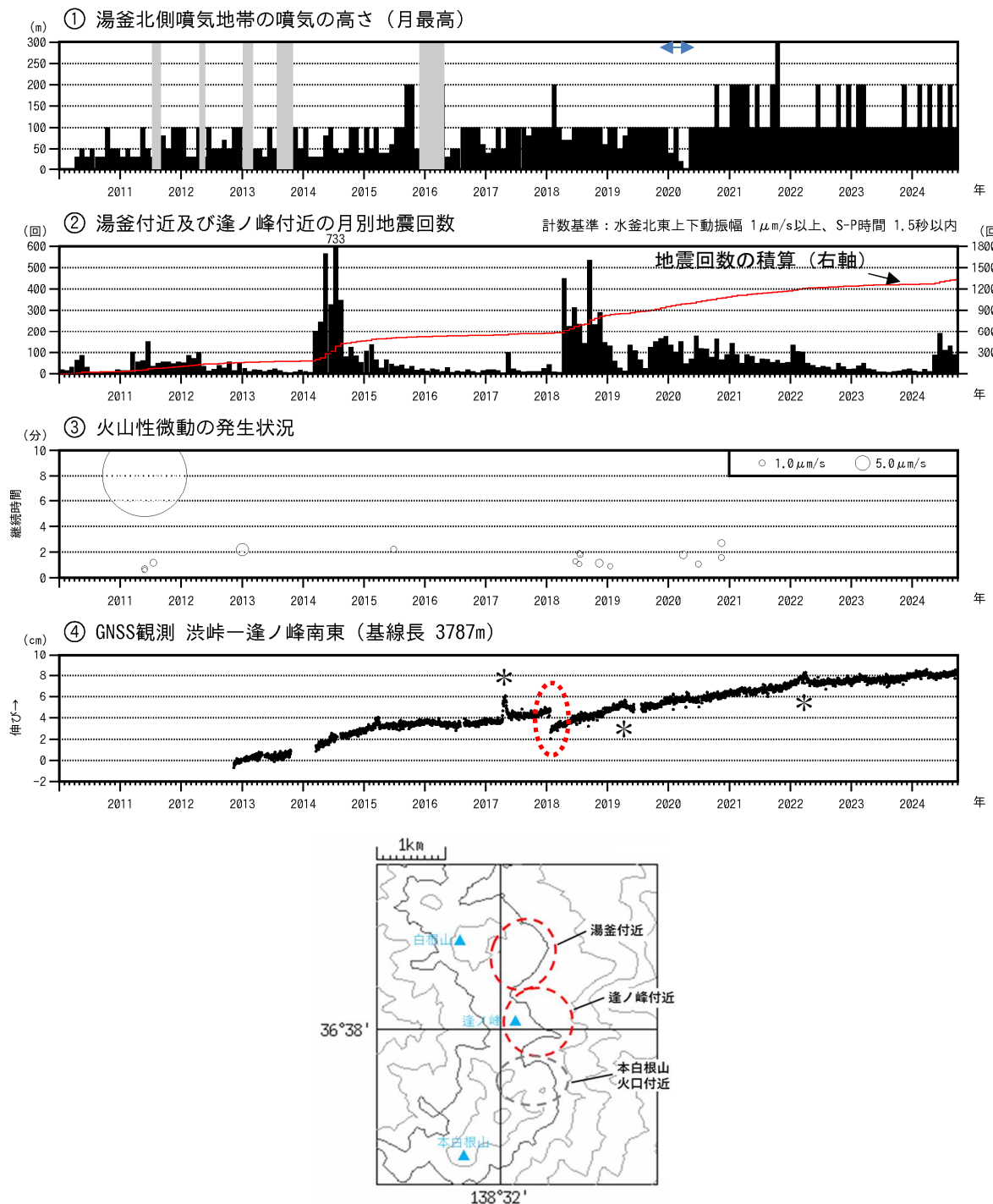
図3 草津白根山（白根山（湯釜付近）） 火山活動経過図（2010年1月1日～2024年9月30日）
