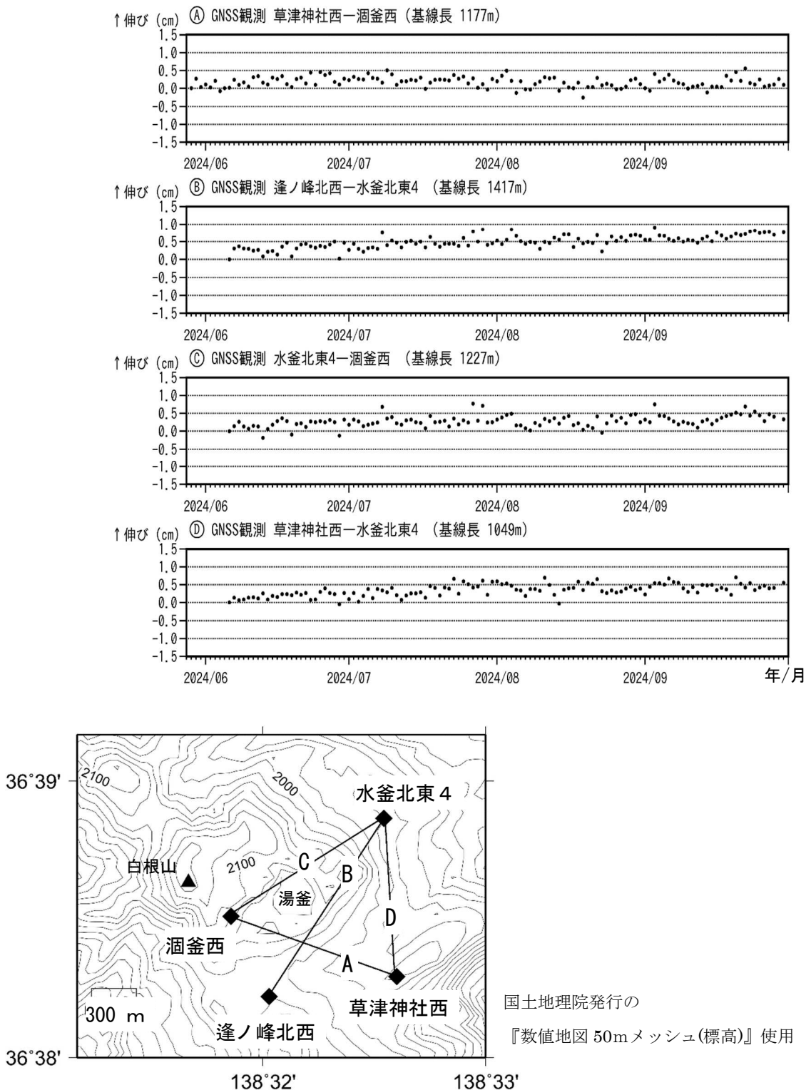
図6－1 草津白根山 湯釜近傍での臨時のGNSS連続観測結果(2024年5月29日～2024年9月30日) 下図の◆(水釜北東4、涸釜西、草津神社西及び逢ノ峰北西)は、臨時に設置したGNSS連続観測点を示します。 上図の①～④は下図のA～Dと対応しています。
