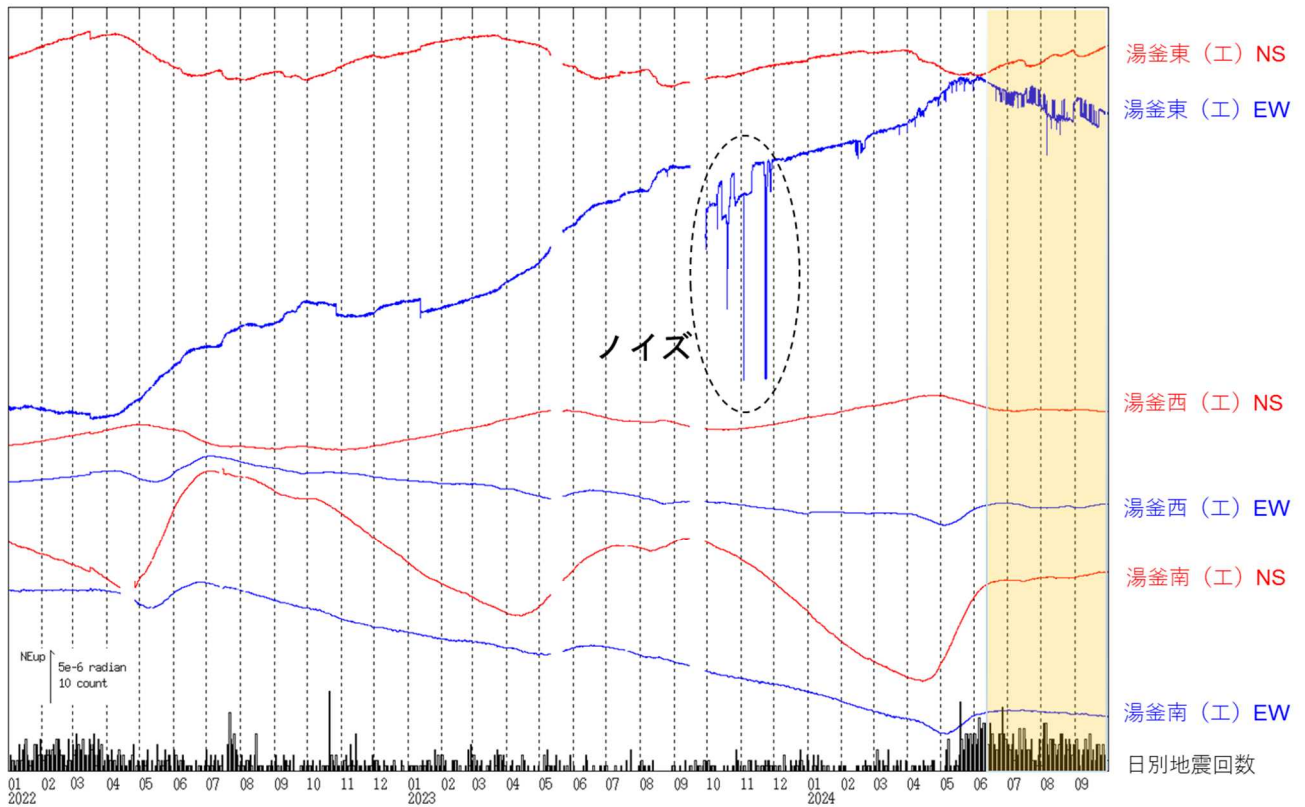
図5 草津白根山（白根山（湯釜付近）） 傾斜変動（2022年1月1日～2024年9月30日）
