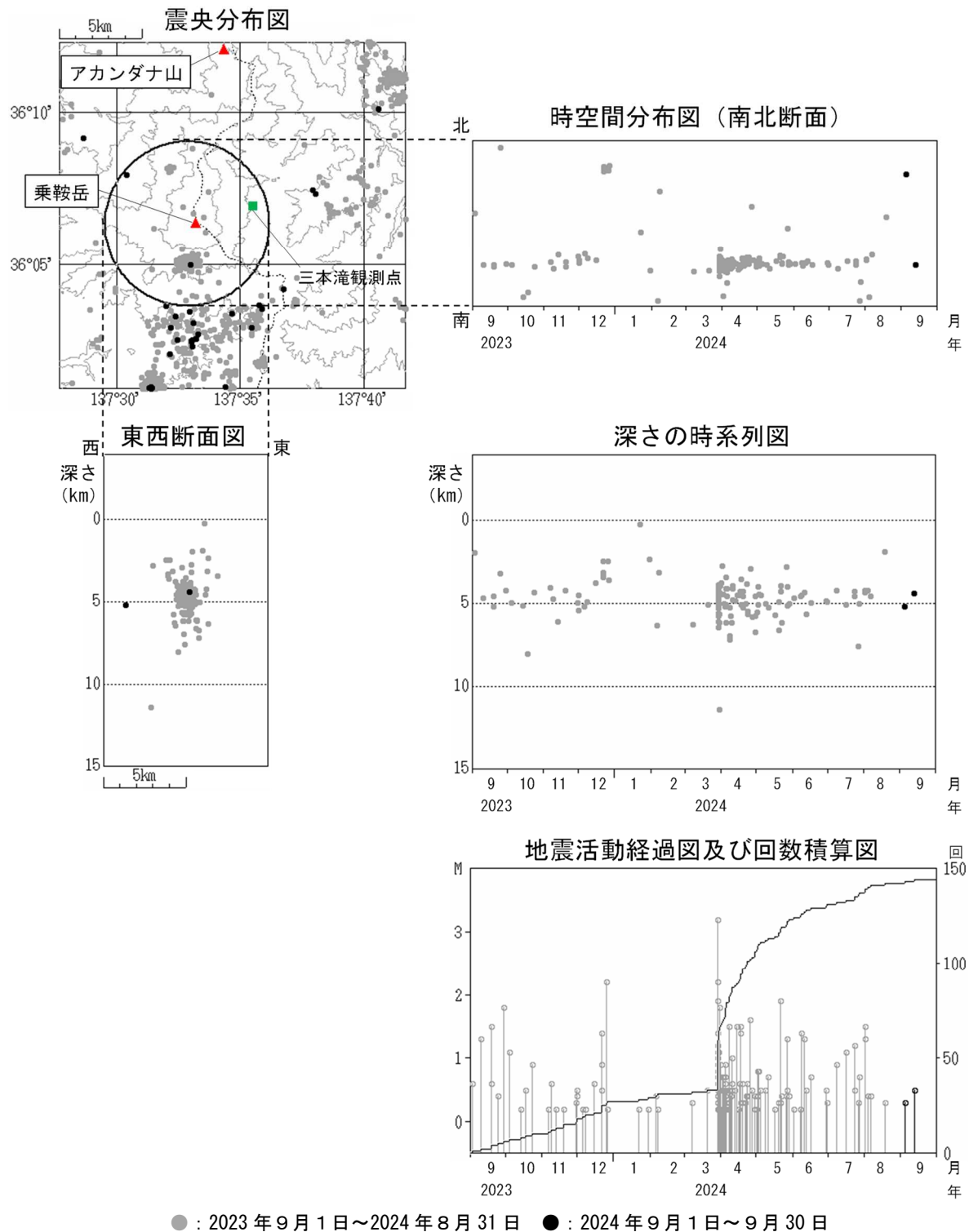
図3 乗鞍岳 広域地震観測網による山体・周辺の地震活動(2023年9月1日～2024年9月30日)
