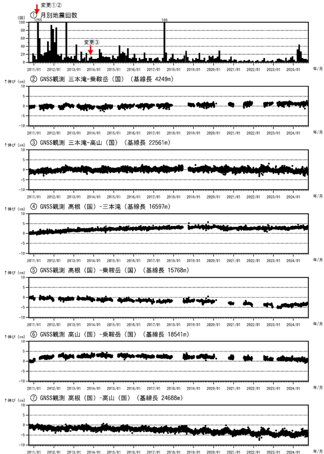
図2 乗鞍岳 火山活動経過図（2010年10月1日～2024年9月30日）
