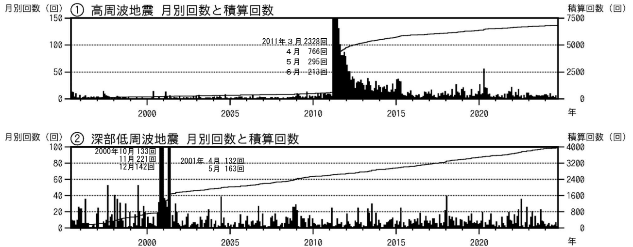
図2 富士山 月別地震回数（1995年6月1日～2024年9月30日）
