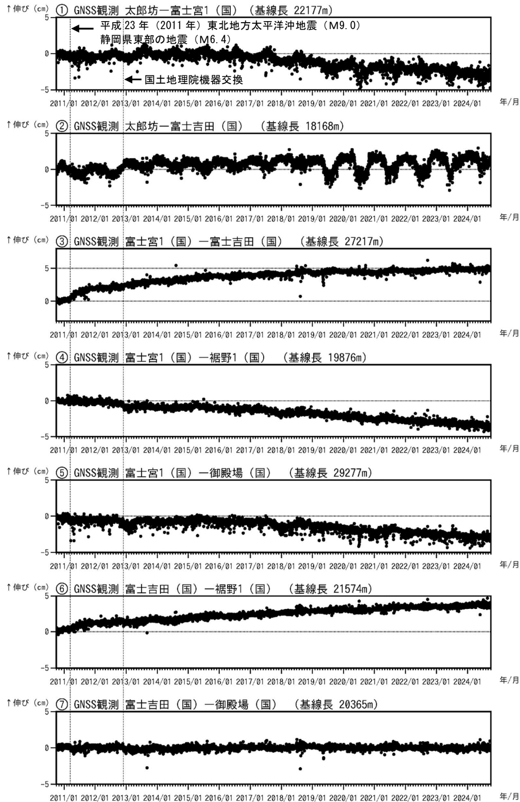
図4 富士山 GNSS 連続観測による基線長変化 (2010年10月1日～2024年9月30日) (国): 国土地理院 「平成23年 (2011年) 東北地方太平洋沖地震」及び2011年3月15日に発生した静岡県東部の地震 (M6.4) によるステップ状の変化を補正しています。 ①～⑦は図5のGNSS基線①～⑦に対応しています。
