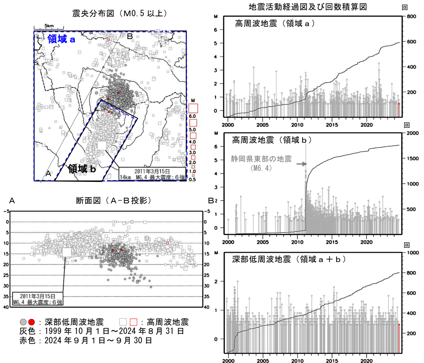
図3 富士山 広域地震観測網による山体及び周辺の地震活動（1999年10月1日～2024年9月30日）
