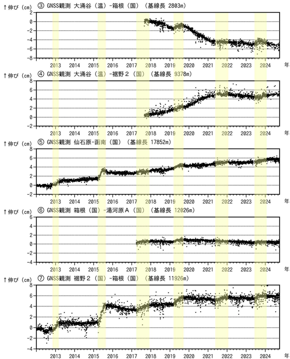
図3-2 箱根山 GNSS 連続観測による 基線長変化及び観測点配置図 (2012年1月1日～2024年9月30日) (国): 国土地理院 (温): 神奈川県温泉地学研究所 空白部分は欠測を示します。
