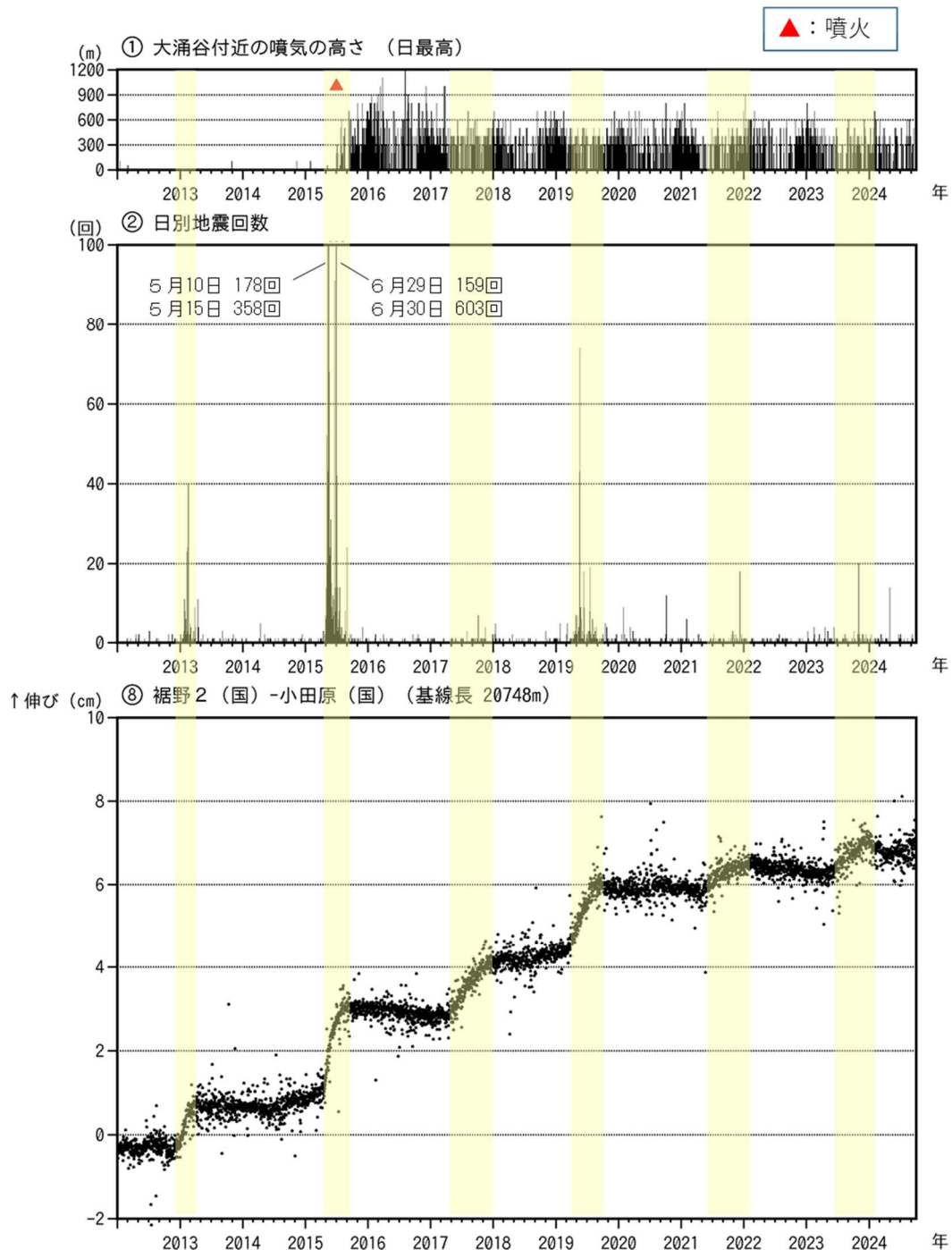
図3-1 箱根山 火山活動経過図（2012年1月1日～2024年9月30日）
