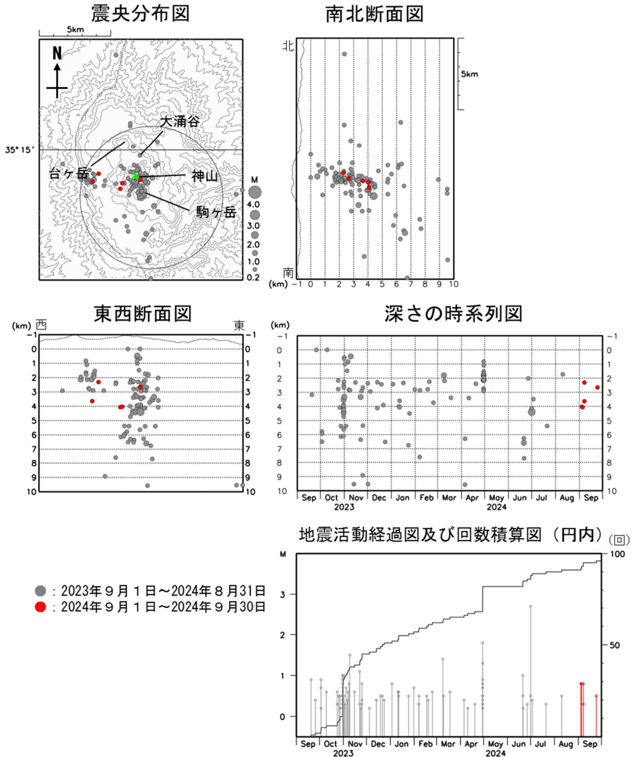
図4 箱根山 広域地震観測網による山体周辺の震源分布図（2023年9月1日～2024年9月30日）
