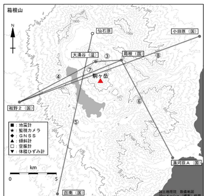
図3-2 箱根山 GNSS 連続観測による 基線長変化及び観測点配置図 (2012年1月1日～2024年9月30日) (国): 国土地理院 (温): 神奈川県温泉地学研究所 空白部分は欠測を示します。
