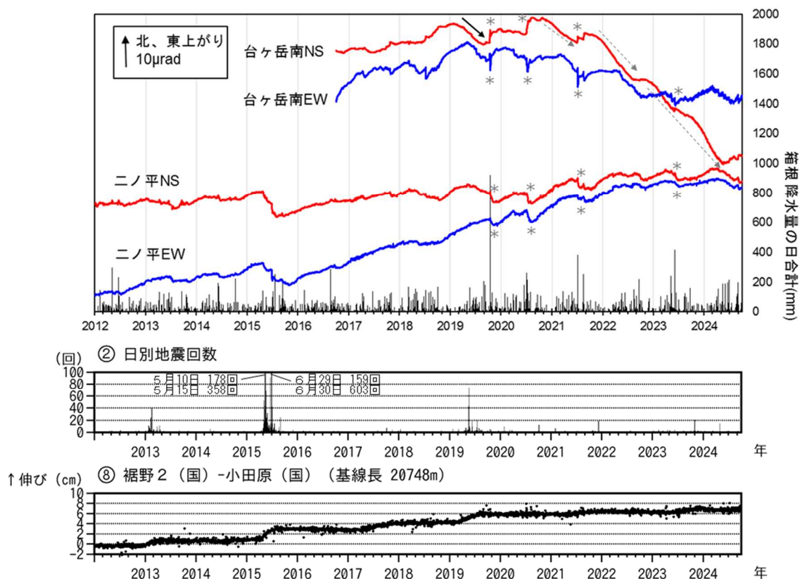
図5 箱根山 傾斜観測及び地震回数・GNSS観測（2012年1月1日～2024年9月30日）
