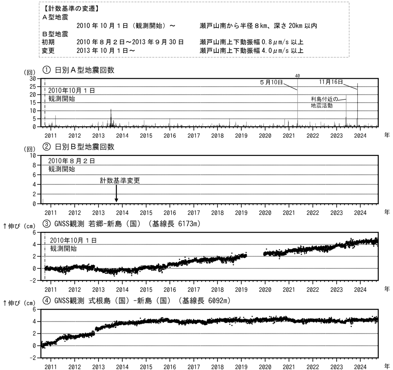
図2 新島 火山活動経過図(2010年8月2日～2024年9月30日)
