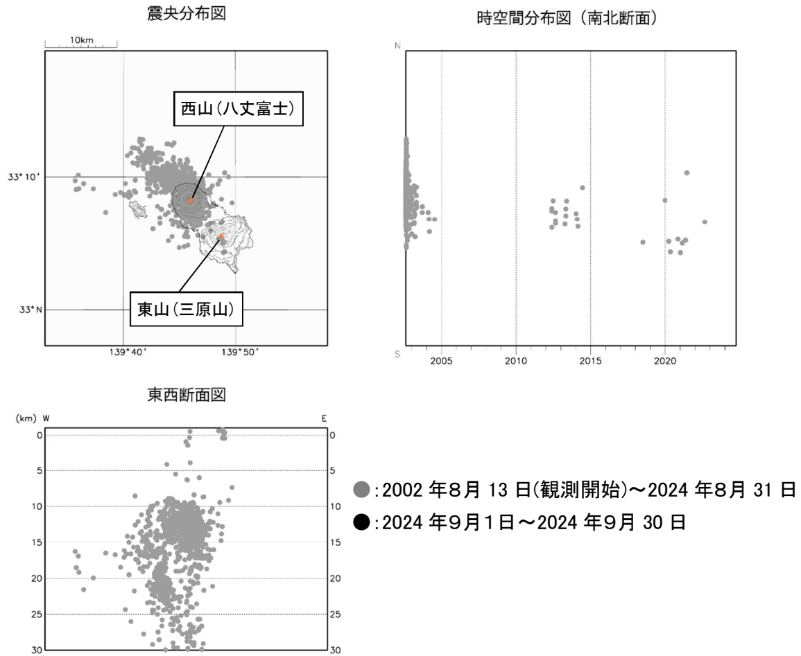
図3 八丈島 震源分布図（2002 年 8 月 13 日～2024 年 9 月 30 日）
