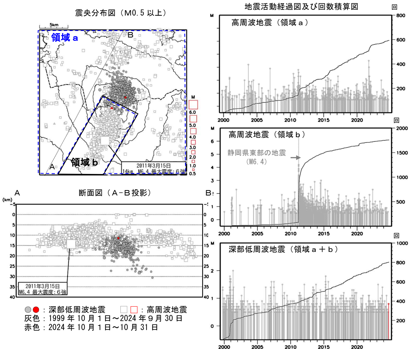
図3 富士山 広域地震観測網による山体及び周辺の地震活動（1999年10月1日～2024年10月31日）
