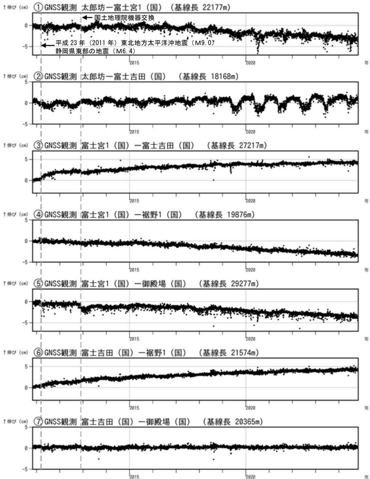
図4 富士山 GNSS連続観測による基線長変化(2010年10月1日～2024年10月31日) (国): 国土地理院 「平成23年(2011年)東北地方太平洋沖地震」及び2011年3月15日に発生した静岡県東部の地震(M6.4)によるステップ状の変化を補正しています。 ①～⑦は図5のGNSS基線①～⑦に対応しています。
