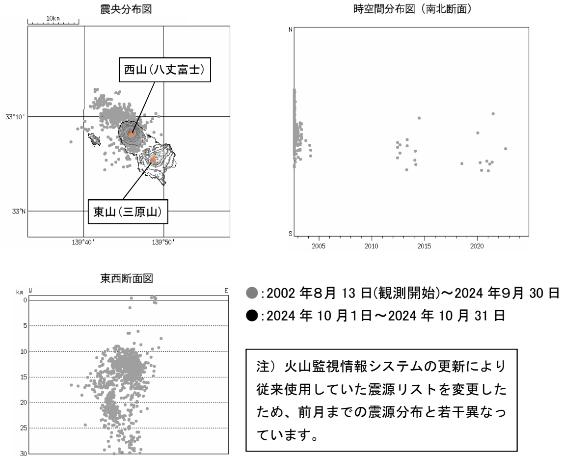
図3 八丈島 震源分布図（2002 年 8 月 13 日～2024 年 10 月 31 日）
