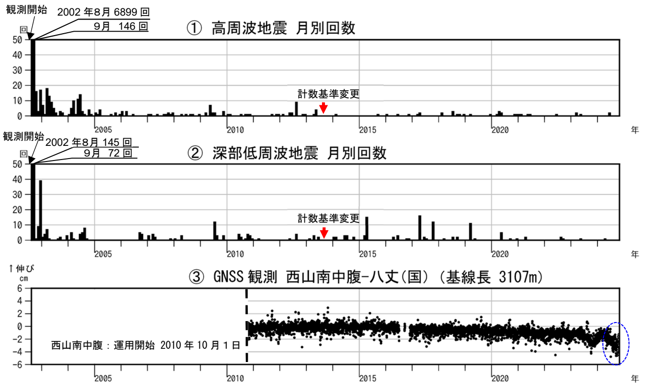
図2 八丈島 火山活動経過図（2002年8月13日～2024年10月31日）
